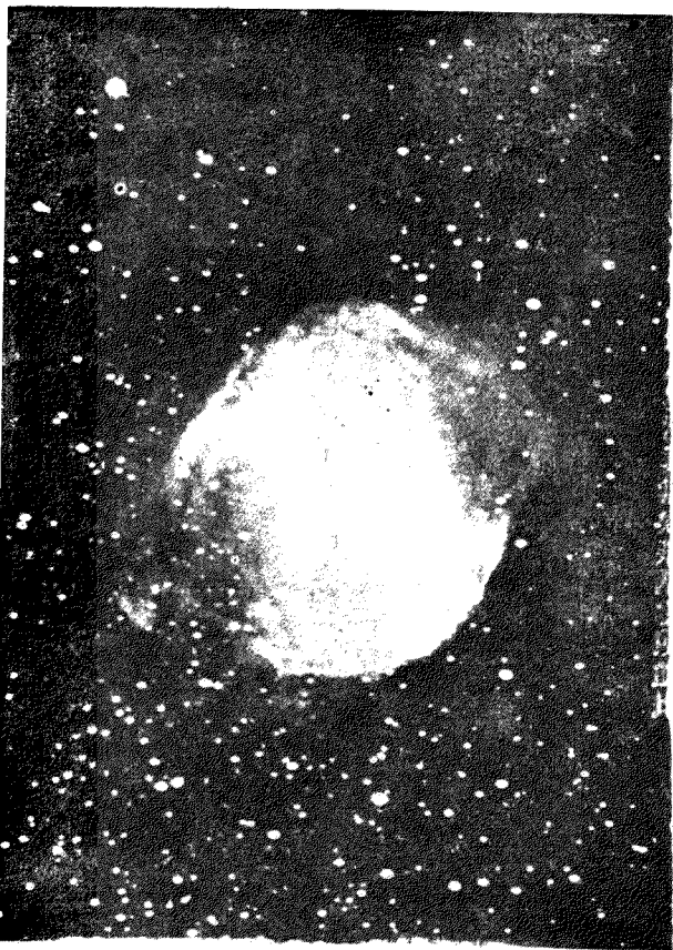
最大形之行星狀星雲，研究上甚重要之星雲。
