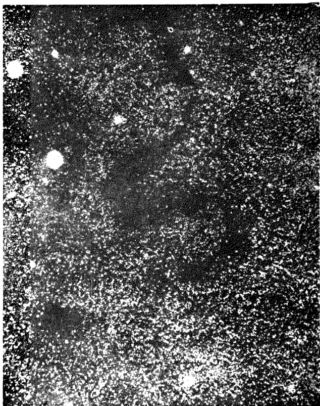
第二百二十四圖 蛇夫座S形暗星雲
