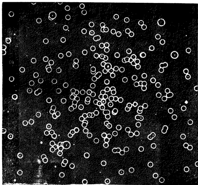
第二百四十一圖 后髮座一隅多數星雲之密集
