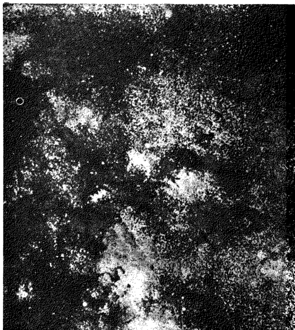
明示暗星雲之複雜。
