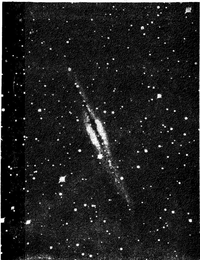
第二百四十七圖 仙女座之梭狀星雲，NGC 891
