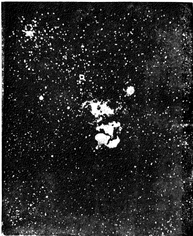
夏季南天人馬座之雲尾體氣，與冬天獵戶星雲相對峙。暗雲橫切而成三裂之形。即 NGC 6514 或 M20。
