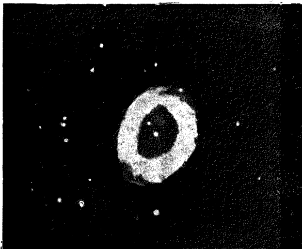
第二百三十二圖 天琴座 \beta 星與 \gamma 星間之大環狀星雲
