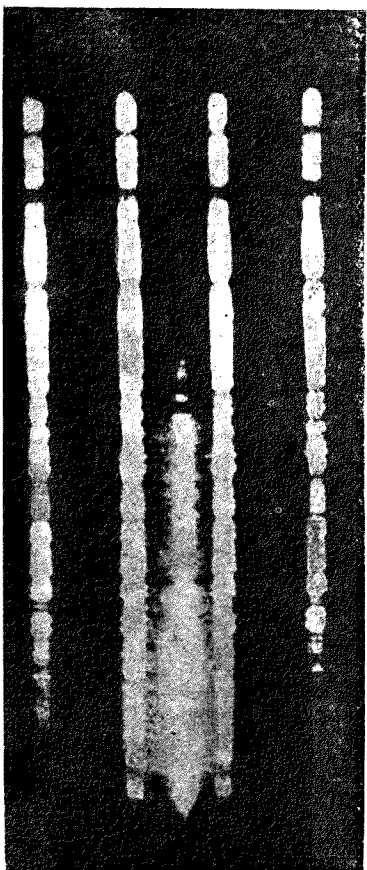
第二百四十三圖 仙女座大星雲之光譜
