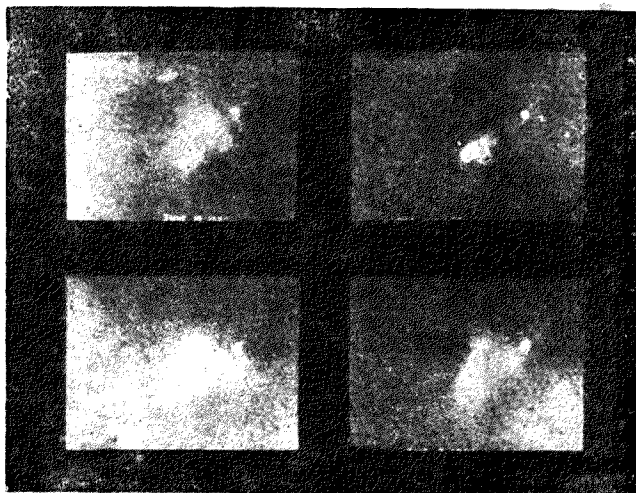
( 威爾遜山百英寸鏡 所攝), 攝影日期, 左上爲一九二〇年 六月十日, 左下爲同年八月十五日, 右上十月十一日, 右 下則在一九二一年八月八日。
