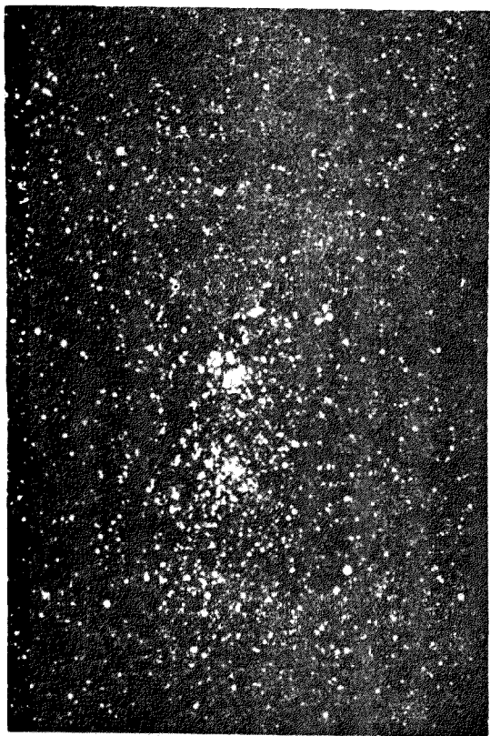
第二百十圖 英仙座二重星團
