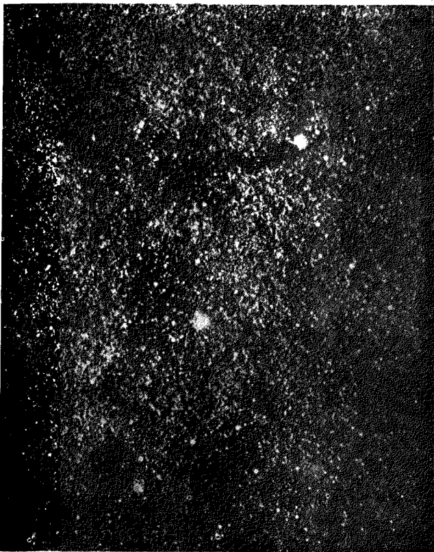
( 德國哈伊迪別天文臺長烏爾夫 所攝) 示暗黑星雲之存在
