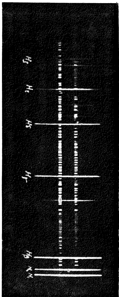
圖明 氫氣與未知星雲氣體爲顯明。
