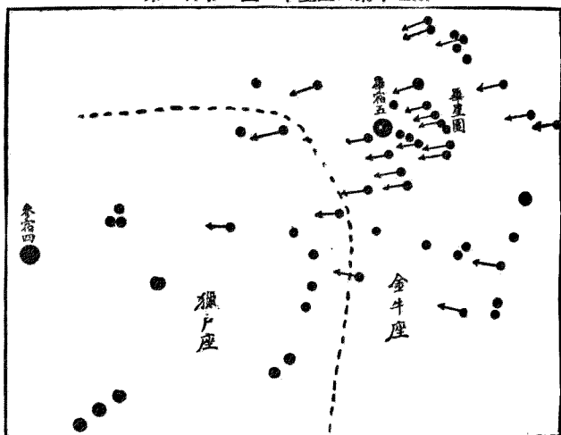
第二百零八圖 畢星團之集中運動
