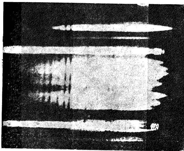
連續光譜中現多數晚期 法朗霍亞 線。
