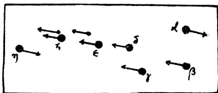
第二百零九圖 北斗七星之自行
