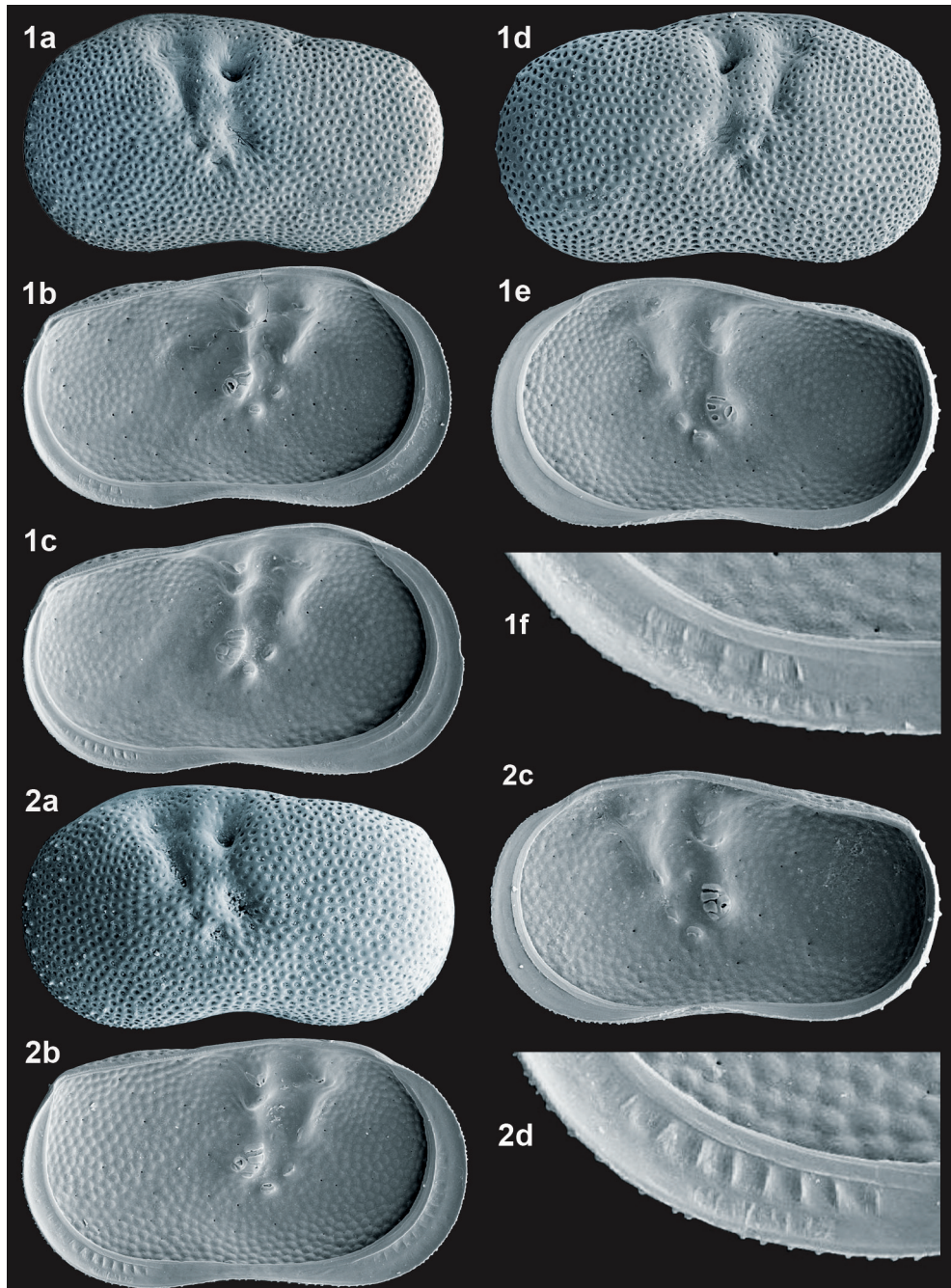
Ilyocypris biplicata (KOCH, 1838) – Neumark-Nord (40) fWaKz Weibchen: 1a - LVa (L 0,83), 1b - LVi (L 0,94), 1c - LVi (L 0,87), 1d - RVa (L 0,90), 1e - RVi (L 0,88), 1f - LVi (Ausschnitt posteroventral L 0,28).
