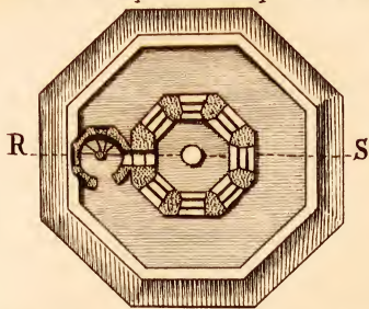
Plano del 4.º piso cortado por la línea NO.
