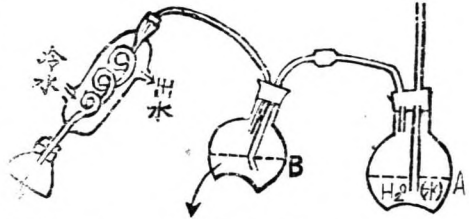
製氯化苦的裝置
