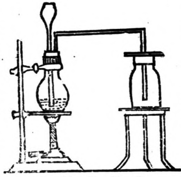
製氯的裝置
