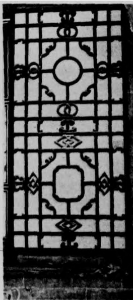
乙 汾陽峪道河某民宅 平窗帶臥簷方勝 工字等花頭
