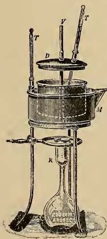
FIG. 393 ENGLER VISCOSIMETER.
