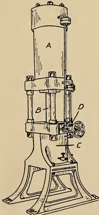
FIG. 252.—HYDRAULIC STRAINER.
