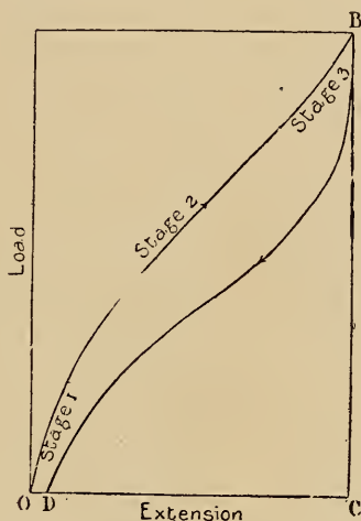
FIG. 415.—HYSTERESIS LOOP.
