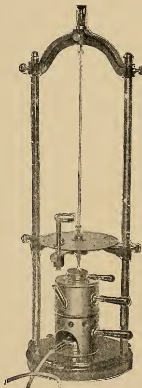
FIG. 394. DOOLITTLE VISCOSIMETER.
