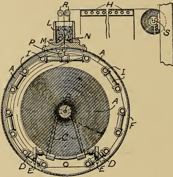
FIG. 230.—THE DESTRIKATS IMPREGNATOR.
