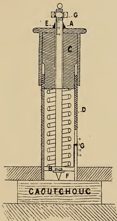
FIG. 419.—ELASTO-DUROMETER.
