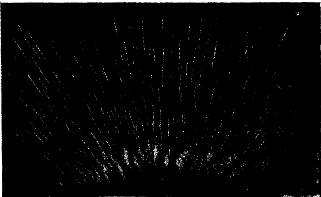
పటము ౨. రెండురకముల ధ్రువజ్యోతిర్భాసులు
