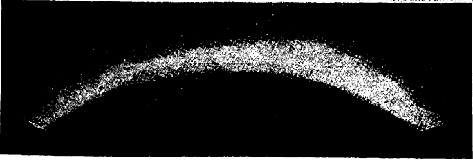
పటము ౧. రెండురకముల ధ్రువజ్యోతిర్భాసుస్సులు
