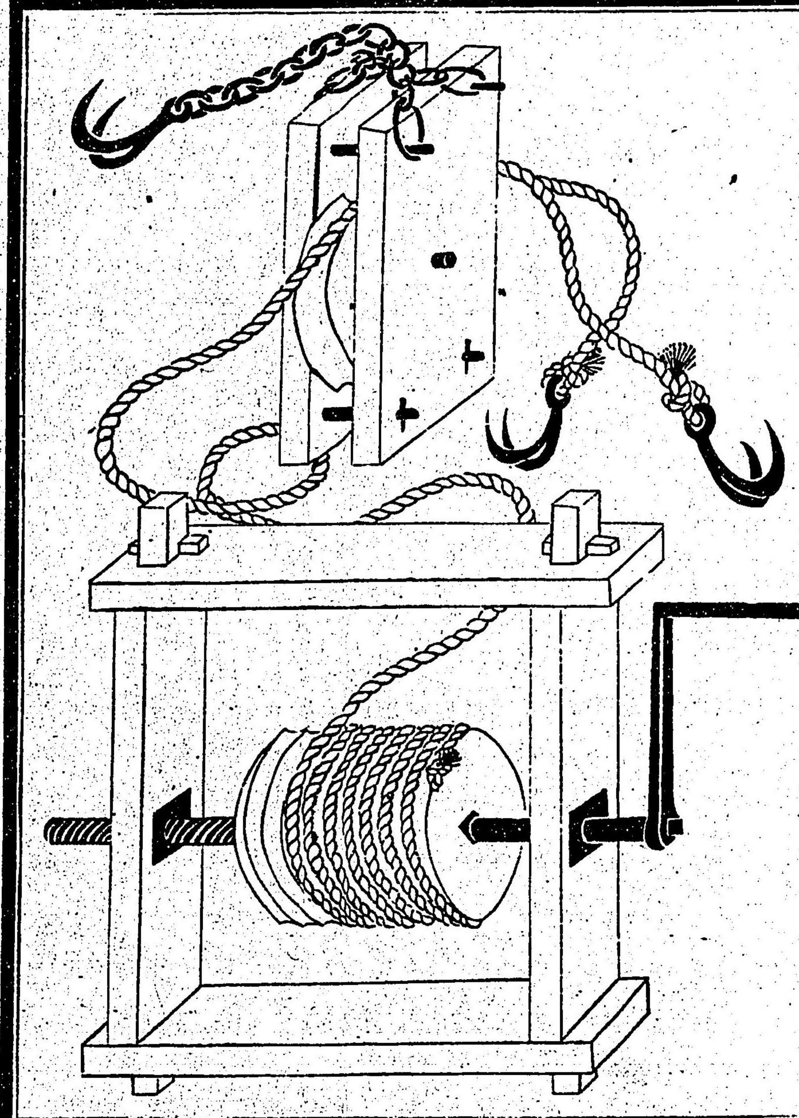
絞車之圖
