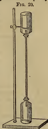
FIG. 20. Diffusion of gases.
