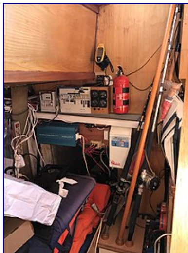
Couchette de quart tribord encombrée . Tableaux électriques, et commandes de batteries du moteur et des services.
