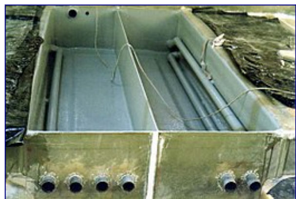
Pose des canalisations de remplissage et de vidange. Finition à la peinture époxy.
