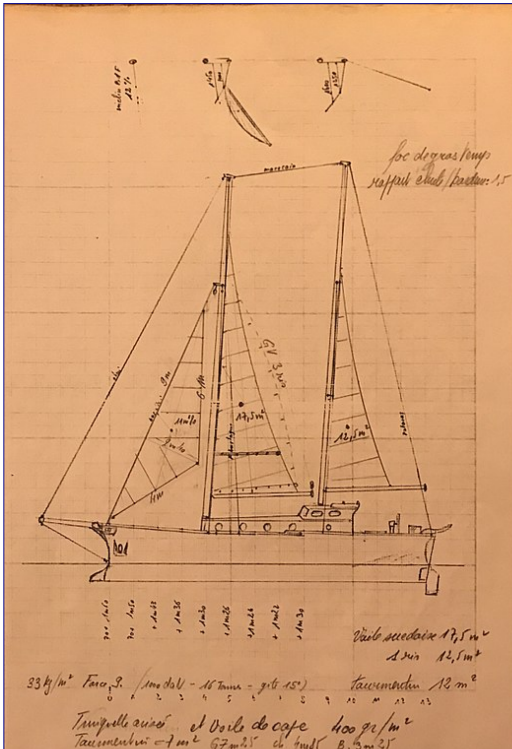
Plan de voilure réduite Force 8, F9 maximum si possible (Plans d'origine retrouvés en 2017)
