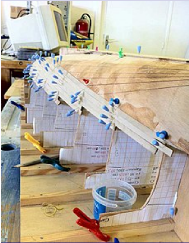
Découpe des baguettes pour le collage des œuvres mortes.
