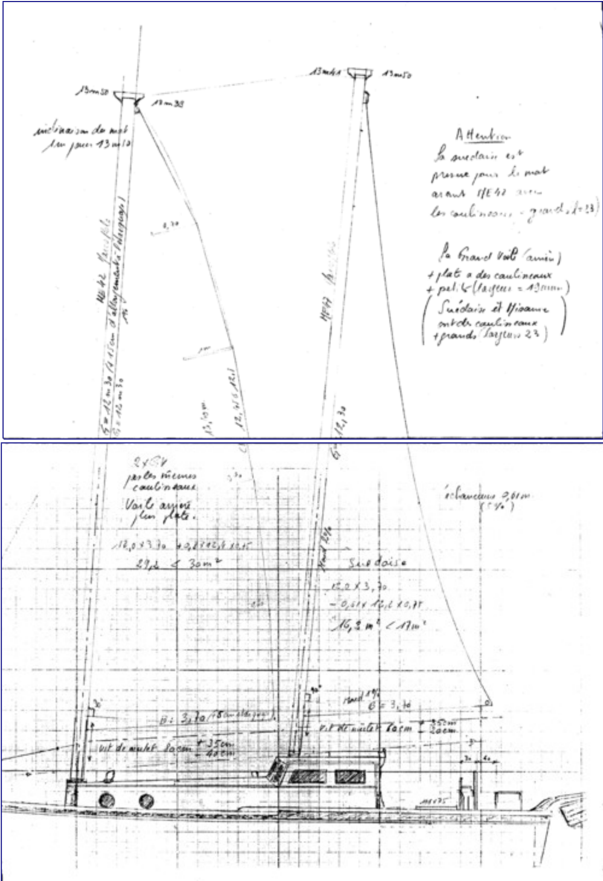
Plans de voiles d'origine (Commande à la voilerie Loize.).
