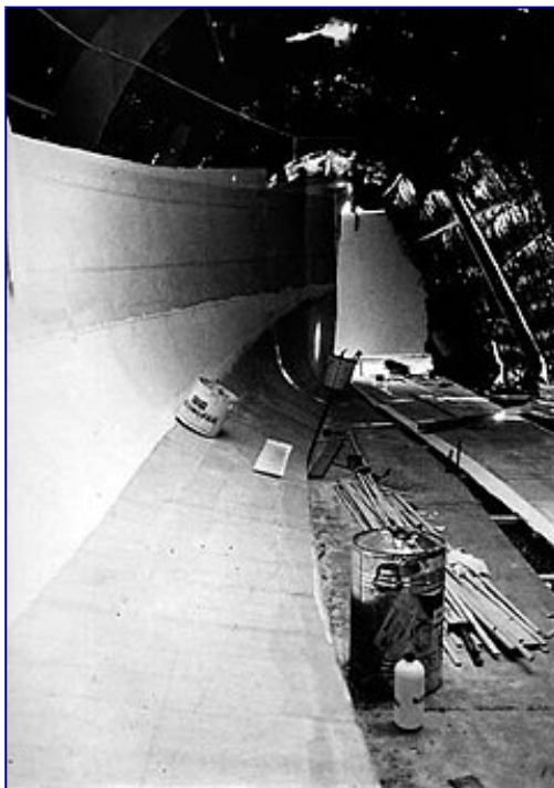
Stratification du bouchain après la pose des plaques de bordé et de carène.
