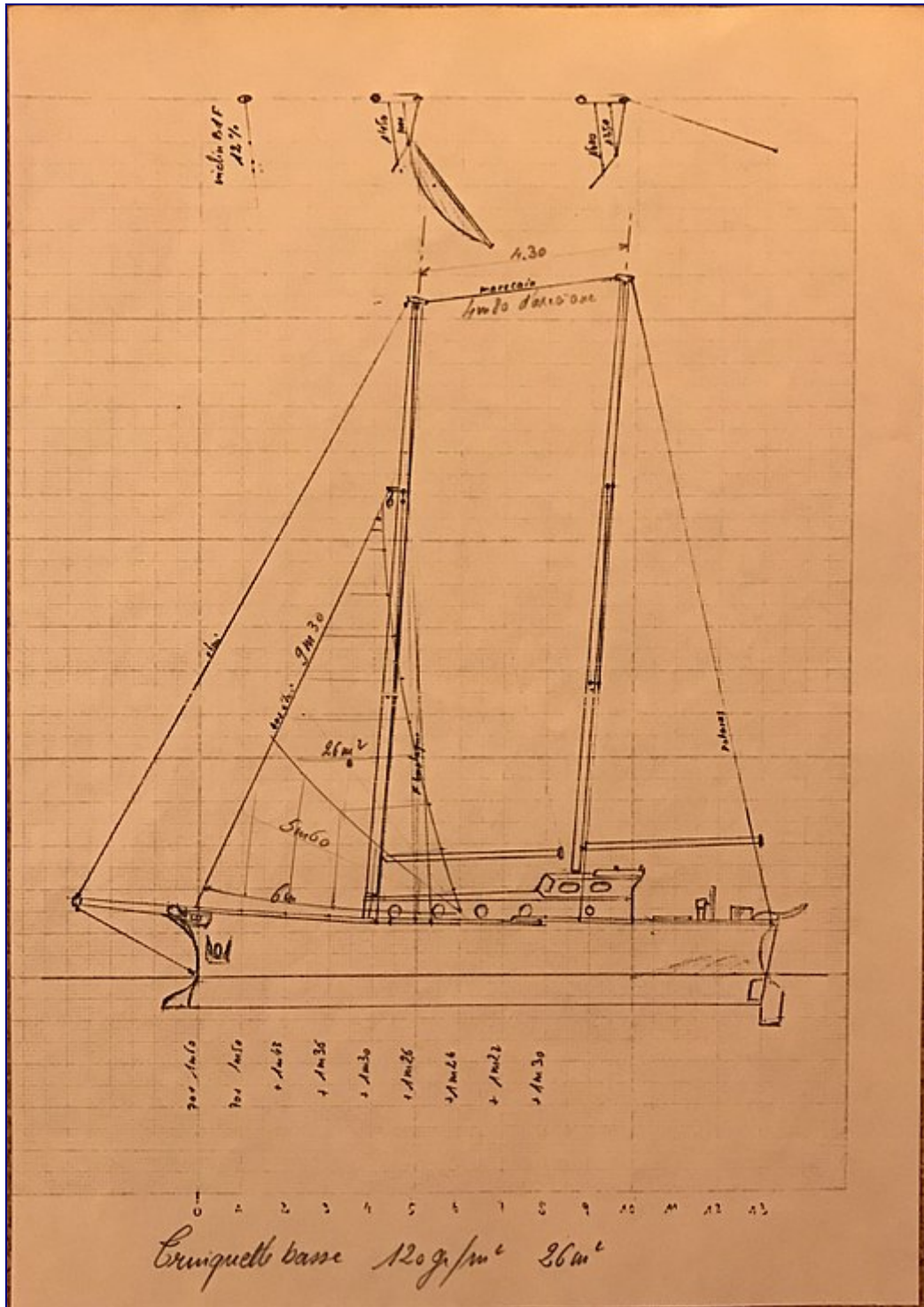
Trinquette basse (Plans d'origine retrouvés en 2017)
