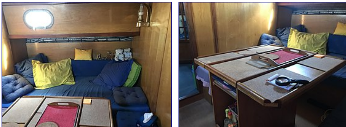
Aménagement du carré avec un lit double transformable en banquette. Table du carré avec les côtés rabattables.
