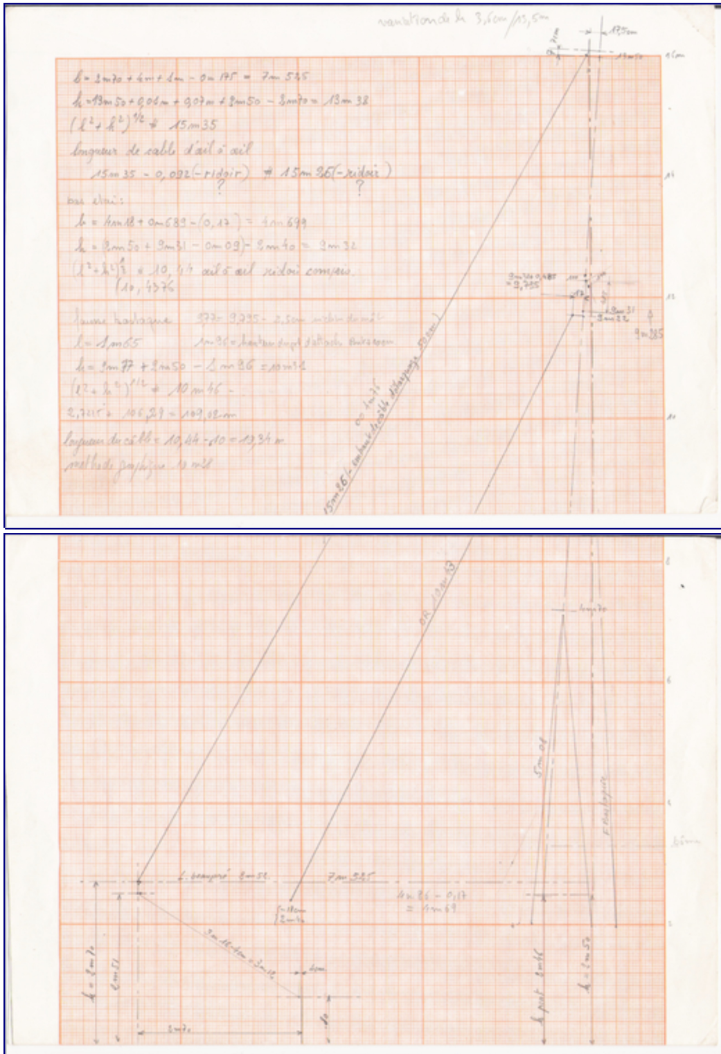
Calculs des longueurs d'étai
