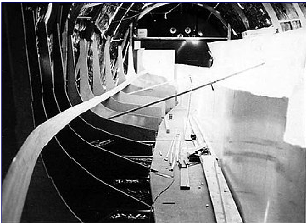
Pose des lattes de moulage sur les gabarits.
