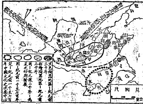
新石器文化之中心及仰光文化之次中心 仰光文化之範圍及仰光文化之發展 圖九第
