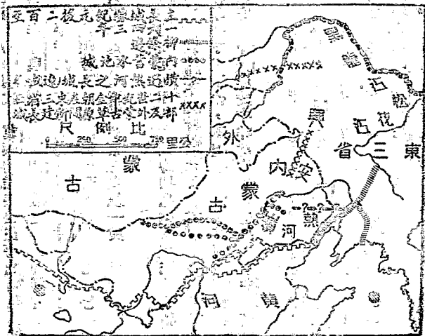
第一圖 城漢方北及城曼
