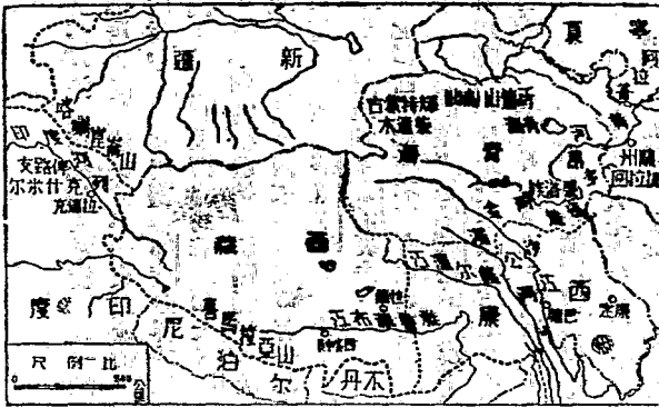
藏西 海青 藏西 圖八第
