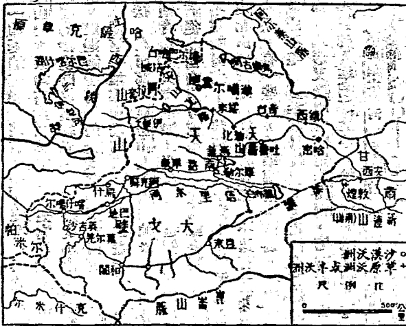
(新疆) 亞洲亞中屬中 圖七第
