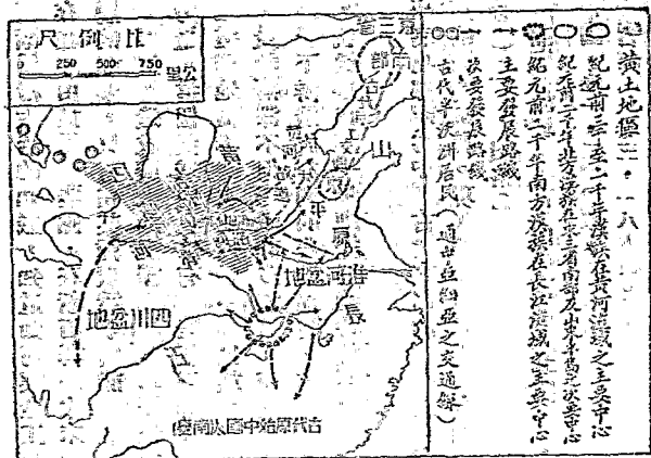
第四圖 紀元前二千至三千年間黃河及南方活動中心及發展路線
