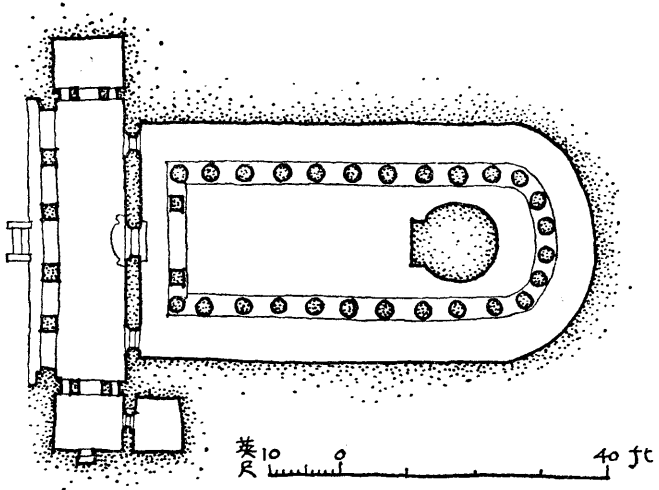
印度 Ajanta 第二十九支提摩平面 (Fergusson)
