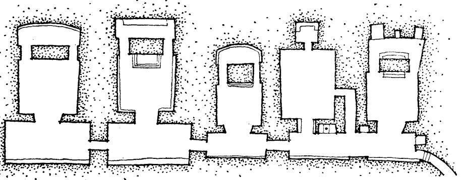
新疆 Kumtura 石窟平面 (Von Le Coq)
