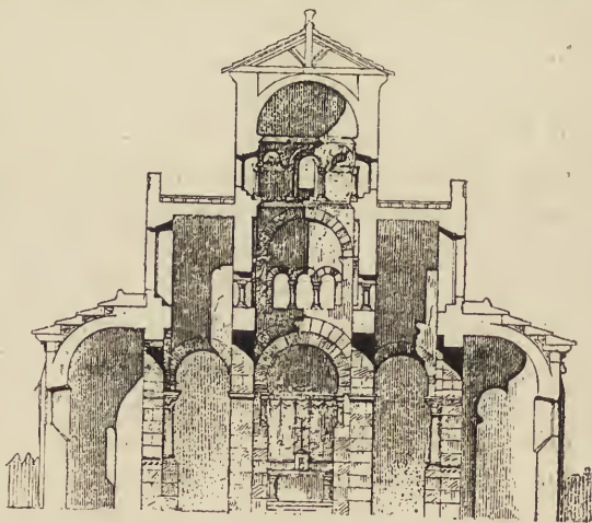
Abb. 28. Germigny-des-Prés, Kirche: Querschnitt. (Nach den Archives de la commission des monuments historiques, Tome, III, pl. 2.)
