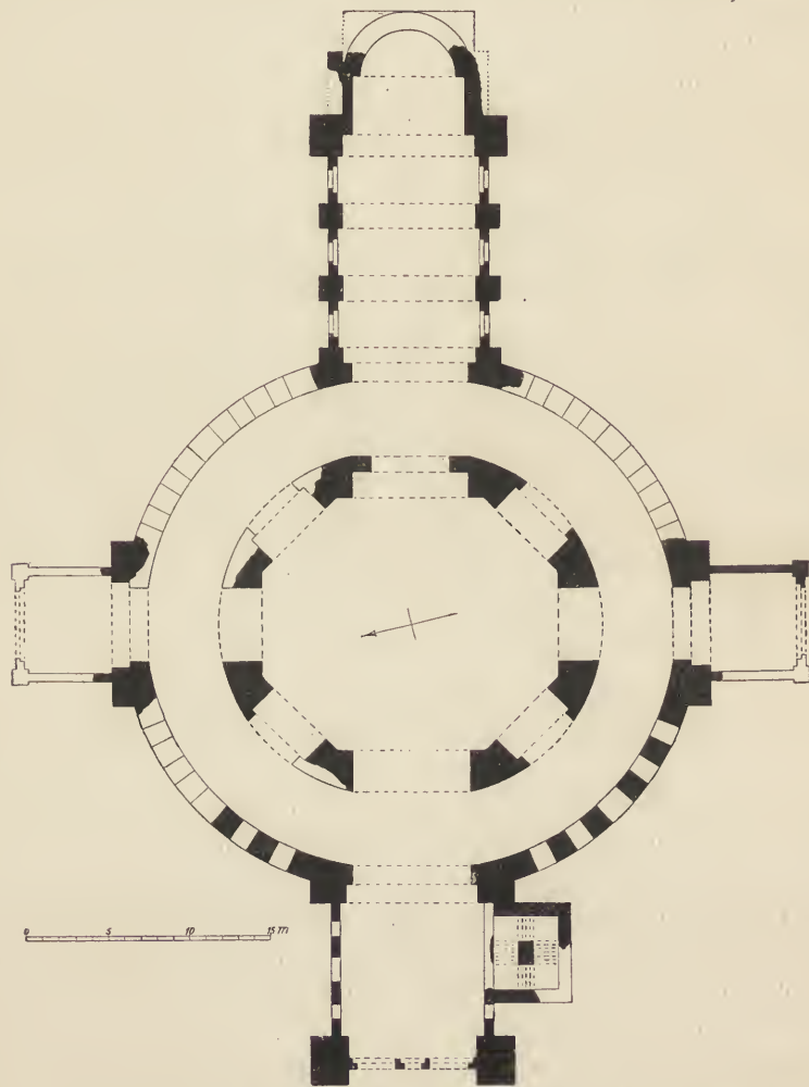
Abb. 23. Wiranschehr, Ovale Oktagon. (Aufnahme von O. Puchstein.)
