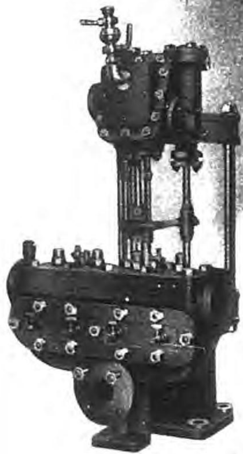
堅型ウォーターシントポンプ
