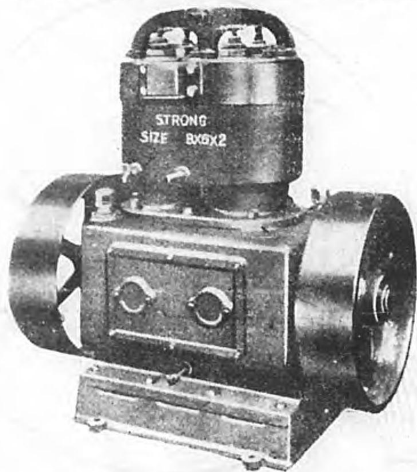
堅型空氣壓縮機
