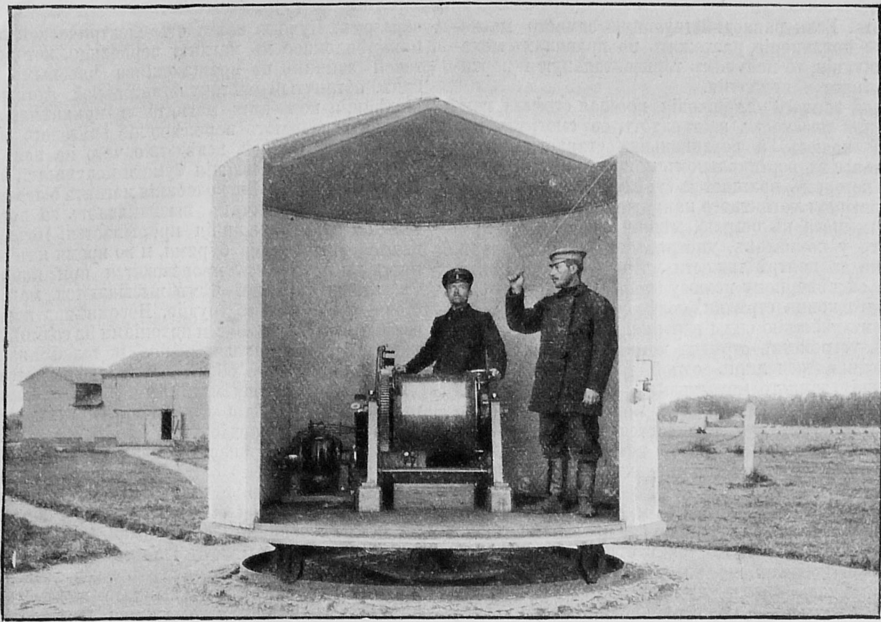
Желѣзный вращающійся павильонъ съ электрической лебедкой для подъема змѣевъ. На валу лебедки намотано около 14 километровъ стальной проволоки, къ которой прикрѣплены змѣи.
