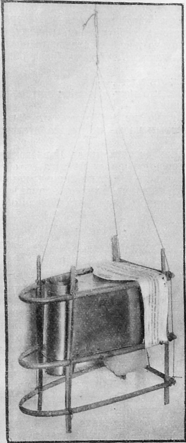
Метеорографъ системы В. В. Кузнецова для шаровъ-зондовъ.
