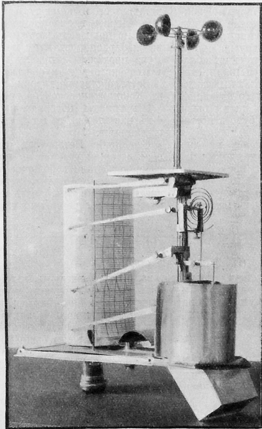
Общій видъ устройства метеорографа В. В. Кузнецова.
