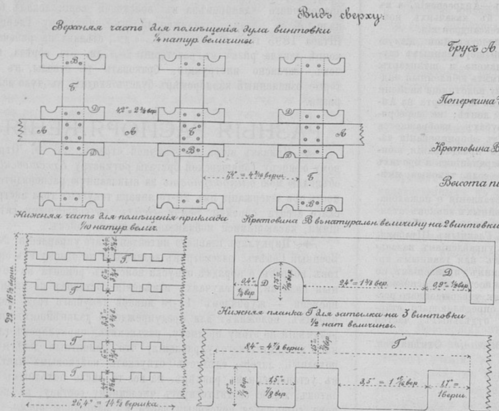
Пирамида для хранения 3-хъ-лин. винтовокъ.
