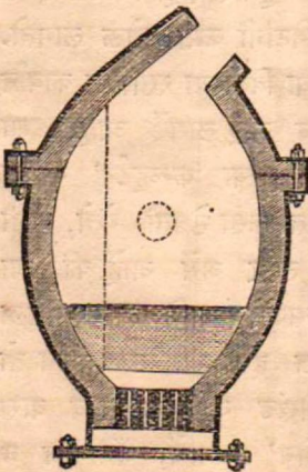
बेसेमर कन्व्हर्टर.
