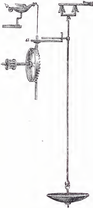
a. Voorstelling van den arm van de onrust, waarvan Huygens de eene helft afnam, om de andere met den slinger te verbinden.
