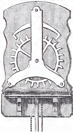
Model IV. Het Grahams anker.
