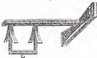
Cycloïde.
