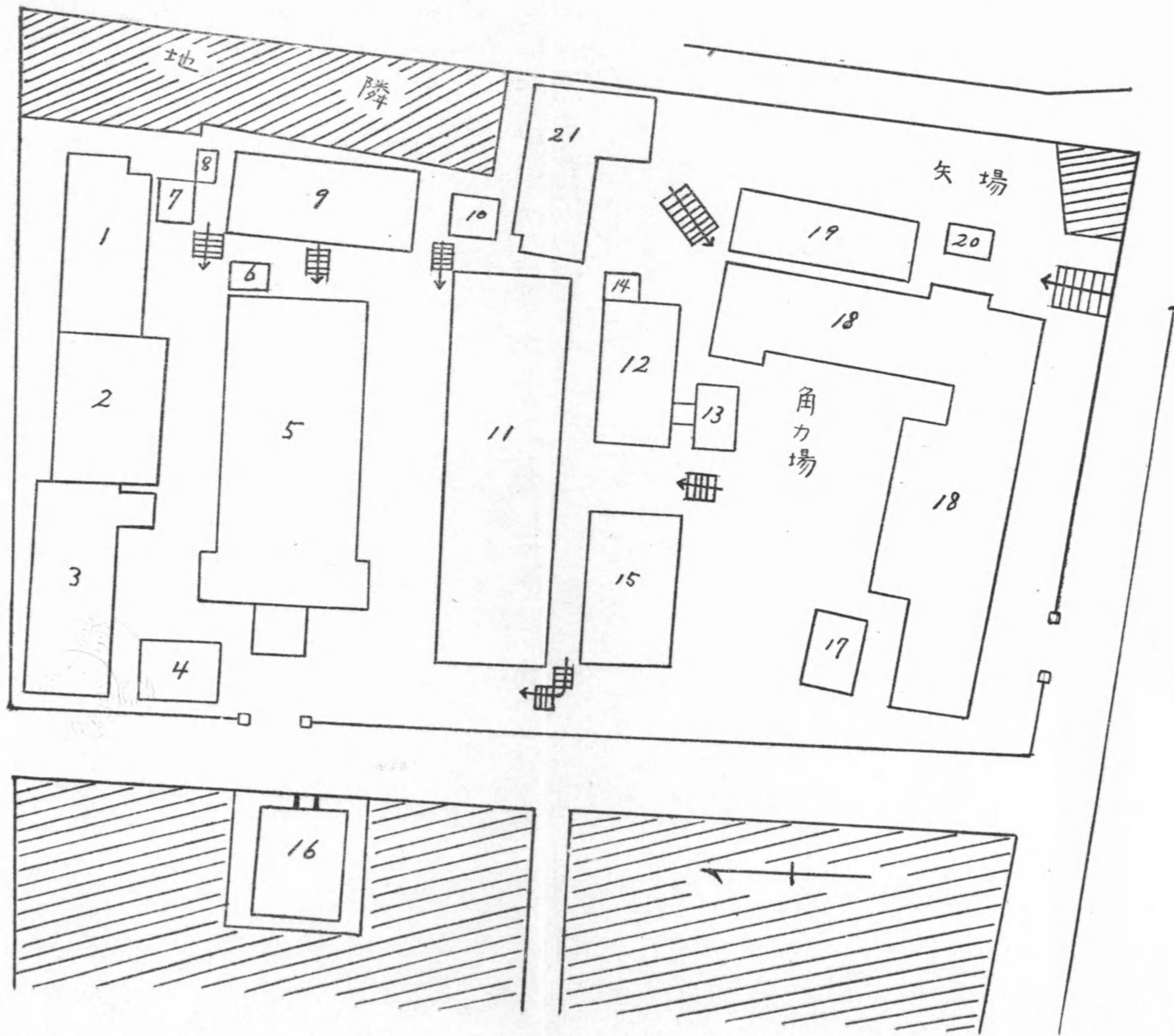
日本醫科大學校舍及附屬第二醫院配置圖
