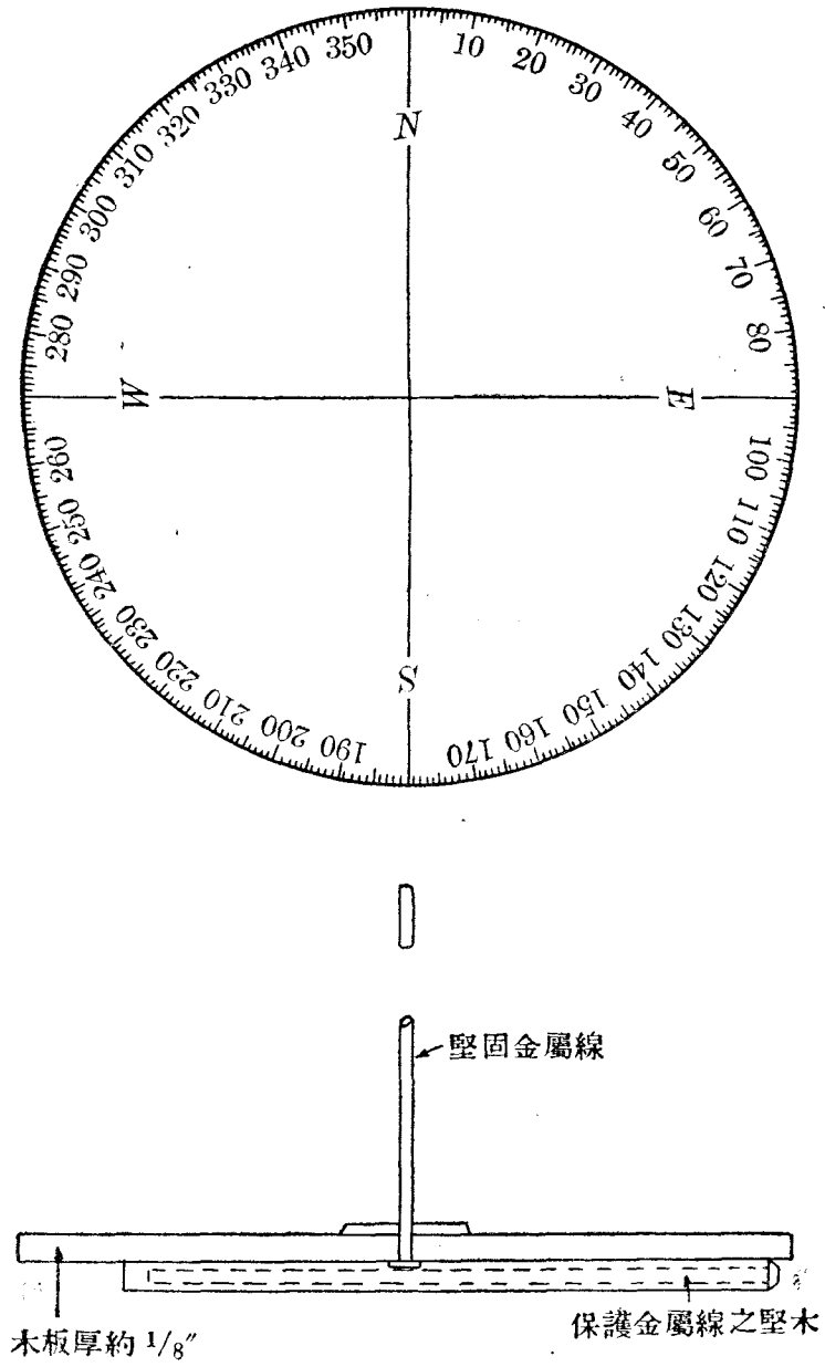
第三十五圖 日規
