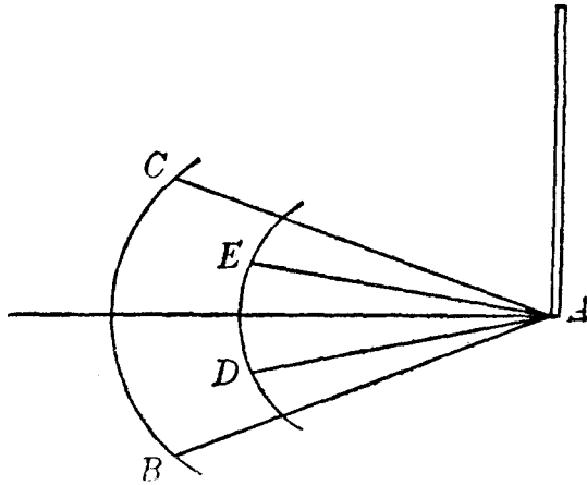
第二十二圖 用太陽求真南北方向
