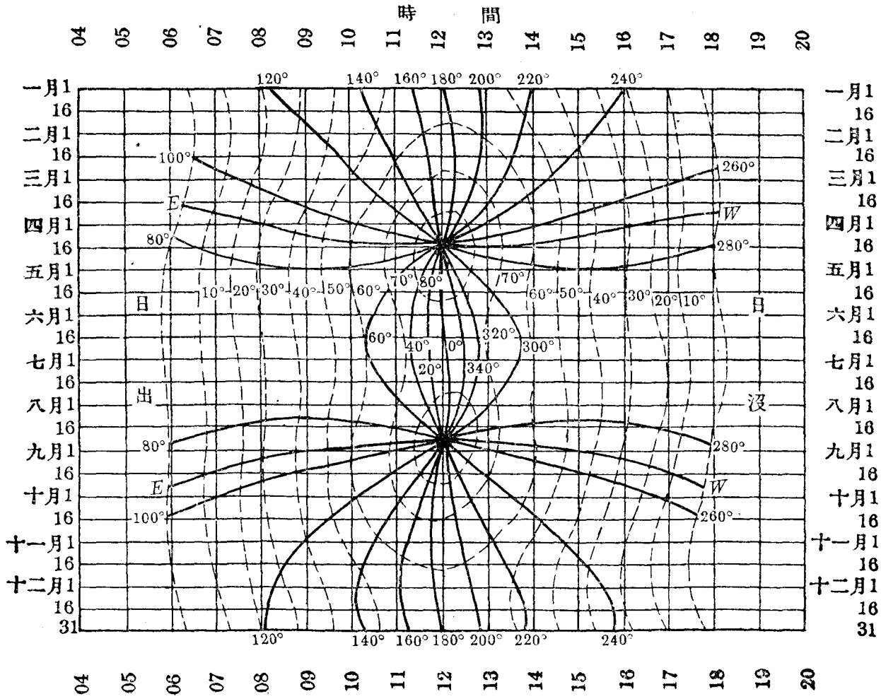
第二十九圖 太陽方位和高度(北緯 10^{\circ} ) 已經加上時差的訂正。若用標準時，應視本地經度在本時區標準子午圈的西或東多少度，每度加減四分；西加東減。夏時也要訂正。 實線表示方位，虛線表示高度。
