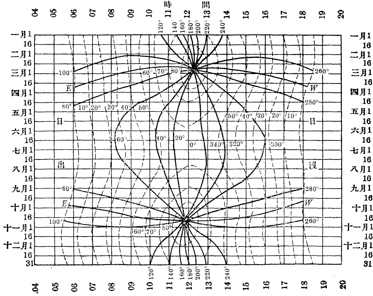
第三十一圖 太陽方位和高度(南緯 16^{\circ} ) 已經加上時差的訂正。若用標準時，應視本地經度在本時區標準子午圈的西或東多少度，每度加減四分；西加東減。夏時也要訂正。 實線表示方位，虛線表示高度。
