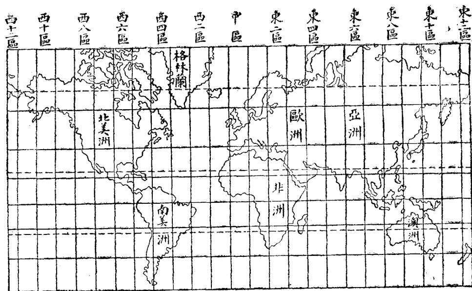
第十七圖 世界標準時區圖
