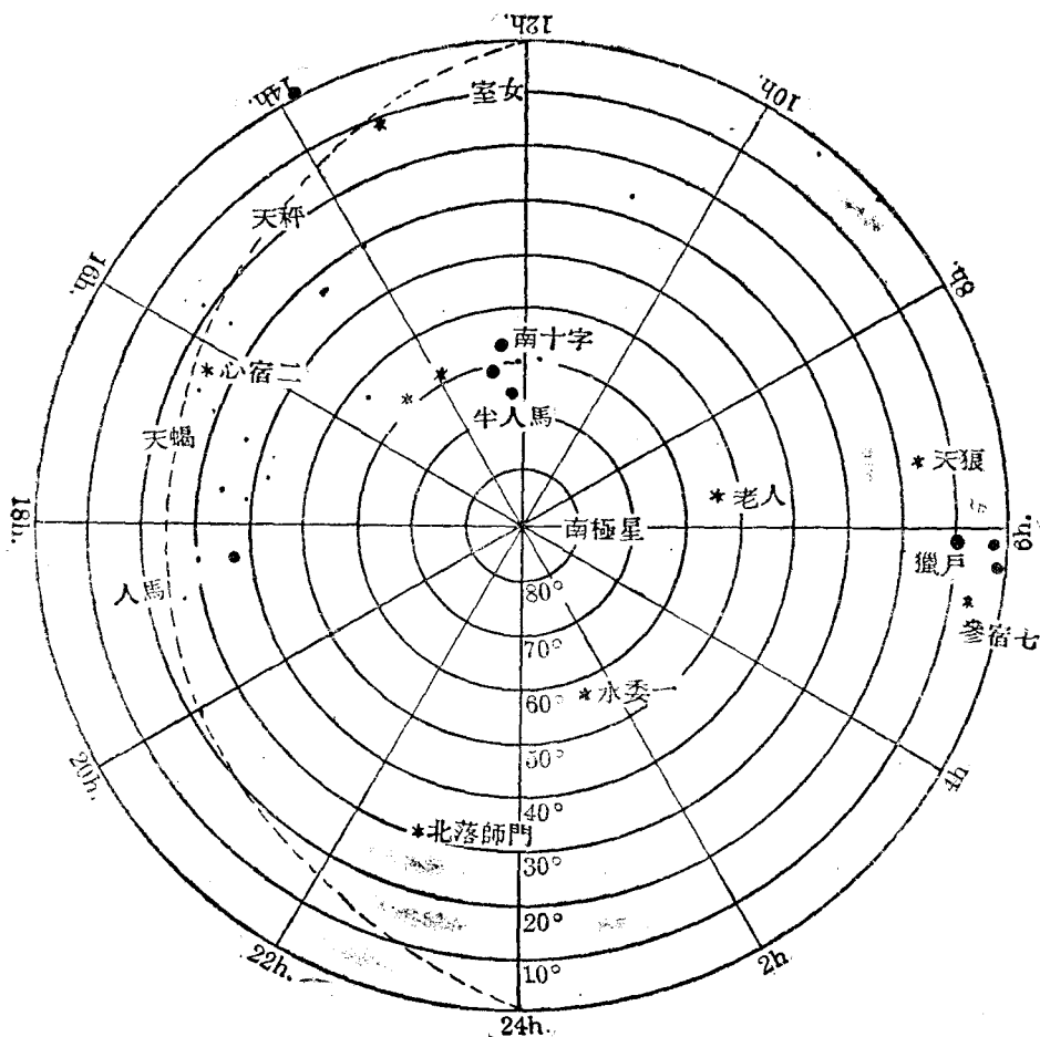
第二圖 南天主要星
