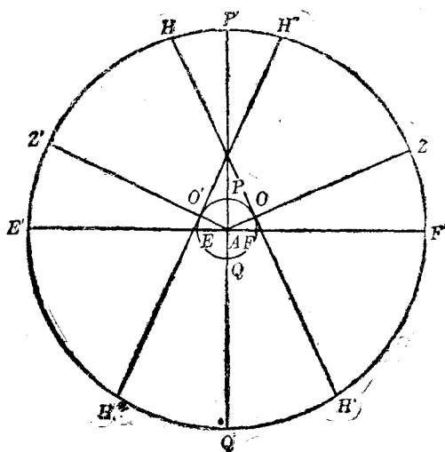
第九圖 出沒現象的說明
