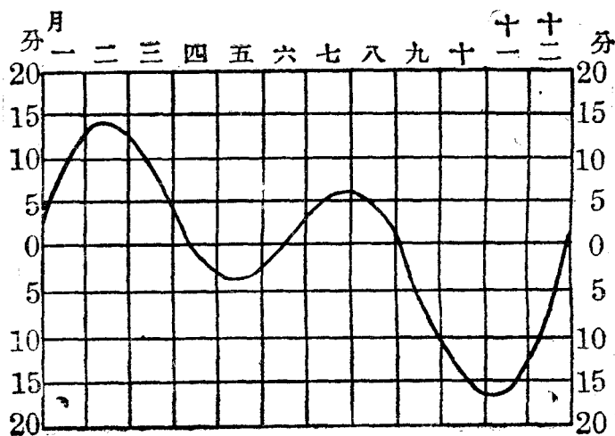
第十六圖 時差
