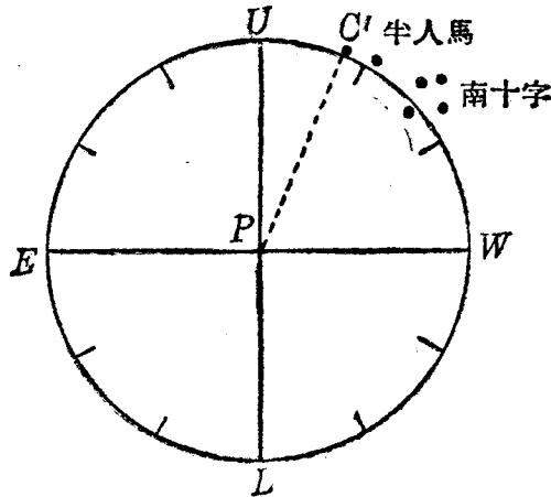
第四十八圖 半人馬座 \alpha 星的利用
