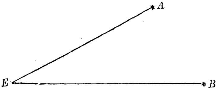
第十一圖 兩天體的角距
