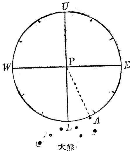
第四十三圖 大熊座 \alpha 星的利用 (一)
