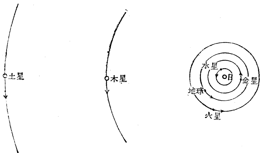
第五圖 太陽系六行星的距離
