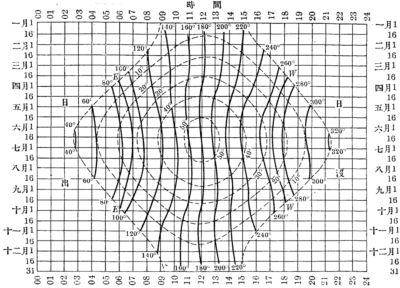
第二十四圖 太陽方位和高度(北緯 30^{\circ} ) 已經加上時差的訂正。若用標準時，應視本地經度在本時區標準子午圖 的西或東多少度，每度加減四分；西加東減。夏時也要訂正。 實線表示方位，虛線表示高度。
