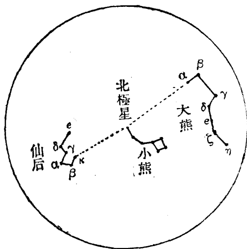
第三圖 北極星的認識
