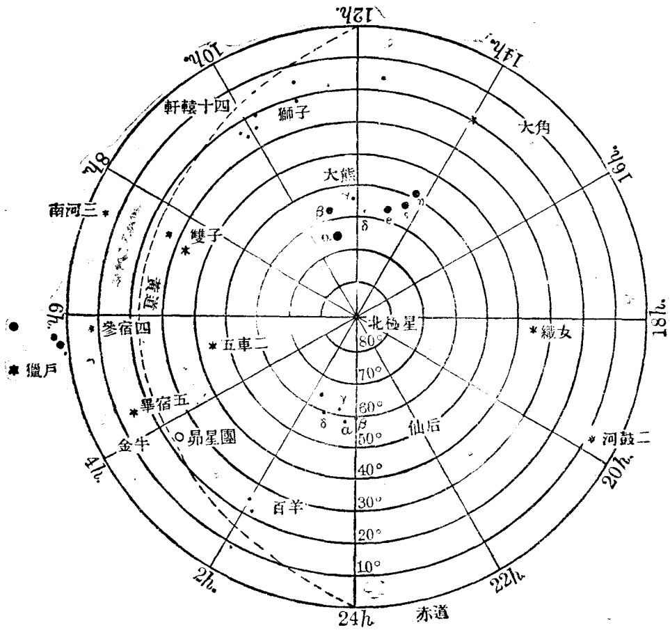
第一圖 北天主要星
