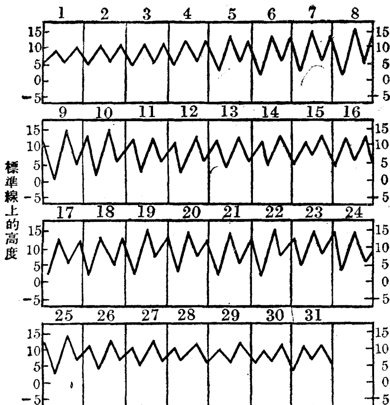
第四十一圖 1917年5月孟買潮汐高度
