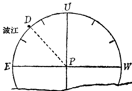
第四十九圖 波江座 \alpha 星的利用
