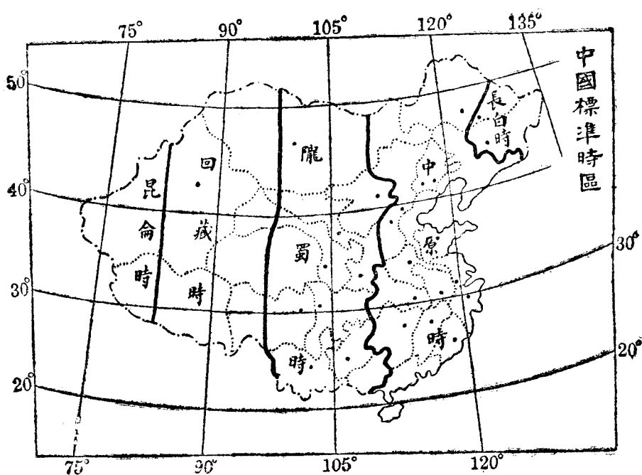
第十八圖 中國標準時區
