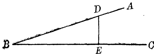
第十五圖 角的正切
