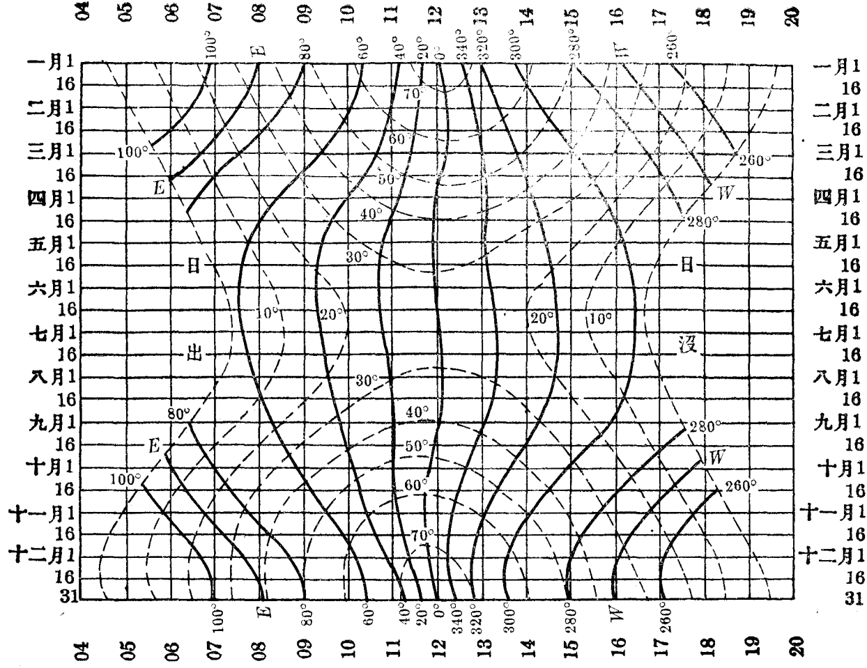
第三十四圖 太陽方位和高度(南緯 30^{\circ} ) 已經加上時差的訂正。若用標準時，應視本地經度在本時區標準子午圈的西或東多少度，每度加減四分；西加東減，夏時也要訂正。 實線表示方位，虛線表示高度。
