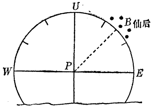
第四十七圖 仙后座 \gamma 星的利用
