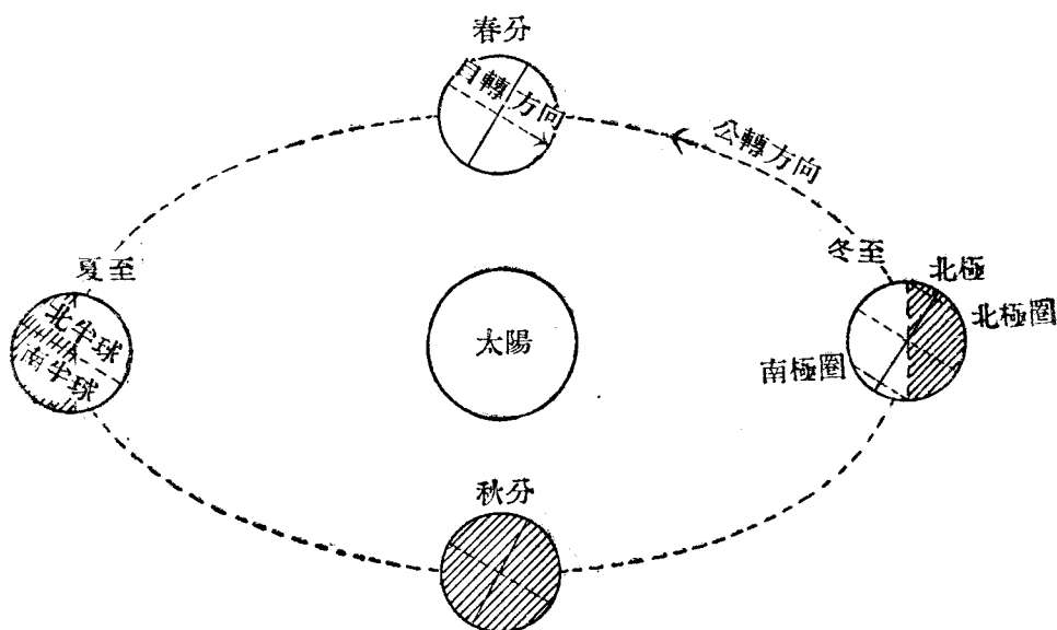
第十九圖 四季地球的位置
