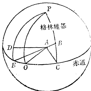
第十圖 經緯度的說明
