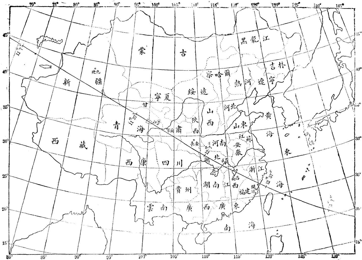
第三十七圖 民國三十年九月二十一日我國得見之日全食。
