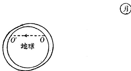
第四十圖 高潮的發生
