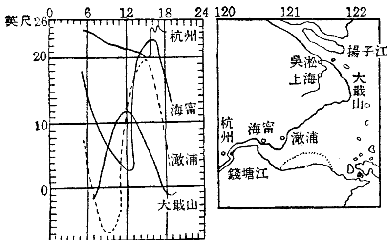
第四十二圖 杭州灣的潮汐 (1919年9月12日)
