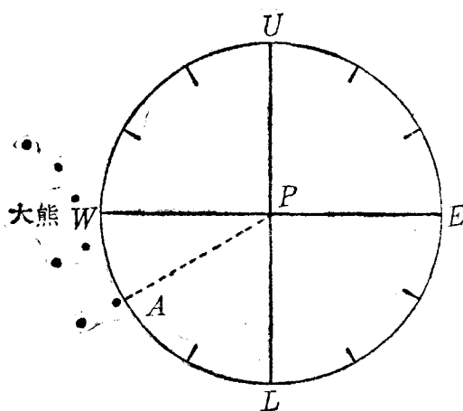
第四十四圖 大熊座 \alpha 星的利用(二)
