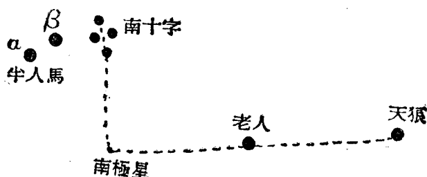
第四圖 南極星的認識
