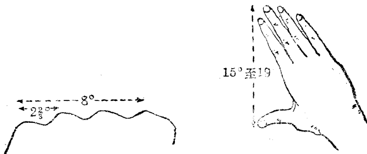
第十二圖 角度的估計方法
