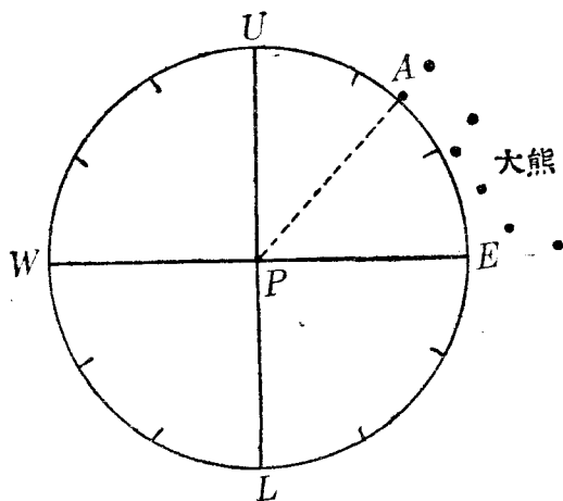
第四十五圖 大熊座 \alpha 星的利用(三)
