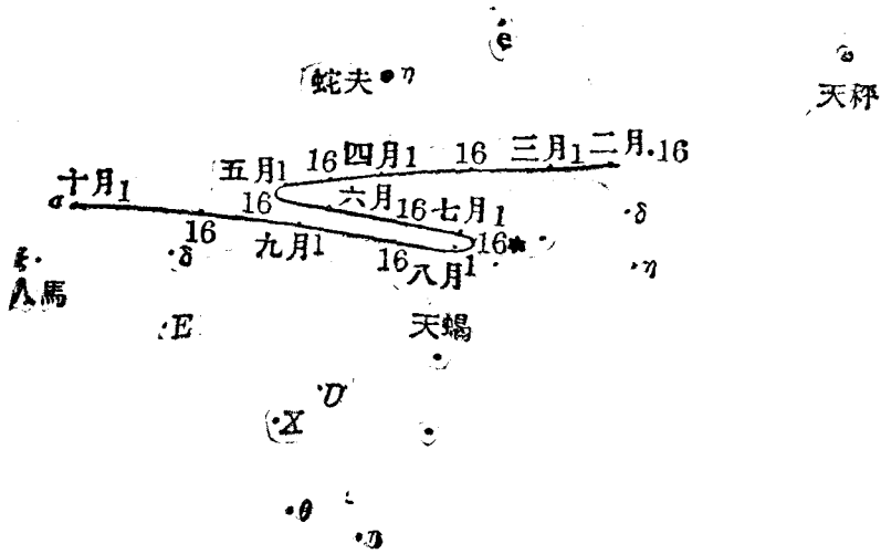
第六圖 一九二二年火星的視徑路
