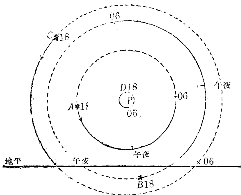
第七圖 星辰的視動(一)
