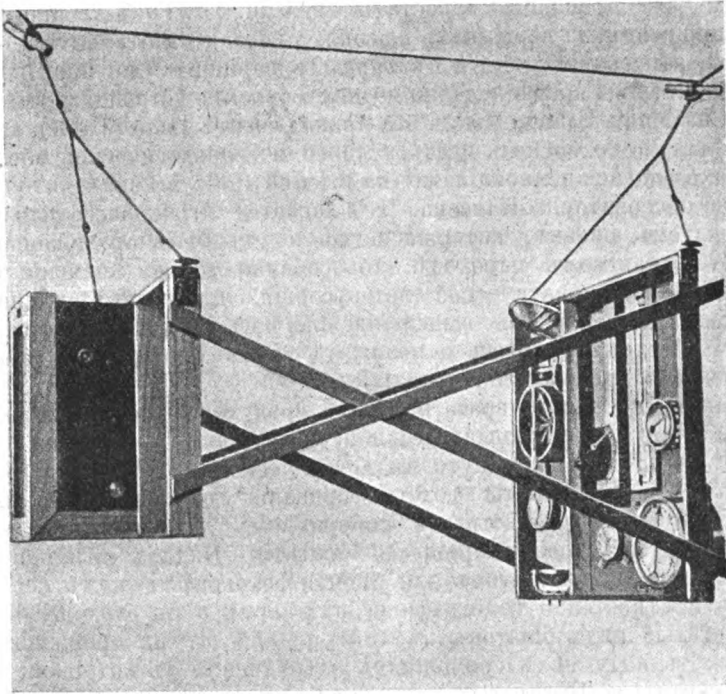
Рис. 88. Обсерваторія-зондъ Ванза.
