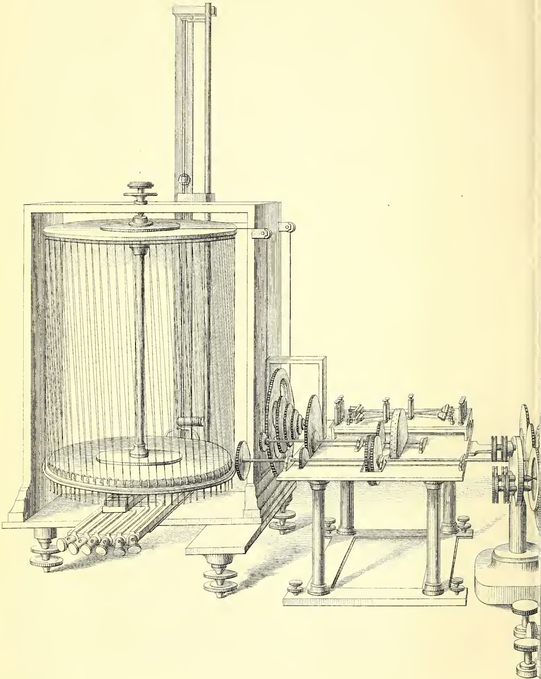
RHÉOCHORDE
