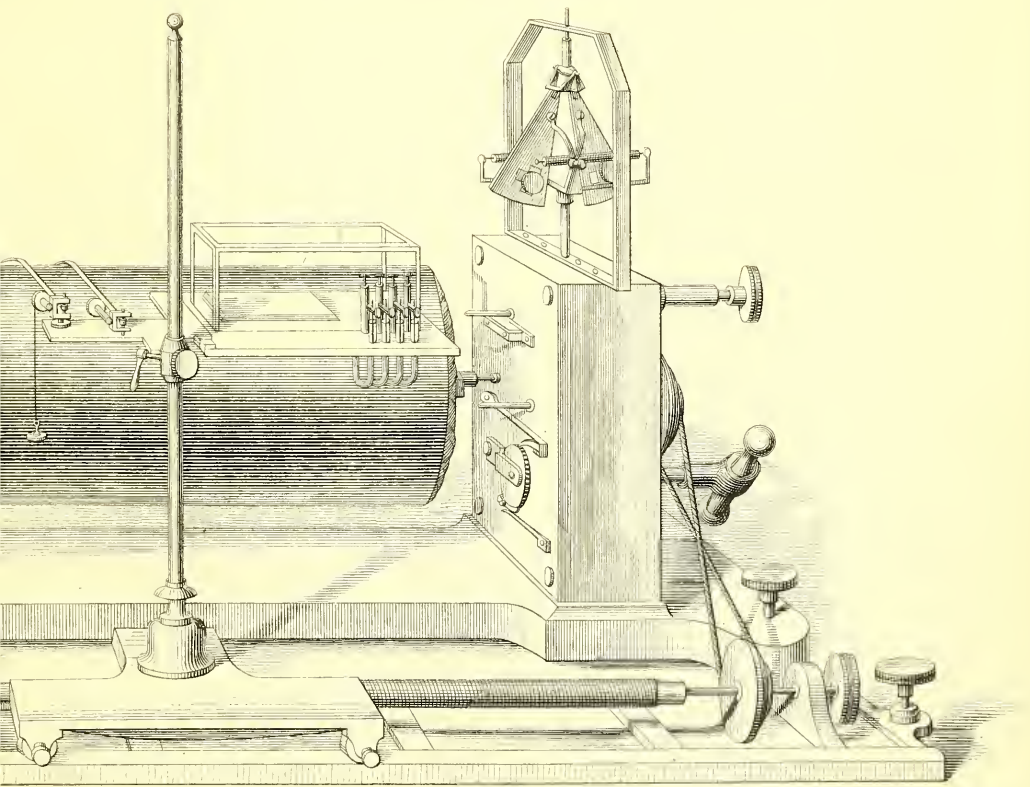
APPAREIL ENREGISTREUR
