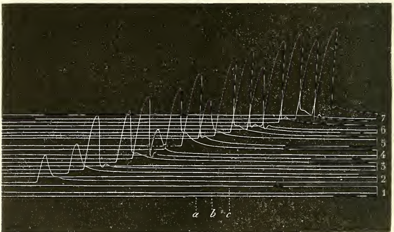
Fig. 9. — Excitabilité de trois points différents du nerf sciatique non sectionné. Pour chacune des intensités successives, l'excitation est faite dans l'ordre suivant : échancre sciatique, milieu de la région fémorale, bifurcation. 20, Daniell, 1 micros. Réoch. de 50 en 50 cent. Pôle négatif sur le nerf.
