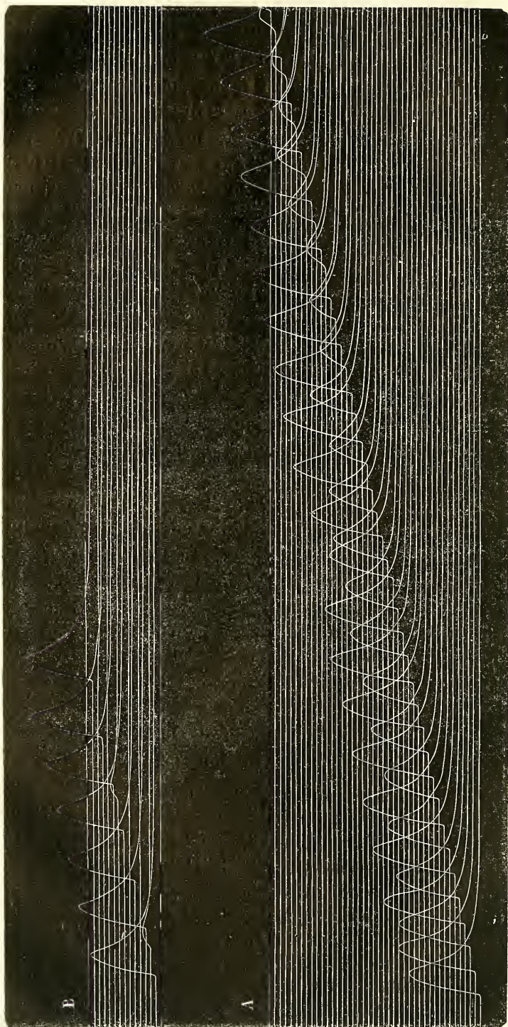
Fig. 21. — Diminution progressive et disparition de la secousse produite par le courant ascendant, pendant le dépolarissement du nerf. Intensité constante à peine supérieure à la minima (2 El. Daniell, n° 2 du Rhéochorde). — Le tracé B, pris cinq minutes après A, lui fait suite, et montre la suppression complète de la contraction par courant ascendant. Dans les deux tracés, la ligne la plus inférieure répond au courant asc. — Commutation après chaque excitation.
