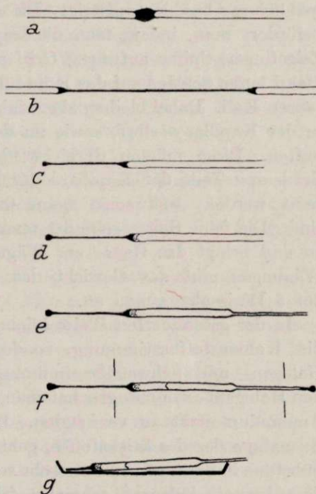
Fig. 15. Anfertigung der Kapillare zum Abwägen der Flüssigkeiten. (Natürl. Größe.) a) Bildung eines Glastropfens in der Mitte, b) Ausziehen desselben, c) Eine Hälfte des in der Mitte durchgeschmolzenen Stückes, d) Nachdem ein Kristall \text{KClO}_3 am Boden angeschmolzen und e) sein offenes Ende zu einer Kapillare ausgezogen worden ist (I. Wägung), f) Nach dem Einfüllen der Flüssigkeit und dem Zuschmelzen, g) Die Kapillare nach Abschneiden des Griffes und Abbrechen der Spitze auf dem Platinblech liegend, im Momente der Einföhrung in das Verbrennungsrohr.
