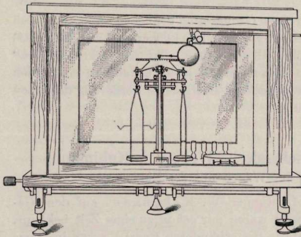
Fig. 1. Mikrochemische Wage.
