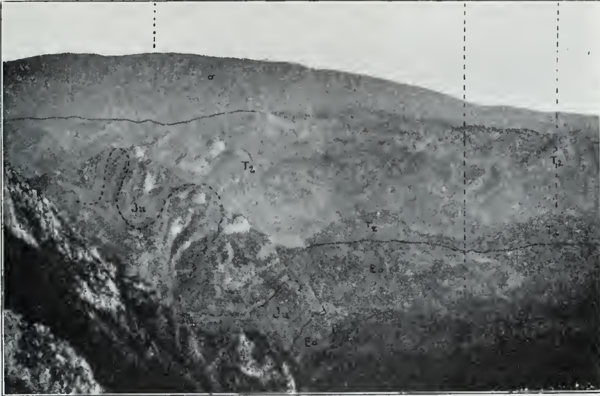
Fig. 1. Posteoocäne Falten der Maja Gušs.
