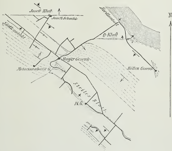
Geologischer Plan des IX. Laufes der Südostgrube. 1:5760.
