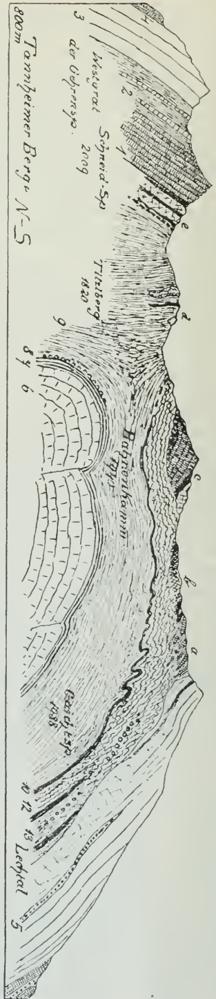
Fig. 6. Profil von der Gaidtspitze zur Tannheimer Kette nach den Aufschlüssen der Westseite.
