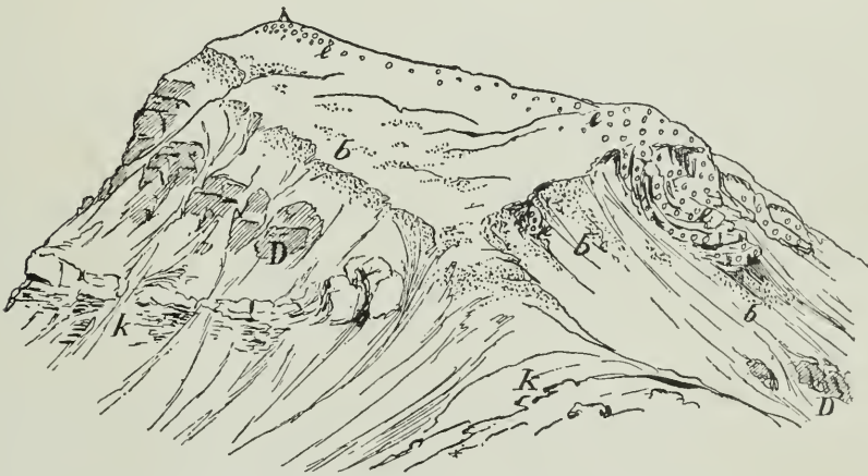
Fig. 4. Gipffläche des Jaggl, gesehen vom Hengst.
