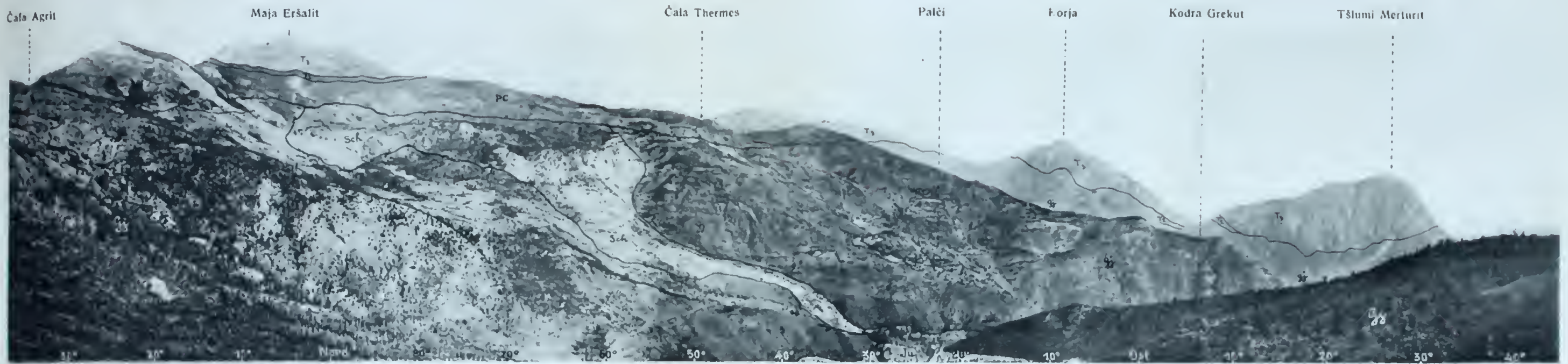
1. Panorama von Kroni Planave unweit Bridža im Gebiete von Palči. Ju = Jurassischer Plattenkalk. Gj = Gjanischiefer. Pc = Permocarbon. T 2 = Mittlere Trias. T 3 = Obere Trias. Sch = Schutt eines recenten Bergsturzes.
