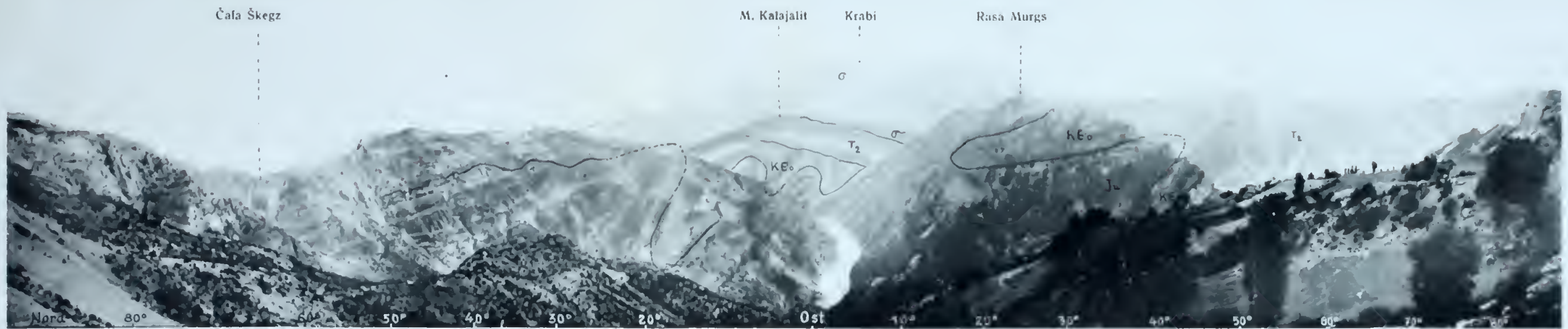
1. Drinatal bei Čereti Vilz Eper. Eocän (KEo) und Jura (Ju) gefaltet, darüber mittlere Trias (T 2 ) und darüber Serpentin ( \sigma ).
