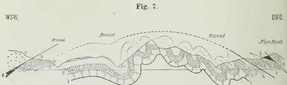
Idealprofil durch die Hauptfalten des Cukali.
