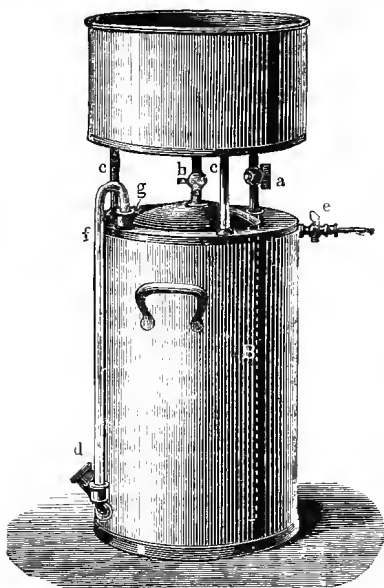
FIG. 23.—Gasholder.
