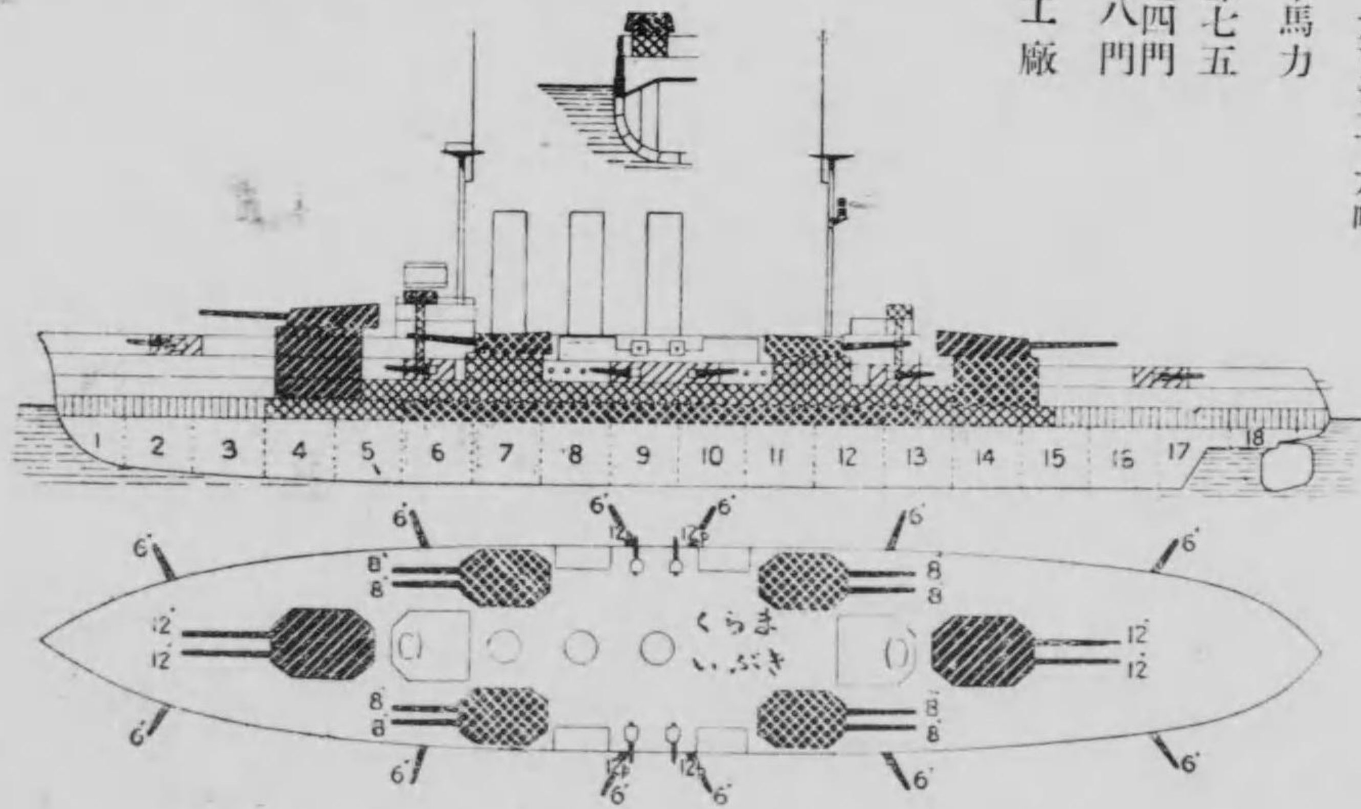
伊吹、馬鞍 及平面圖 長艦 四〇五呎 艦幅 七五呎 吃水 六十二呎
