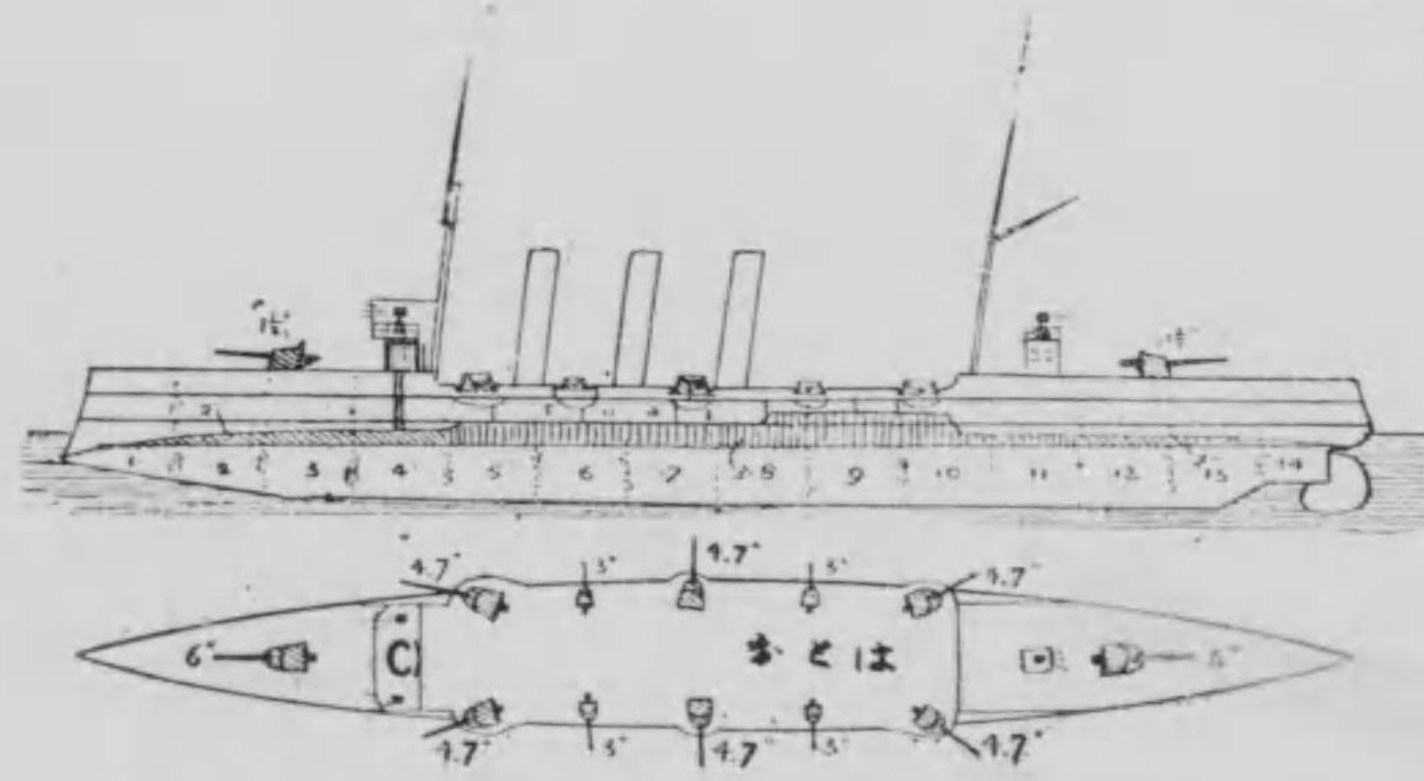
音羽 平面及側面圖 艦長三五尺一 艦幅四一尺 吃水六一尺
