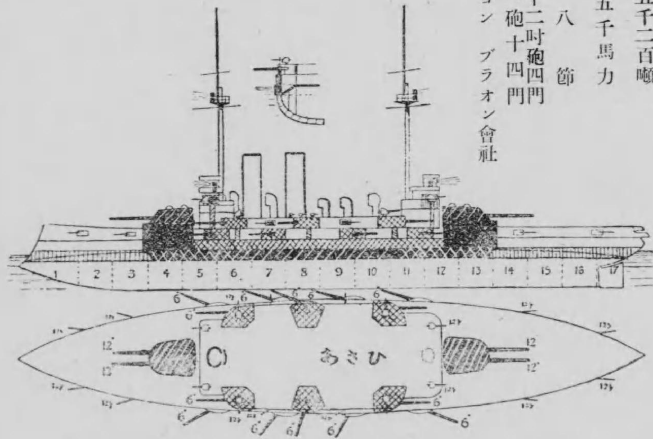
朝日艦 平面及側面圖 長 四一五呎 寬 六十七呎 吃水 八二呎
