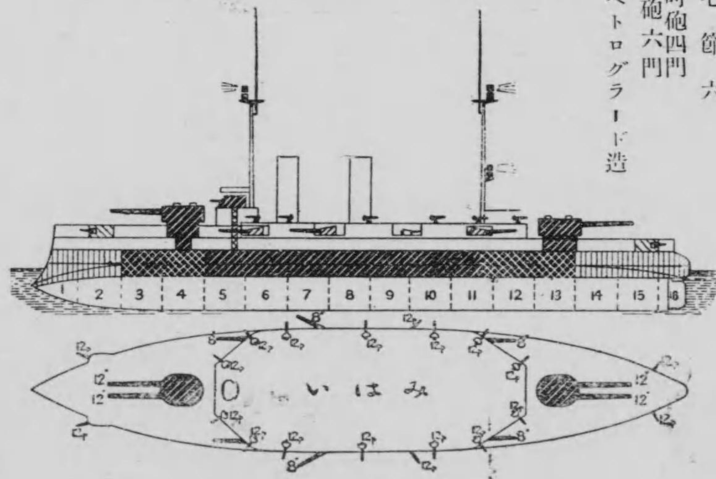
石見 平面及側面圖 艦長三十七呎六寸 艦幅七呎六寸 吃水六呎二寸
