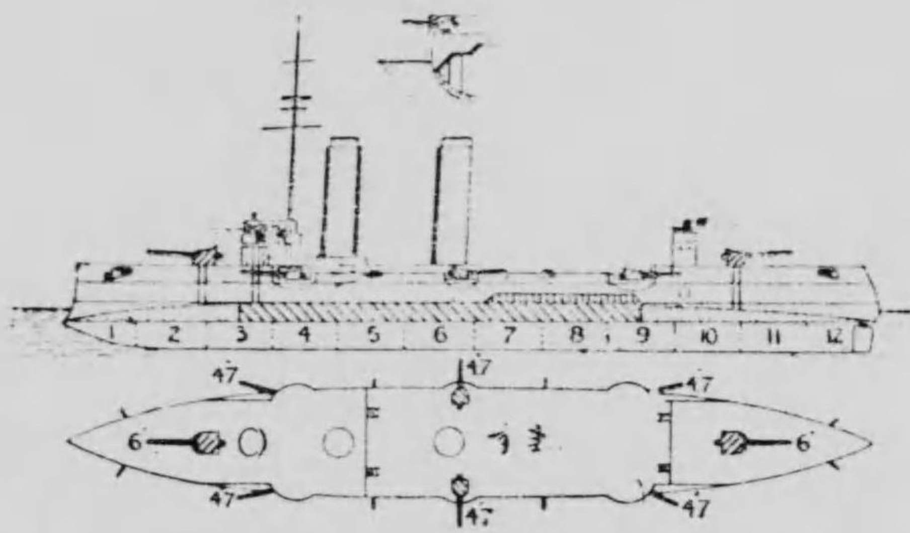
須磨 平面及側面圖 艦長五〇呎 幅四一呎 吃水六呎
