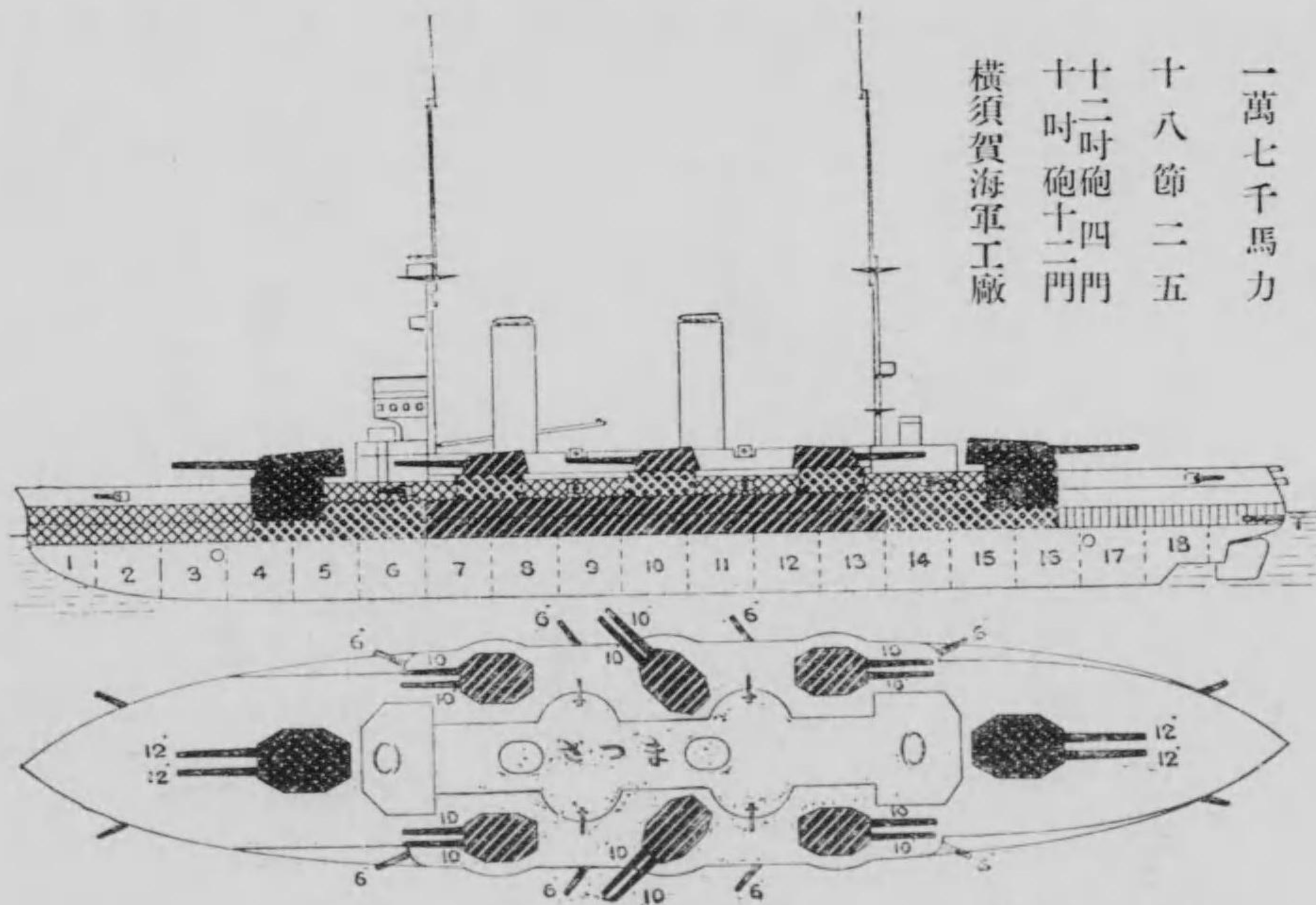
戰艦薩摩 平面及側面圖 艦長四七九呎 艦幅三八呎 吃水二八呎
