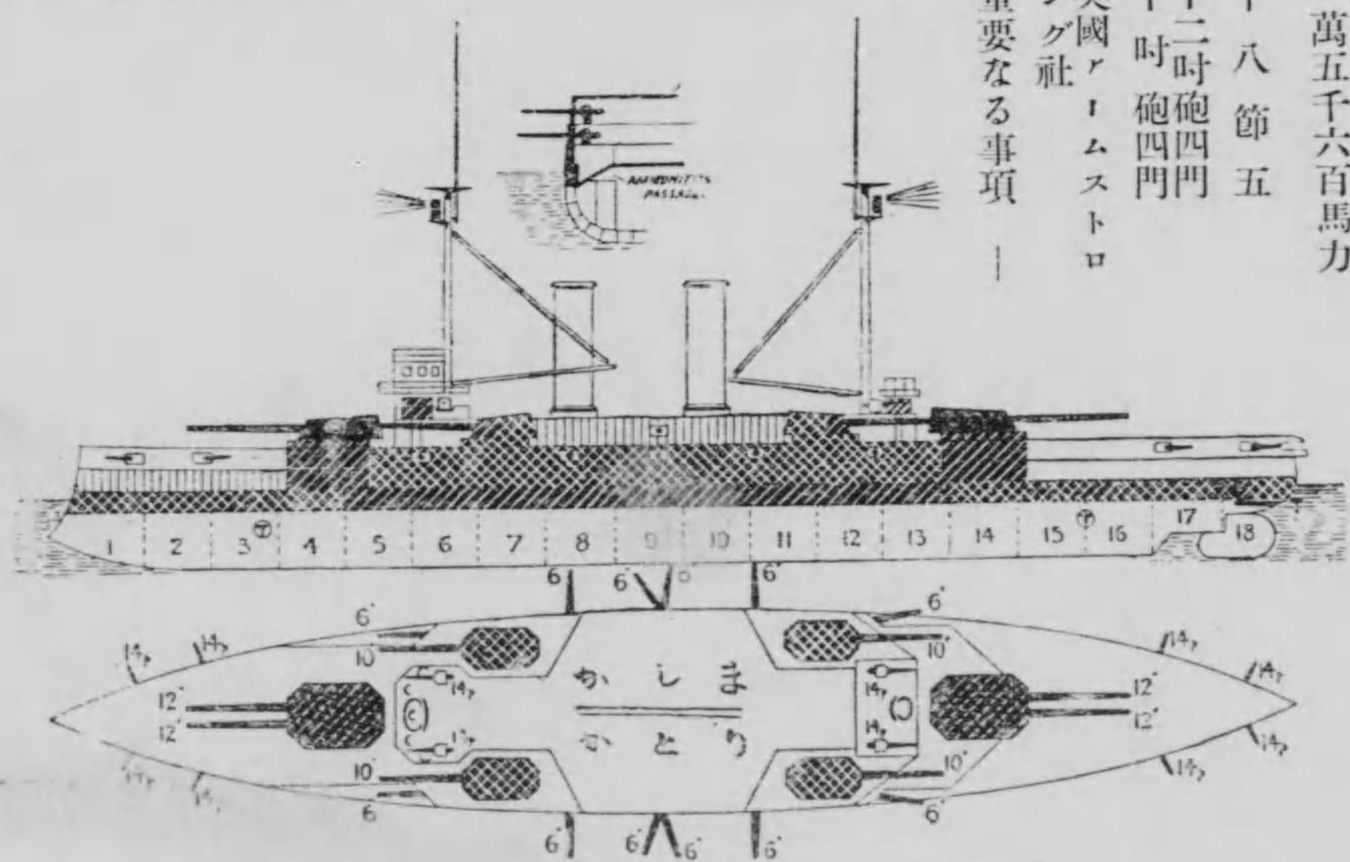
戰艦鹿島 平面及圖面 艦長四十五呎 艦幅七呎八吋 吃水六呎二吋
