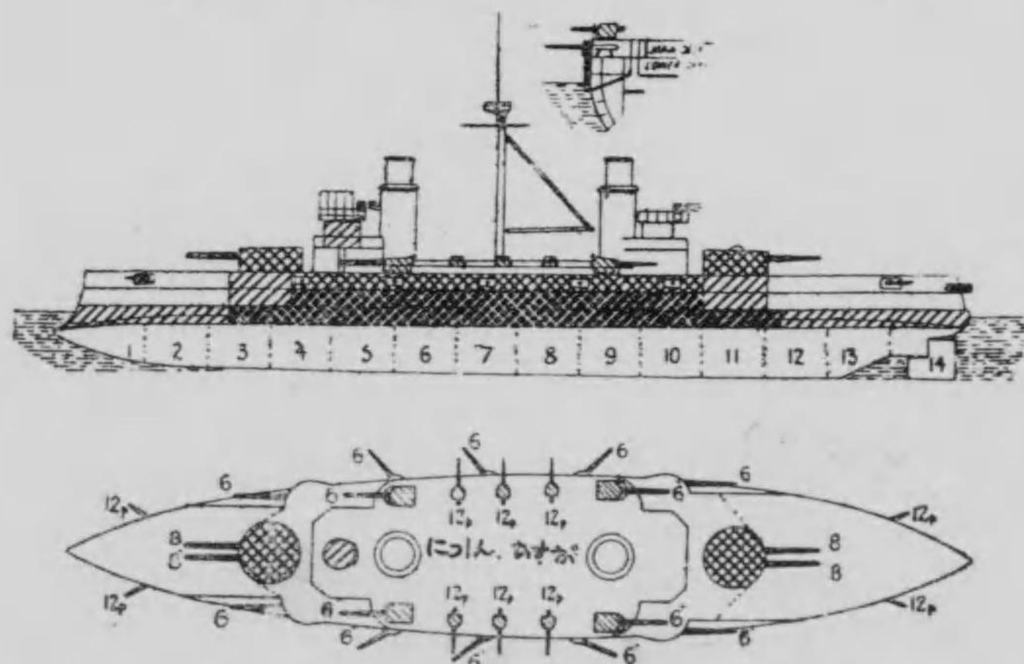
日進、春日 平面及側面圖 艦長三五七呎 艦幅六一呎 吃水二五呎
