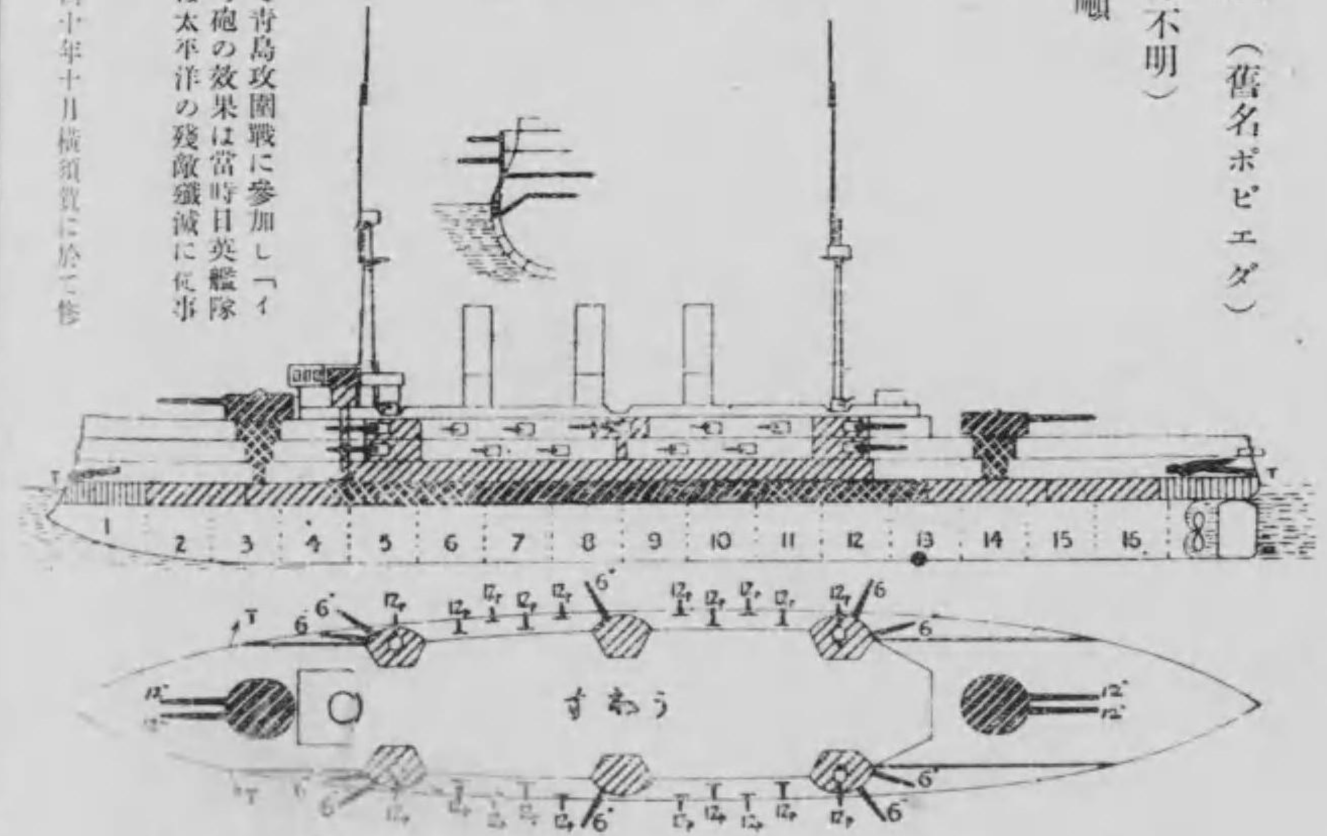
周防 水面及側面圖 長艦 四三二呎 幅艦 一七呎 吃水 二七呎
