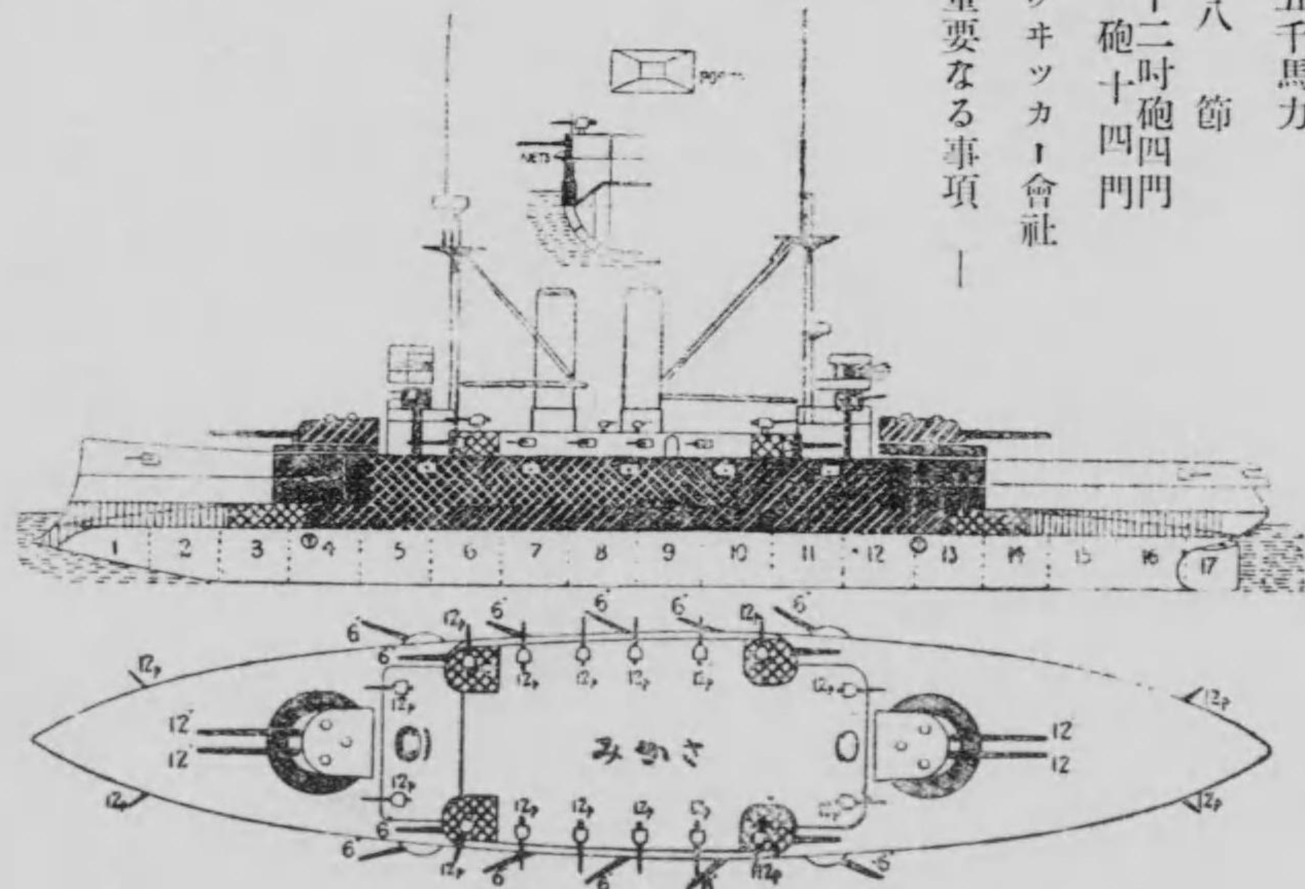
戦艦三笠 平面及側面圖 艦長四二四 幅艦一七一 吃水二七呎
