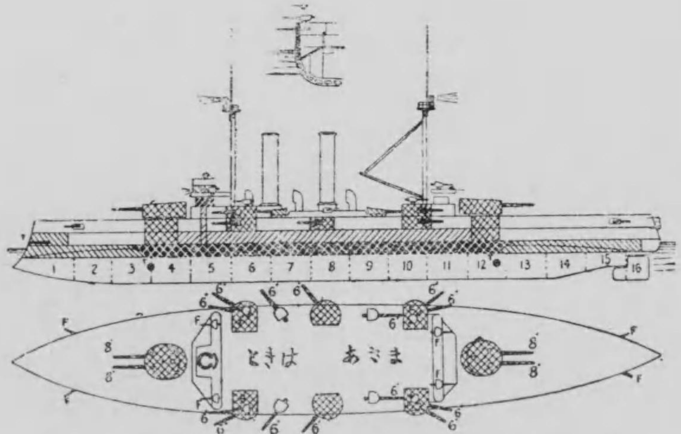
吃水四二呎 艦幅六七呎 艦長八〇呎 平面及側面圖 常磐 淺間
