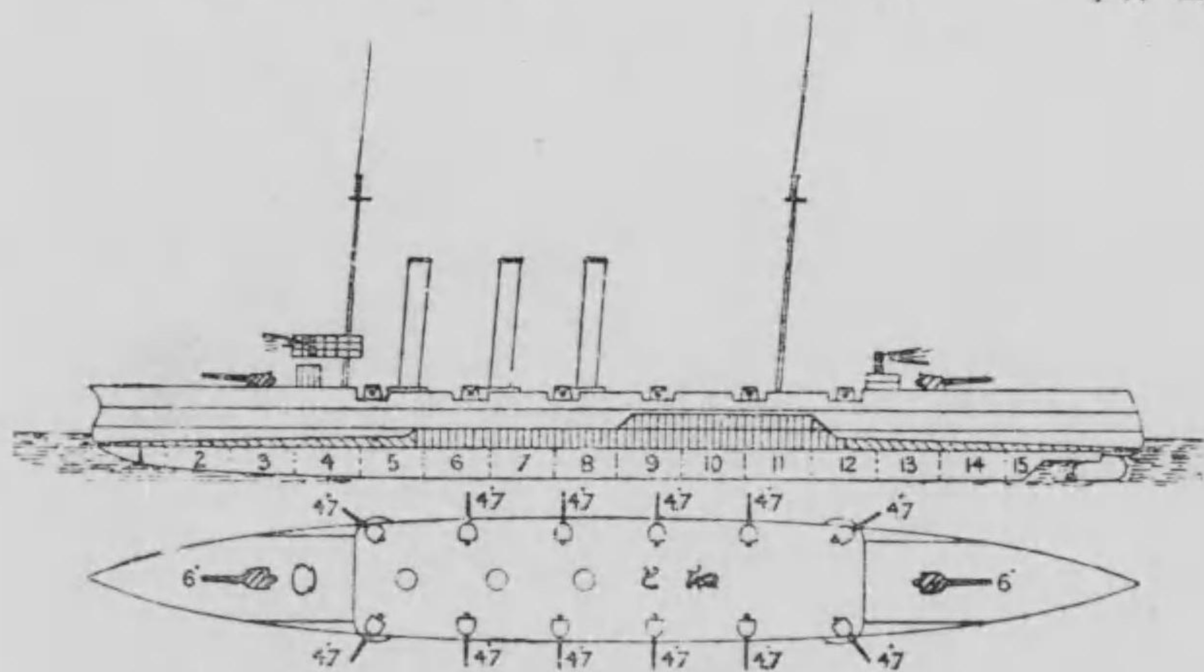
利根 平面及側面圖 長一四〇呎 幅四九呎 吃水七一呎
