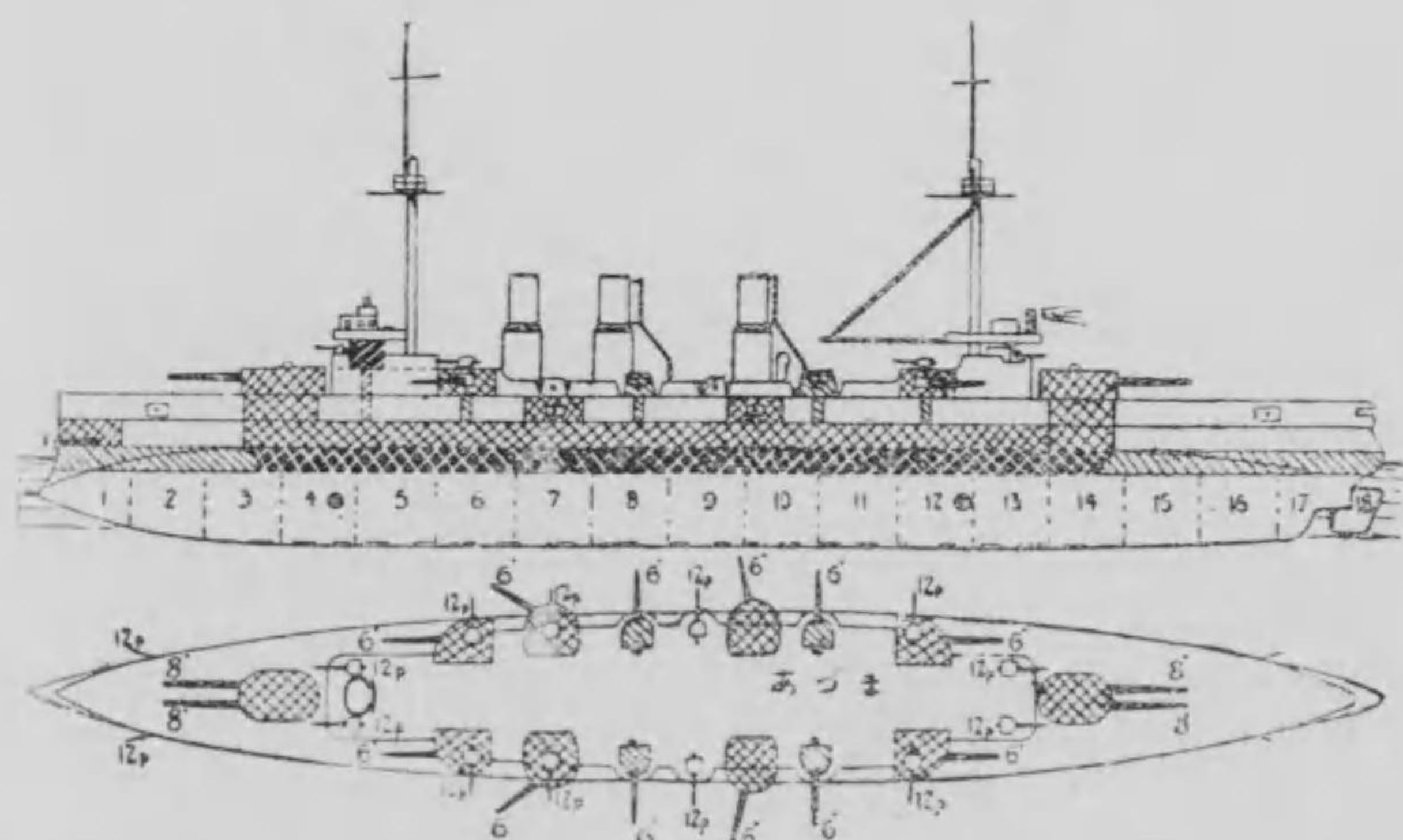
吾妻 平面及側面圖 艦長三四三呎 艦幅九五呎 吃水五二呎
