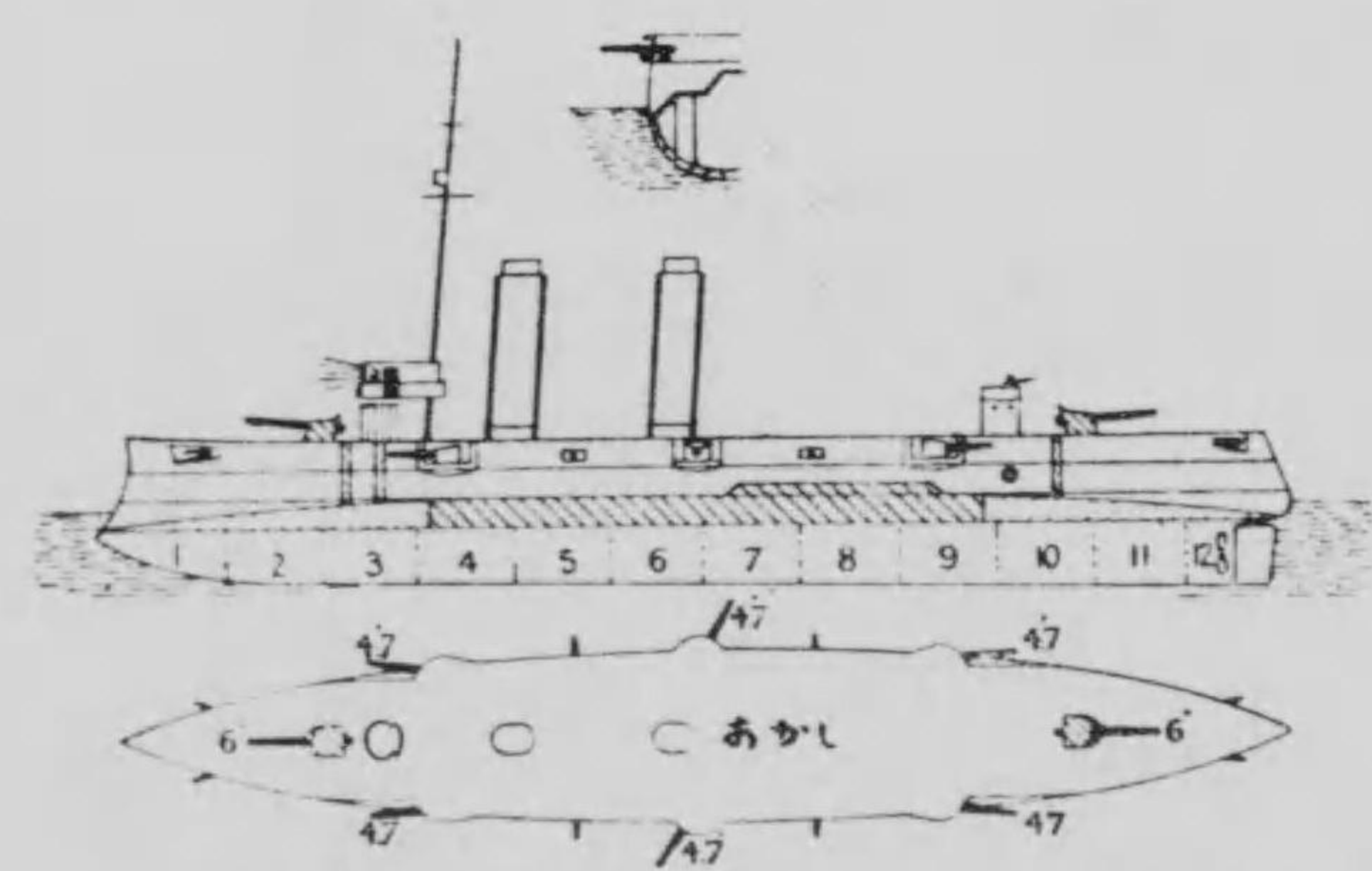
明石 平面及側面圖 艦長五〇呎 幅四一呎 吃水六呎
