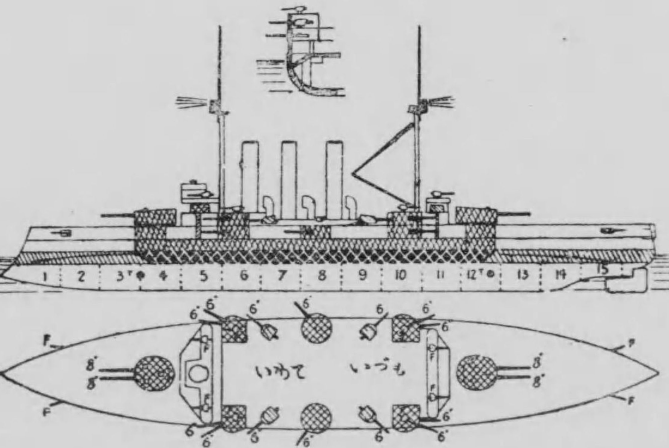
出雲、手磐 圖面側及面平 砲長四〇〇 艦幅六八吋 吃水二四呎
