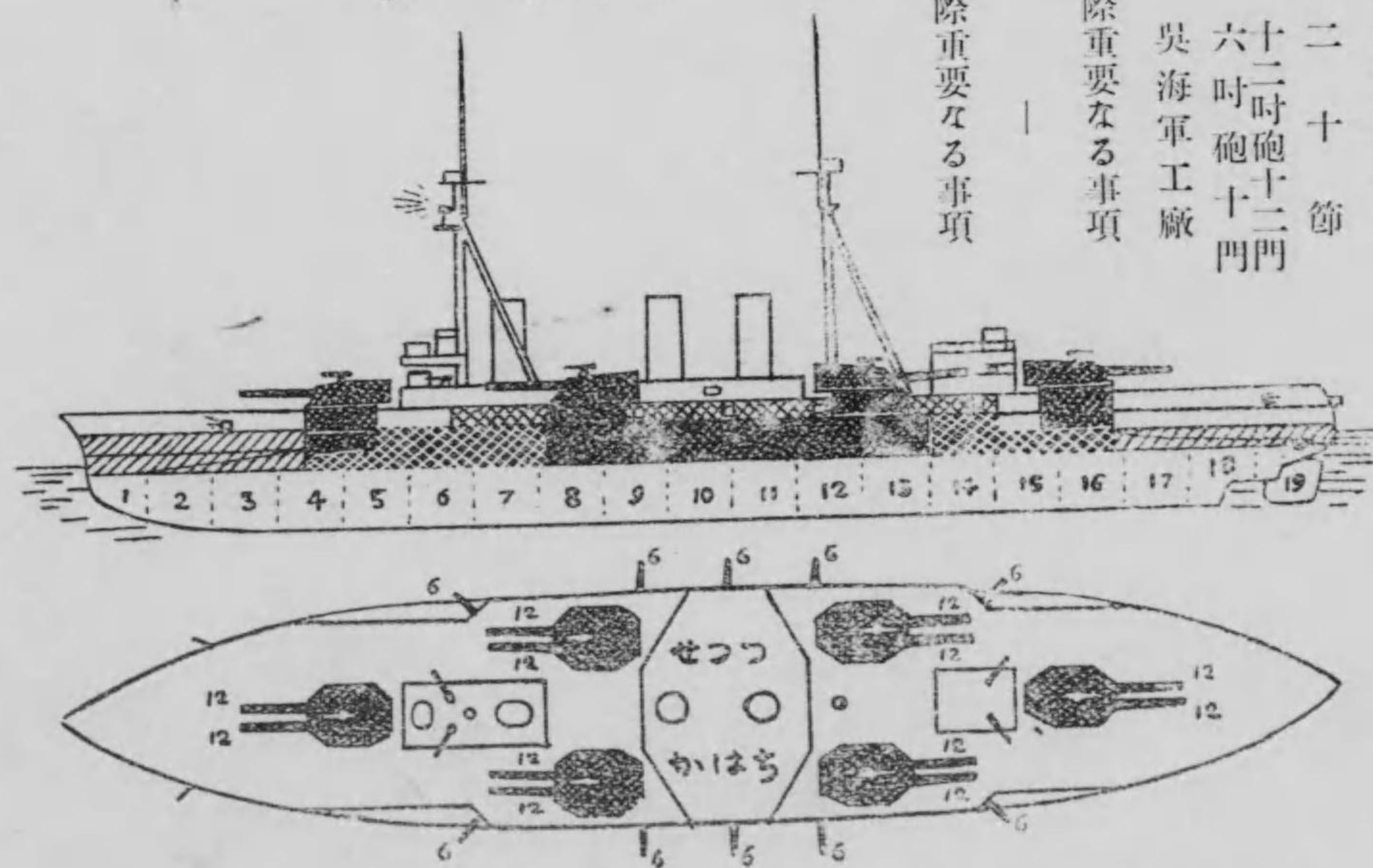
戦艦 攝津、内河、平面及側面圖 長艦 五〇〇 幅艦 八四 吃水 二八
