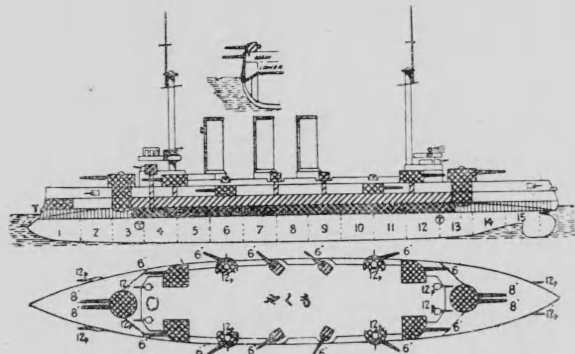
八雲 平面及側面圖 艦長三〇九呎 艦幅五六呎 吃水三三呎
