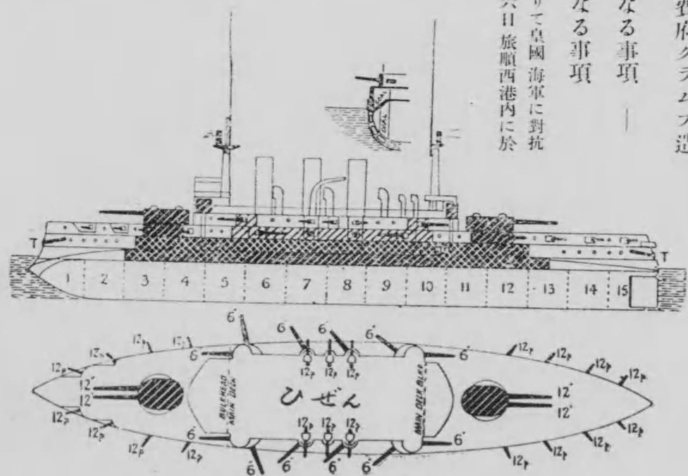
肥前艦面平及側面圖 艦長三十七呎 艦幅七呎六寸 吃水二呎六寸
