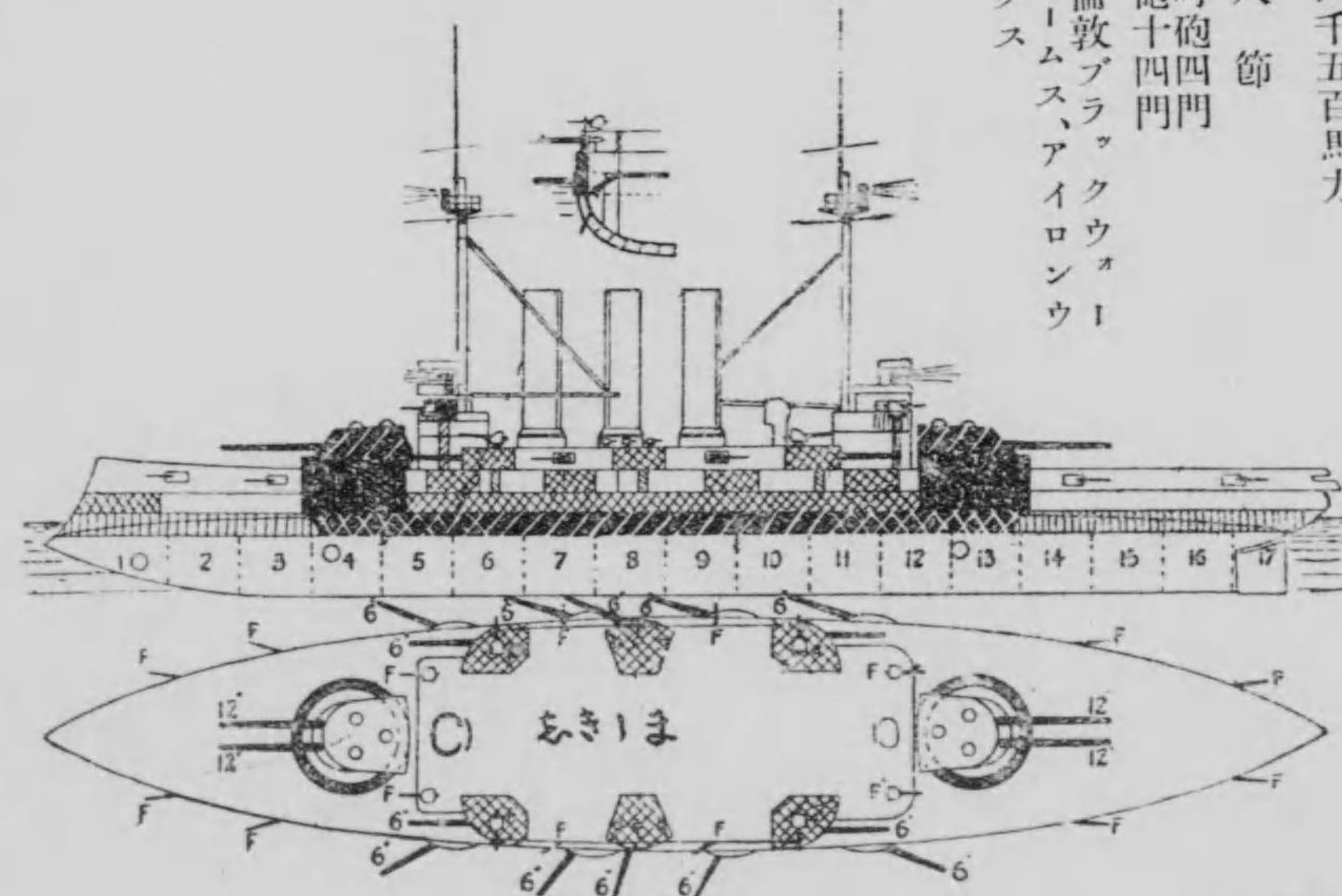
戰艦敷島 水面及砲面圖 長鑿 四一五呎 鑿幅 七六呎 吃水 二八呎
