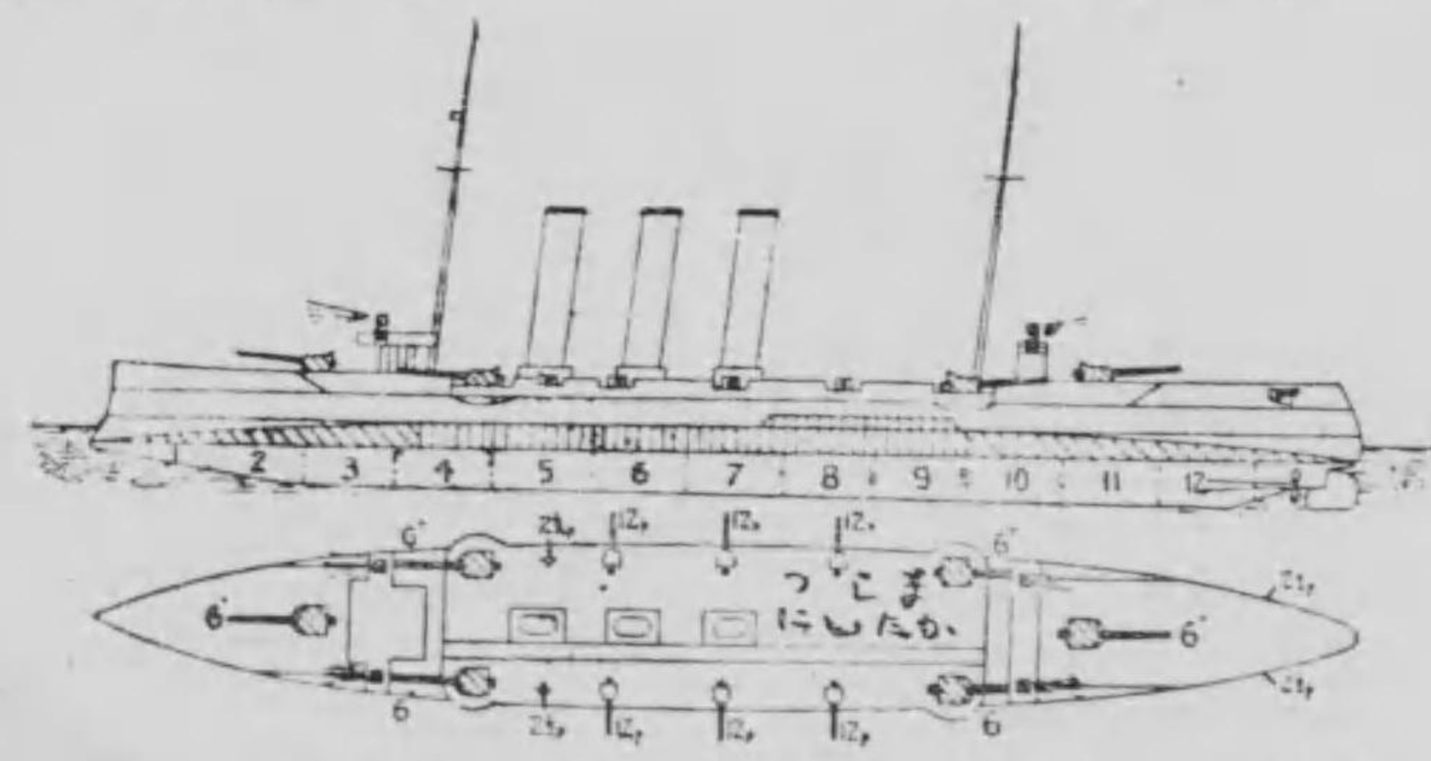
對島、新高 平面及側面圖 艦長三三尺四 艦幅四四尺 吃水六一尺
