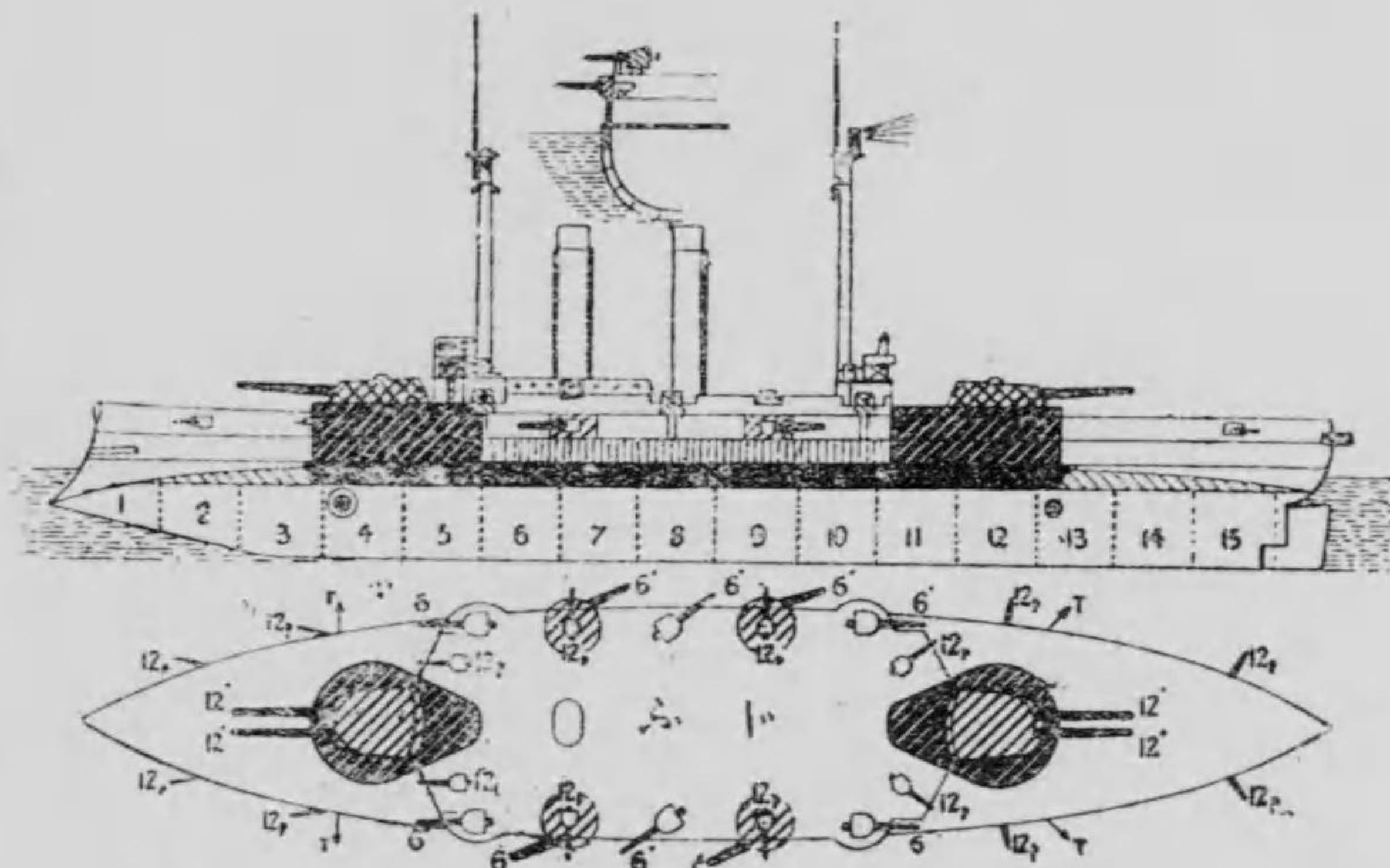
富士 水面及側面圖 長艦 三九〇呎 幅艦 三七呎 吃水 二九呎
