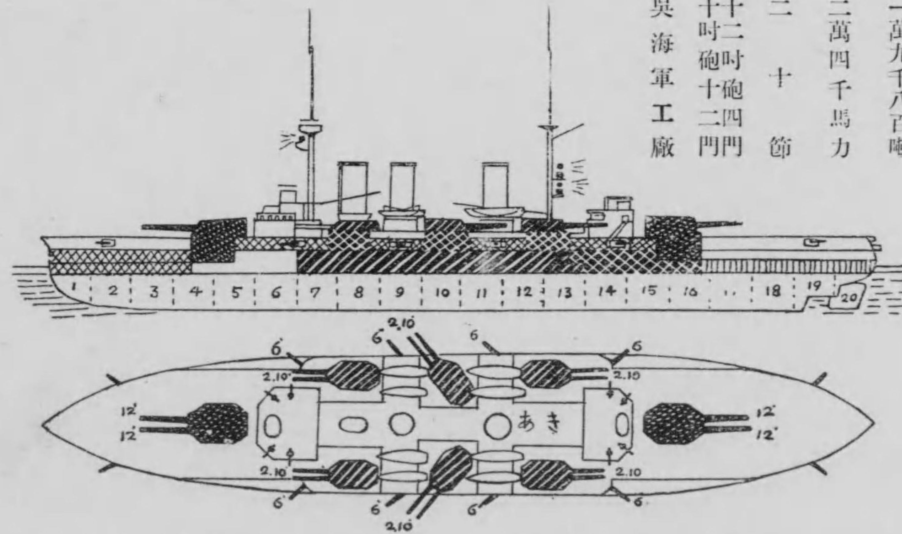
戰艦安藝 平面及側面圖 艦長四九二呎 艦幅三八呎 吃水二七呎
