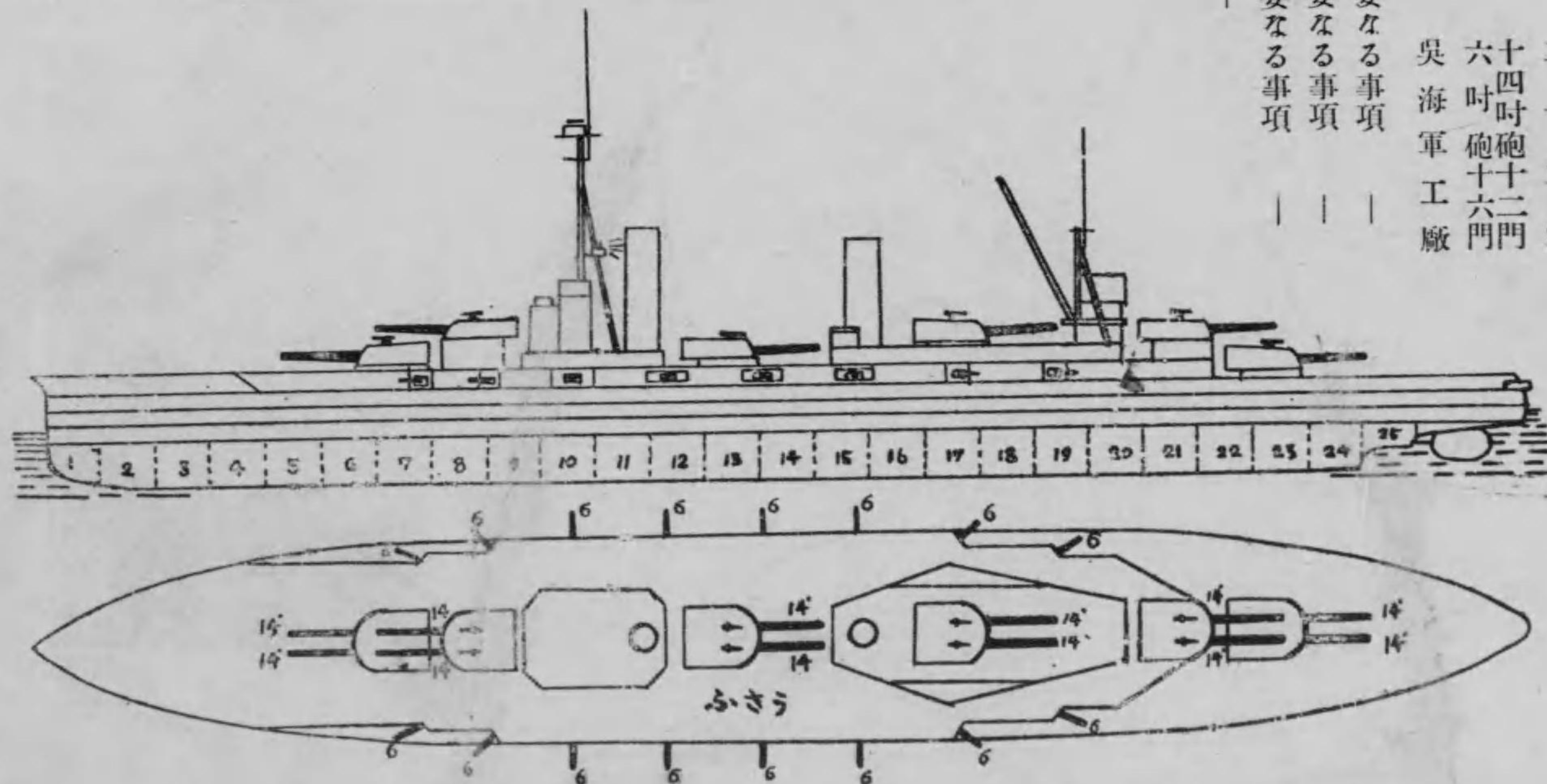
戰艦扶桑平面及側面圖 長艦 三七六呎 幅艦 四九呎 吃水 二八呎
