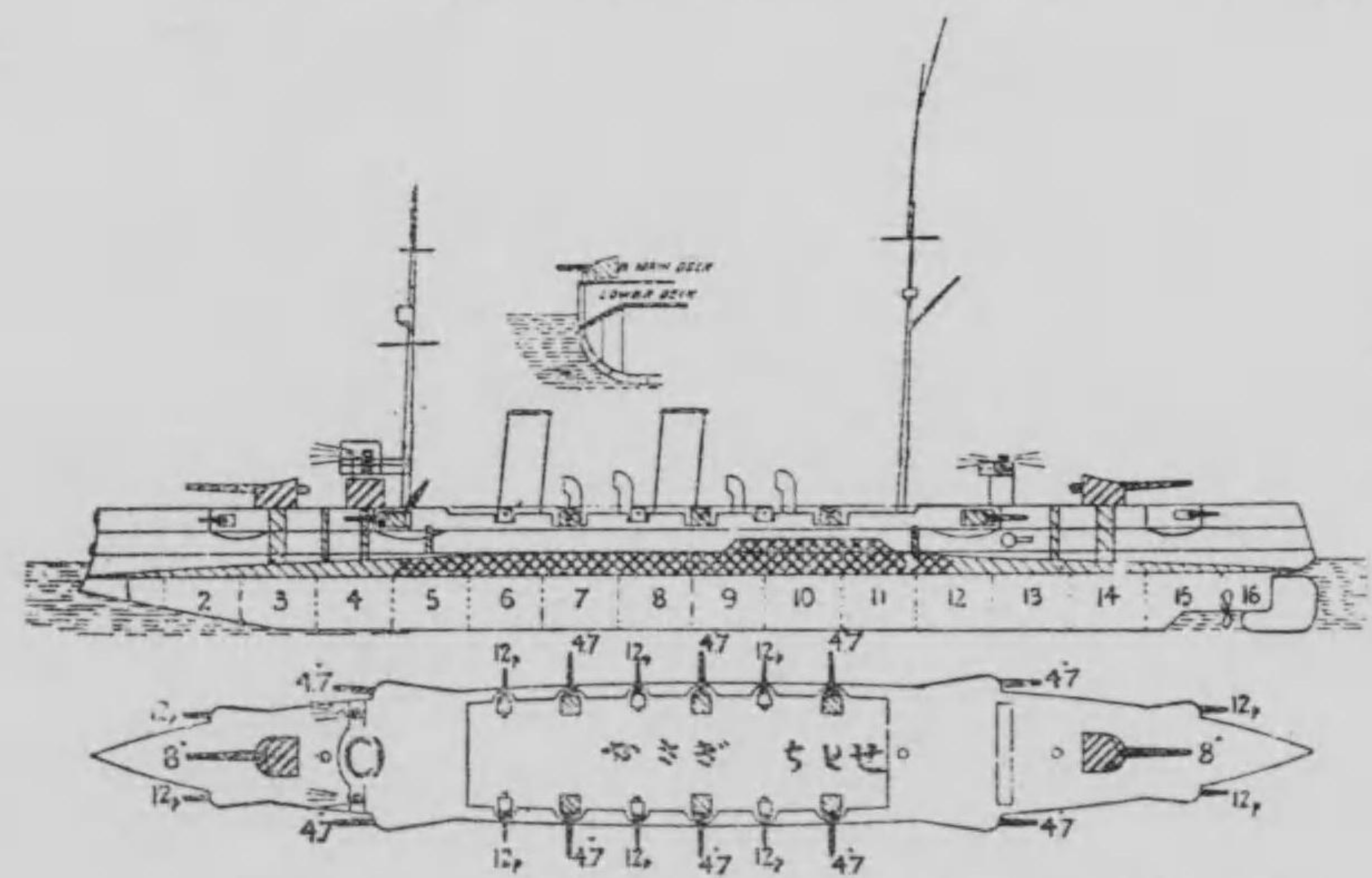
笠置、千歳 平面及側面圖 艦長三九六呎 艦幅四八呎 吃水四二呎
