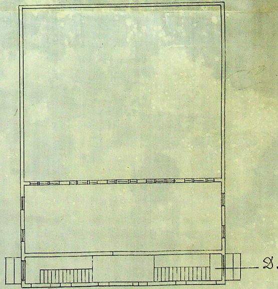
Планъ второго внутренняго этажа.
