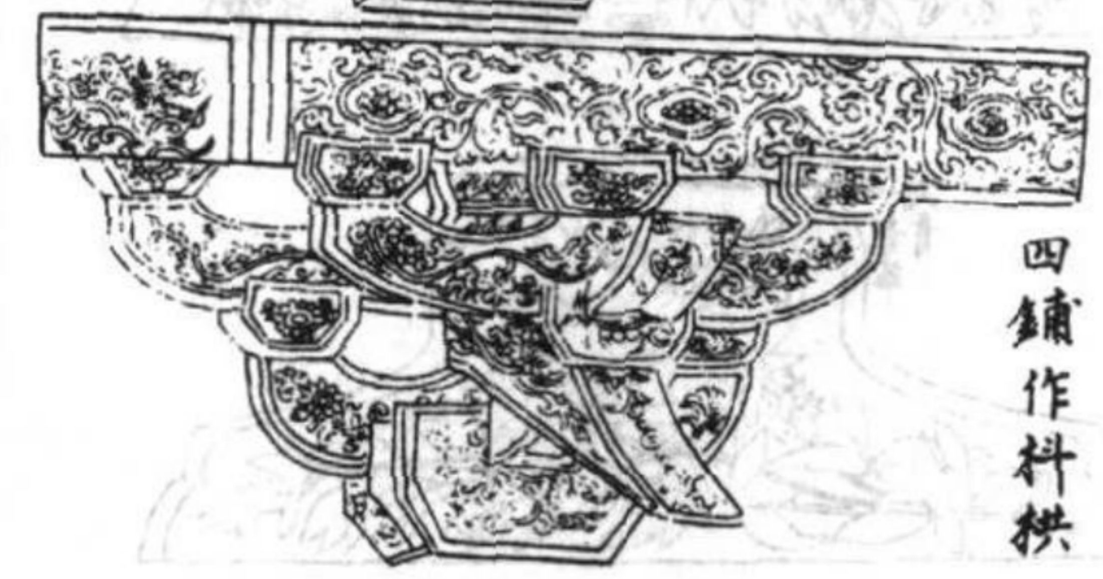
五鋪作料拱
