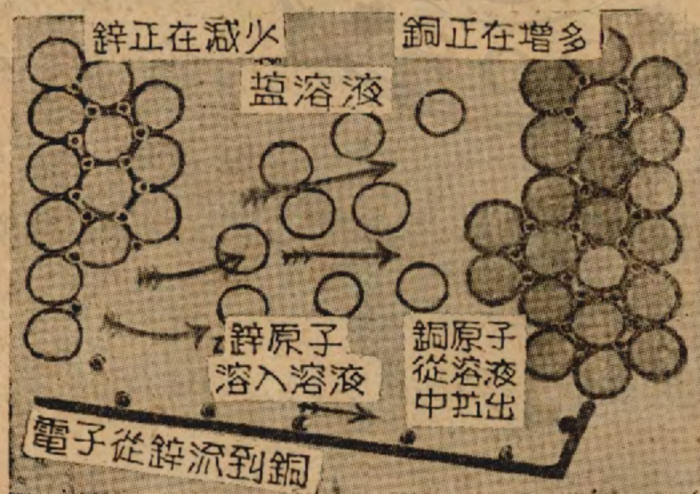
圖九 (2) 電子正在從鋅版流到銅版，使溶液中的原子能夠積集于銅版上，而一方面把鋅版蝕掉。
