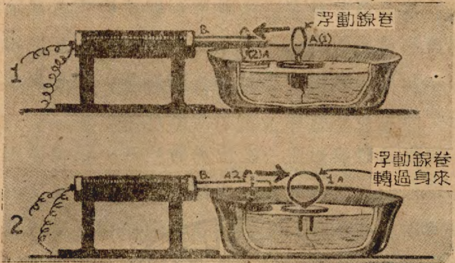
圖五 在一個線卷的磁場和一根固定磁鐵間之力。 (1)浮動線卷“A”會自己飄過去套在磁鐵B上。 (2)把固定線卷中的電流反向時,浮動線卷會飄開,翻一轉身,又飄回去套在磁鐵上。
