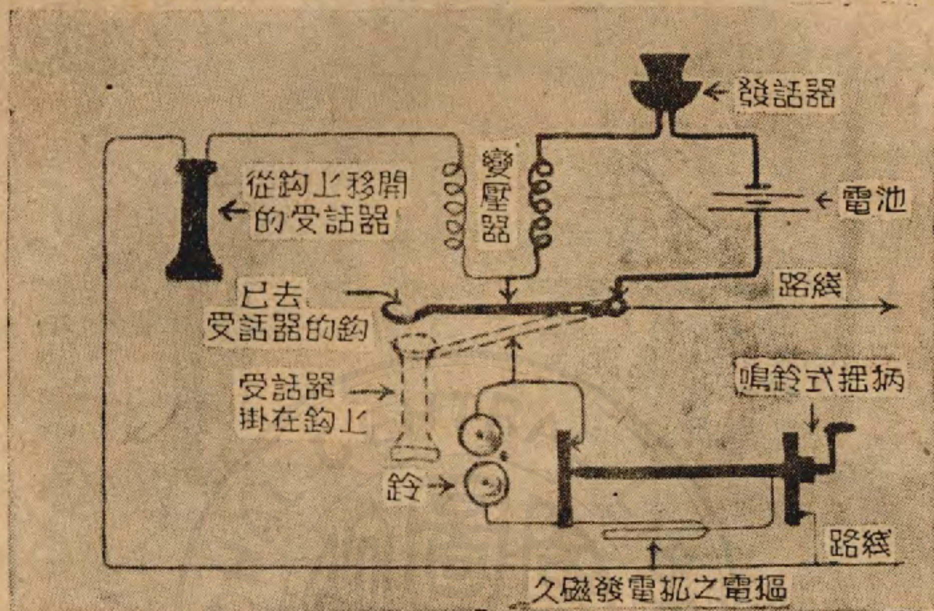
圖六 上圖表示倘使我們把受話器從鉤上移開, 為什麼我們的鈴就不會振響。倘使那受話器是掛在鉤上, 綫路和我們的鈴即接通, 把它移開時, 綫路即與發話器和受話器接通了。
