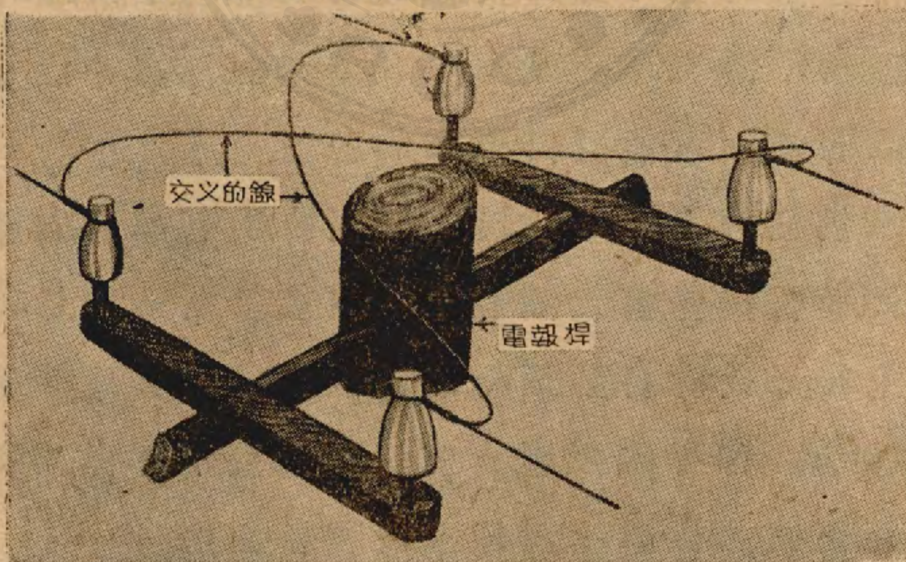
圖七 保證電話不漏聽的裝置法; 交叉的線設在細心計算出之點。
