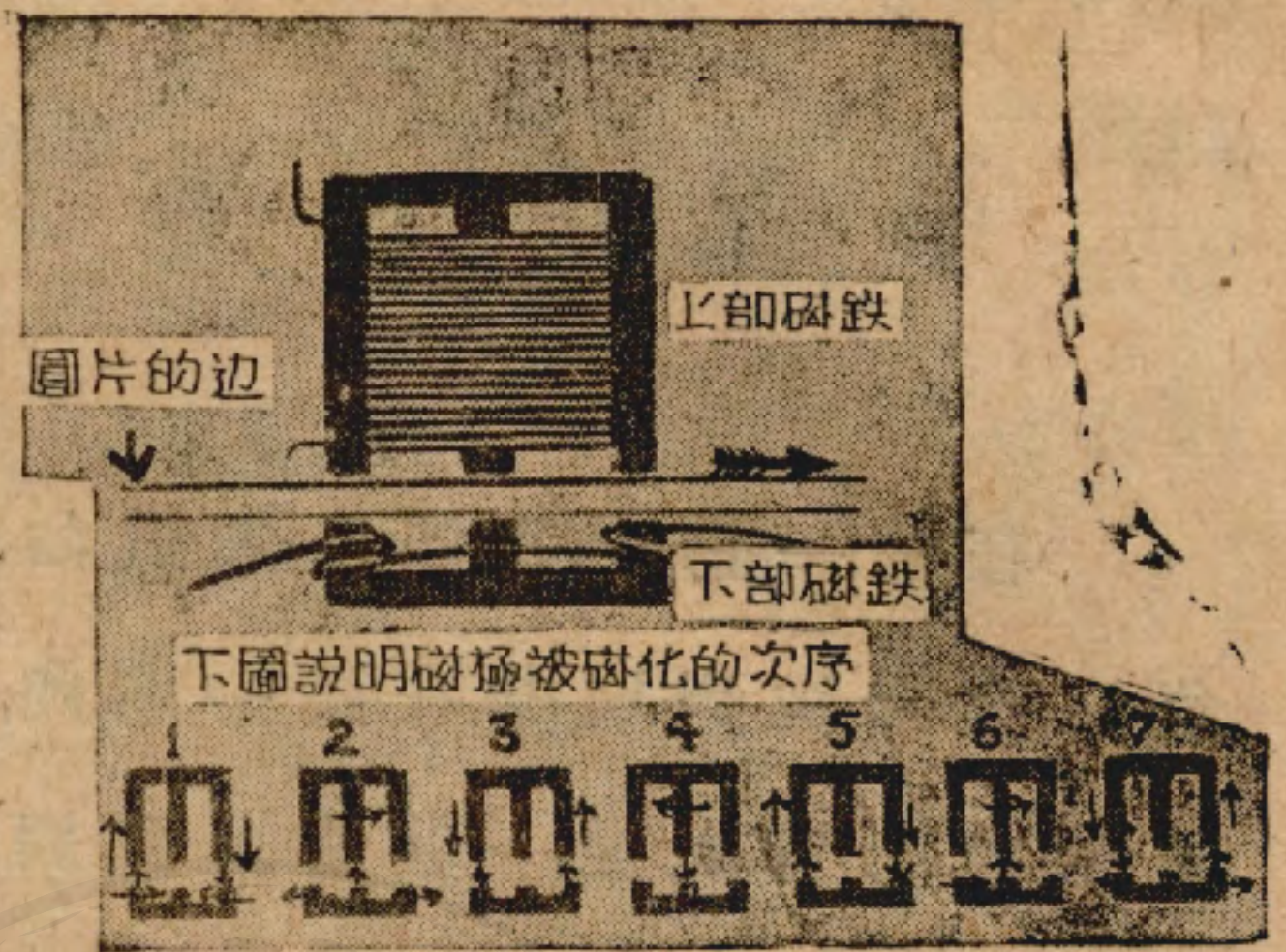
圖十二 磁鐵如何轉動這金屬圓片： 上部磁鐵的線卷有較多匝的線，故比下部磁鐵被磁化得慢些。因此發生一種作用，好像這磁鐵在不斷地從左向右移動。
