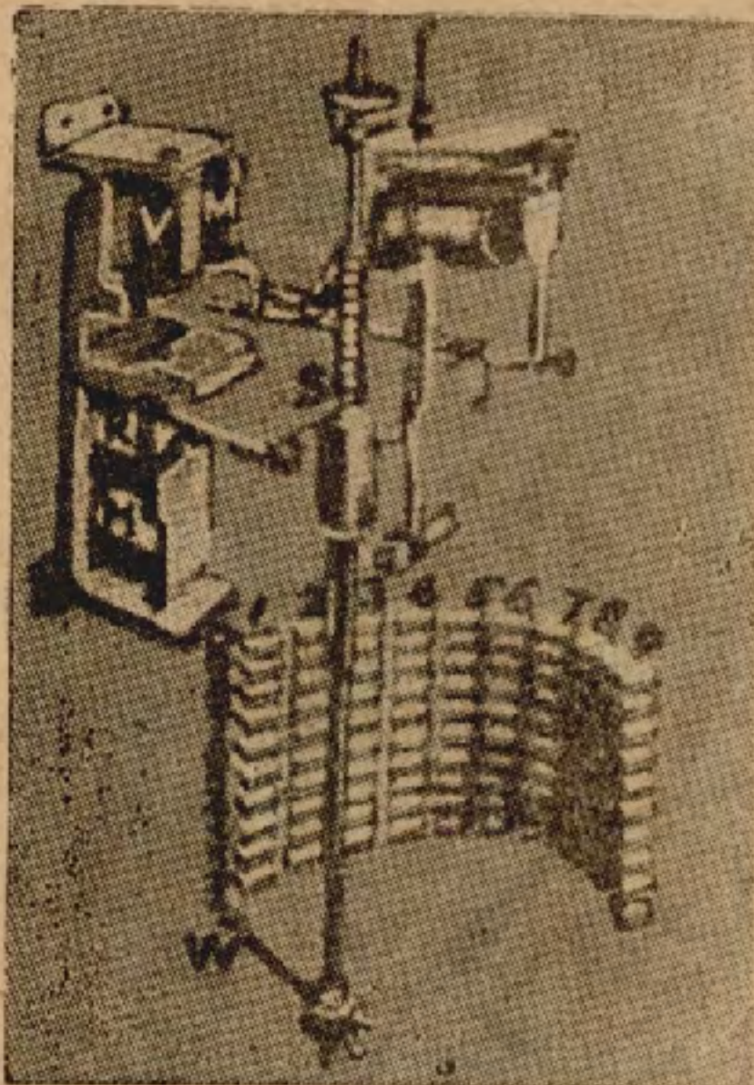
圖九 自動電話交換機中的奇器。
