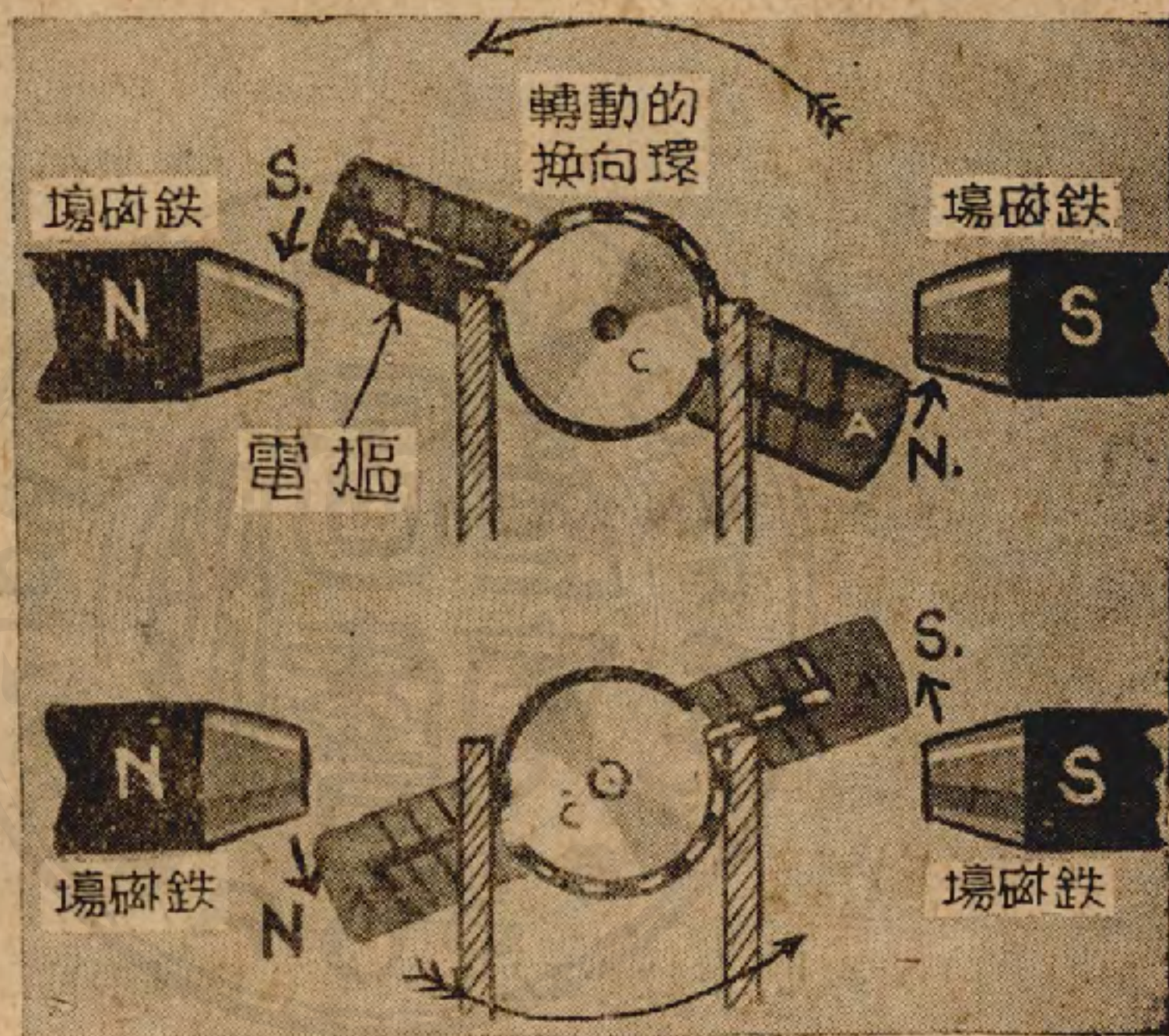
圖八 電動機的原理
