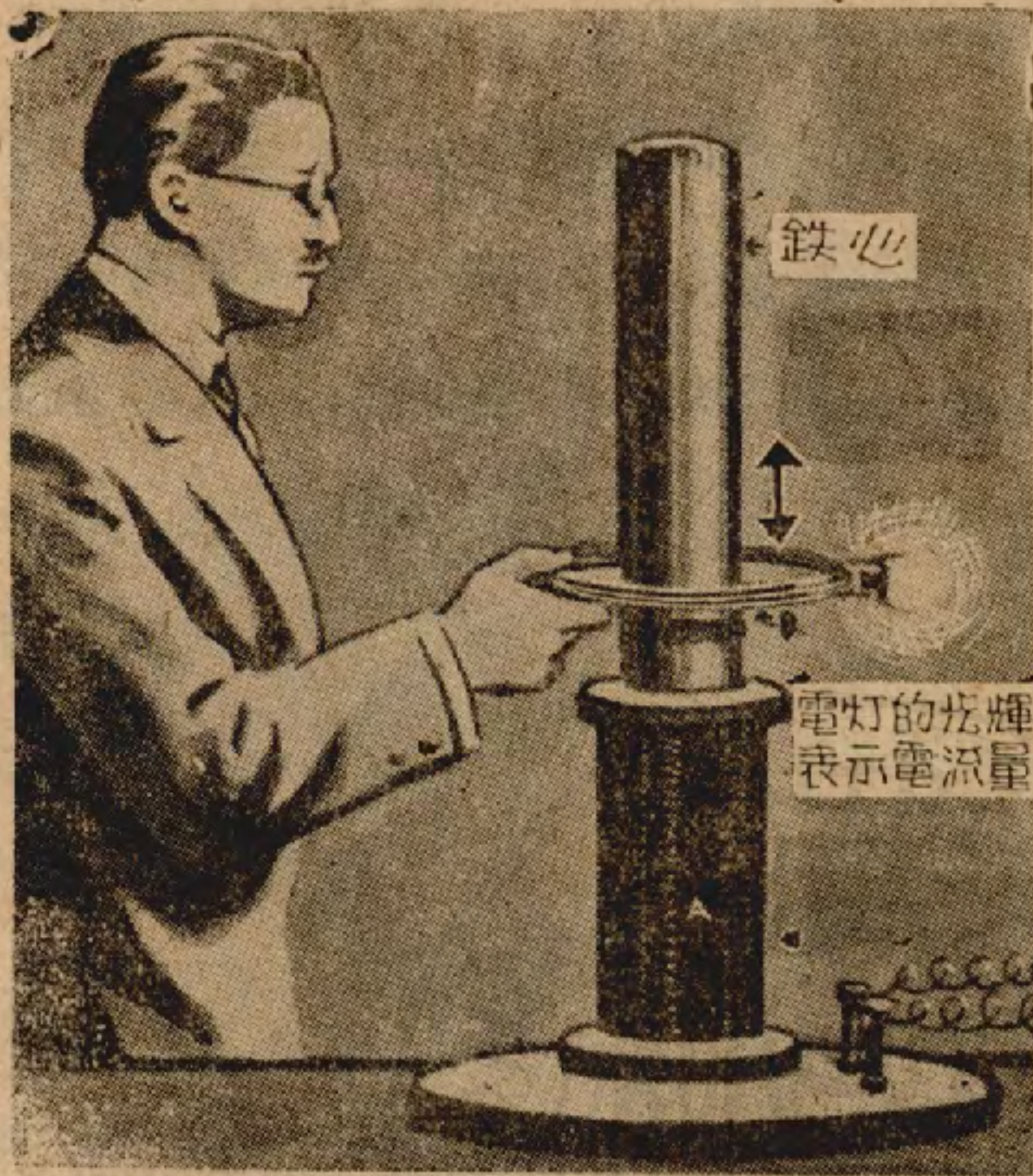
圖六 變壓器的原理（該器只能應用於交流電）。把交流饋入線卷“A”，線卷“B”中即感生交流。
