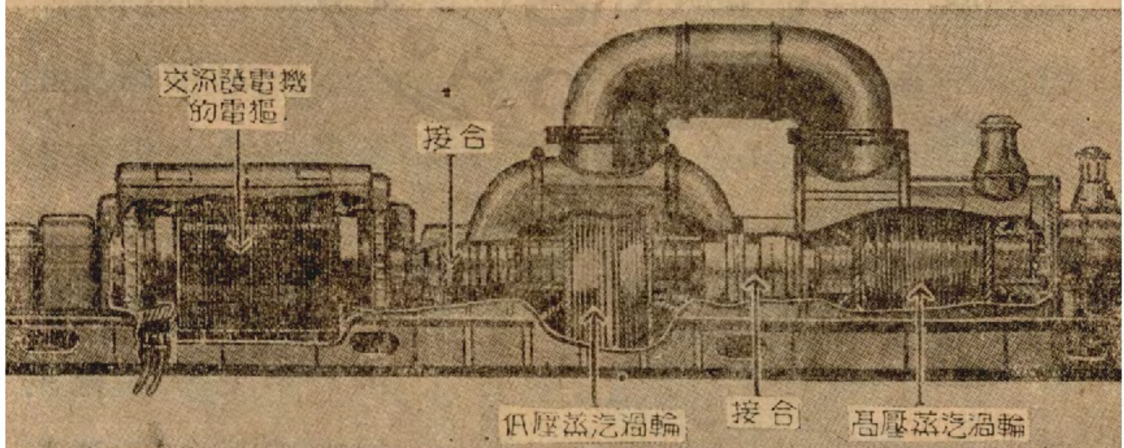
圖一 靠蒸汽渦輪來轉動的發電機：法國郵船『諾曼地』號所裝的一座龐大的33,400 仟瓦特汽渦輪傳動交流發電機。從船上汽鍋中出來的蒸汽先入高壓渦輪，再入低壓渦輪。它們與交流發電機直接相連，轉動其電樞而發電，用以動四隻電動機，每只電動機傳動一只推進器。
