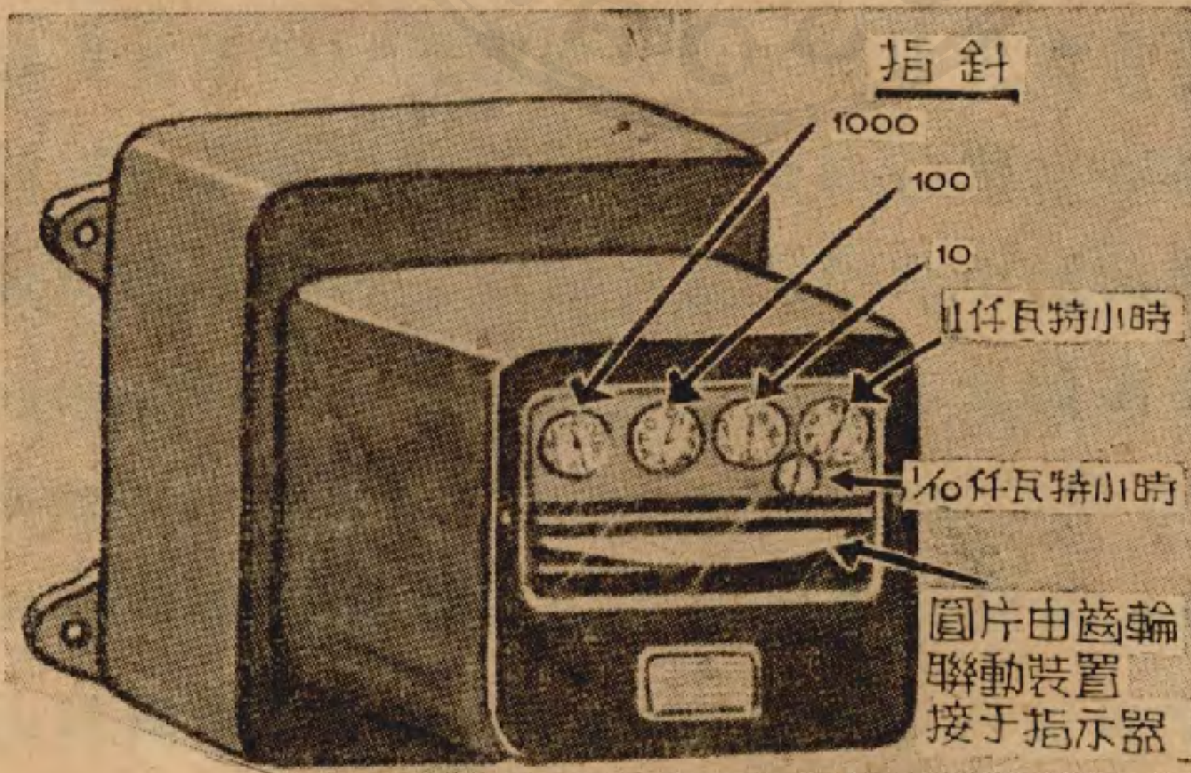
圖八 家用電能計,開燈愈多,圓片轉動愈快。
