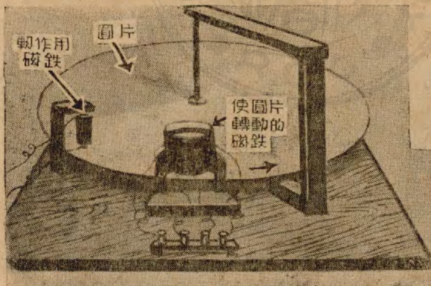
圖十一 我們應用此種渦流的粘滯拉力來運用我們的電能計(瓦特小時計),藉以量出所用去的電能量。上圖是一具瓦特小時計中轉動圓片的簡單模型。
