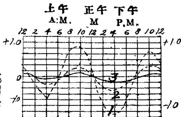
氣壓之日變化
