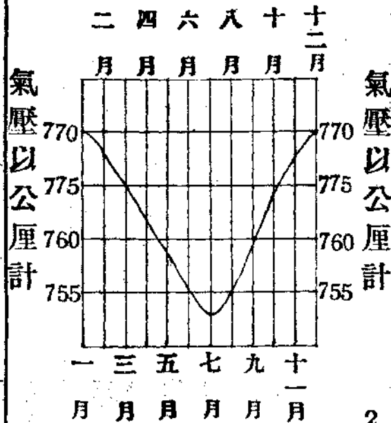
第六圖 氣壓之年變化
