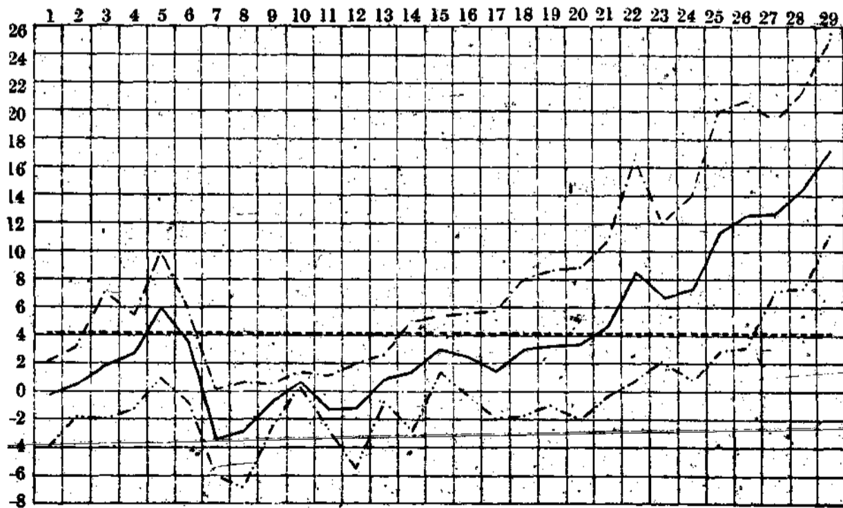
中華民國十七年二月份氣溫變遷圖 (°C) The March of Temperature in the Month of February, 1928 (°C)
