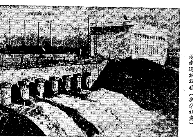
越南民主共和国最大的水电站——清化省的班合水电站，今年元月就已落成，开始发电。它的发电能力为一千零八十瓩，可以满足全省工业区的用电，有了这个水电站，附近几个县的农田也得到灌溉。
