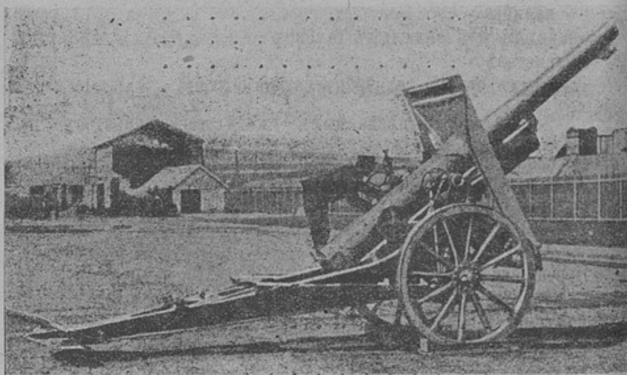
Фиг. 2. 15 см. (6 дм.) осадная пушка.
