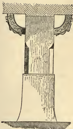
FIG. 44.—BRACKET CAPITAL.
