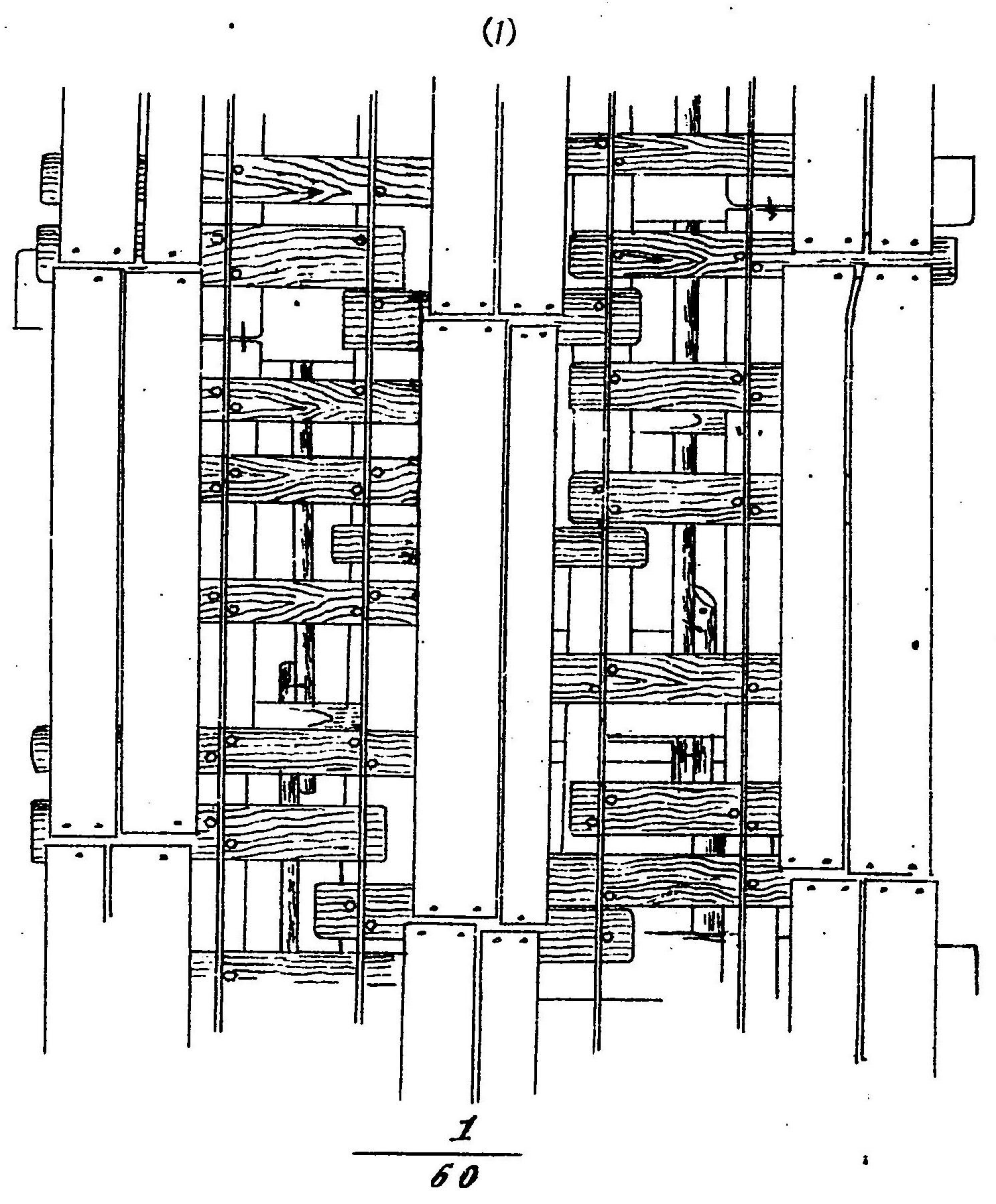
東清鐵道ニ於ケル橋梁
