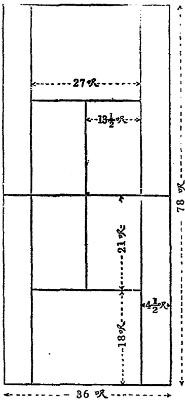
場球網 (22)圖
