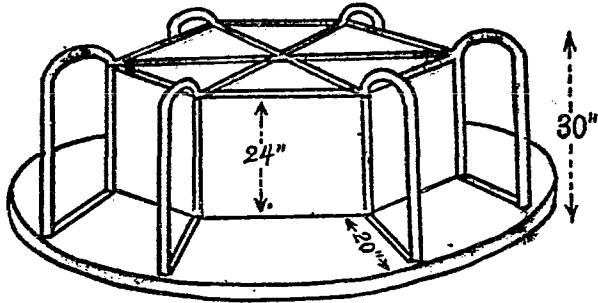
圖約寸尺槓轉(43)圖
