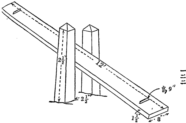
圖 33 軒輕板
