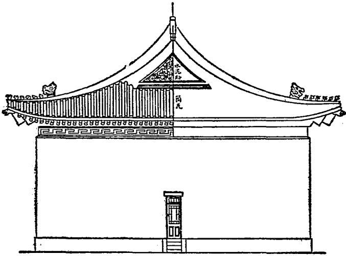
圖面側院平和(9)圖
