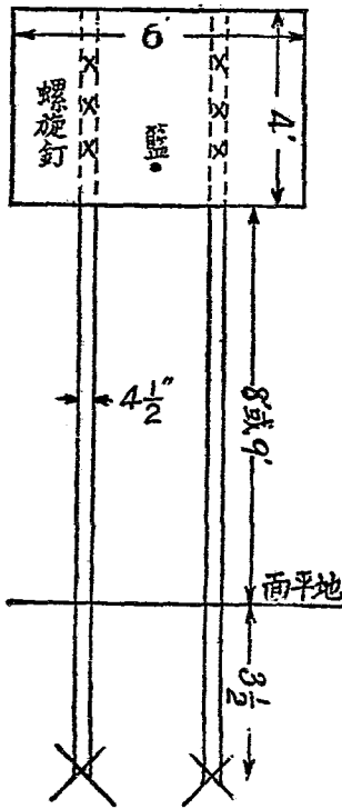
圖面正架球籃 (17) 圖
