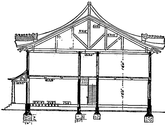
圖面剖院平和(10)圖
