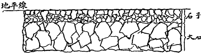
(23) 圖 碎石路剖面
