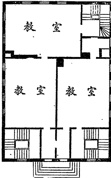
圖(2) 阿拉白馬學校校舍
