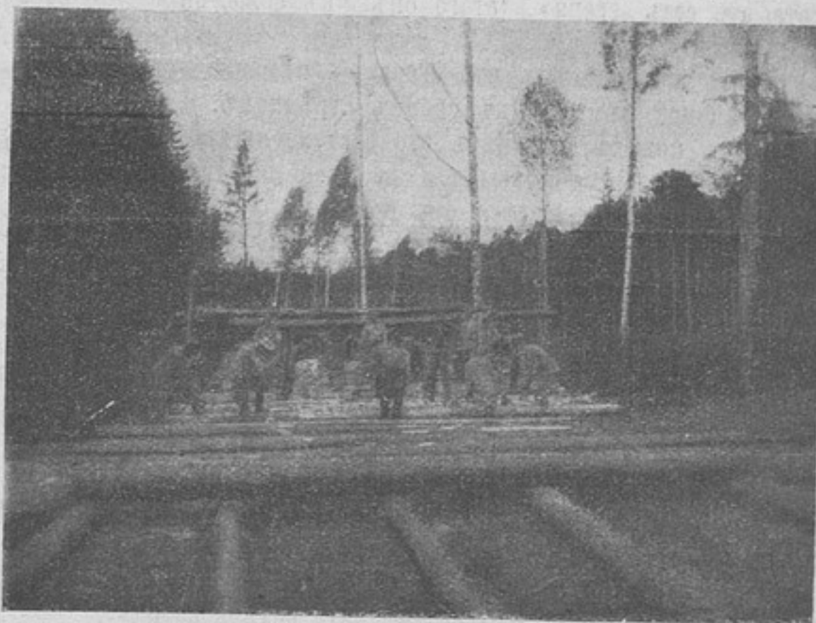
Устройство дороги съ бревенчатымъ настиломъ.
