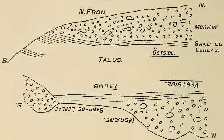
Fig. 3. Profil fra Kampesæter. N. Fron.
