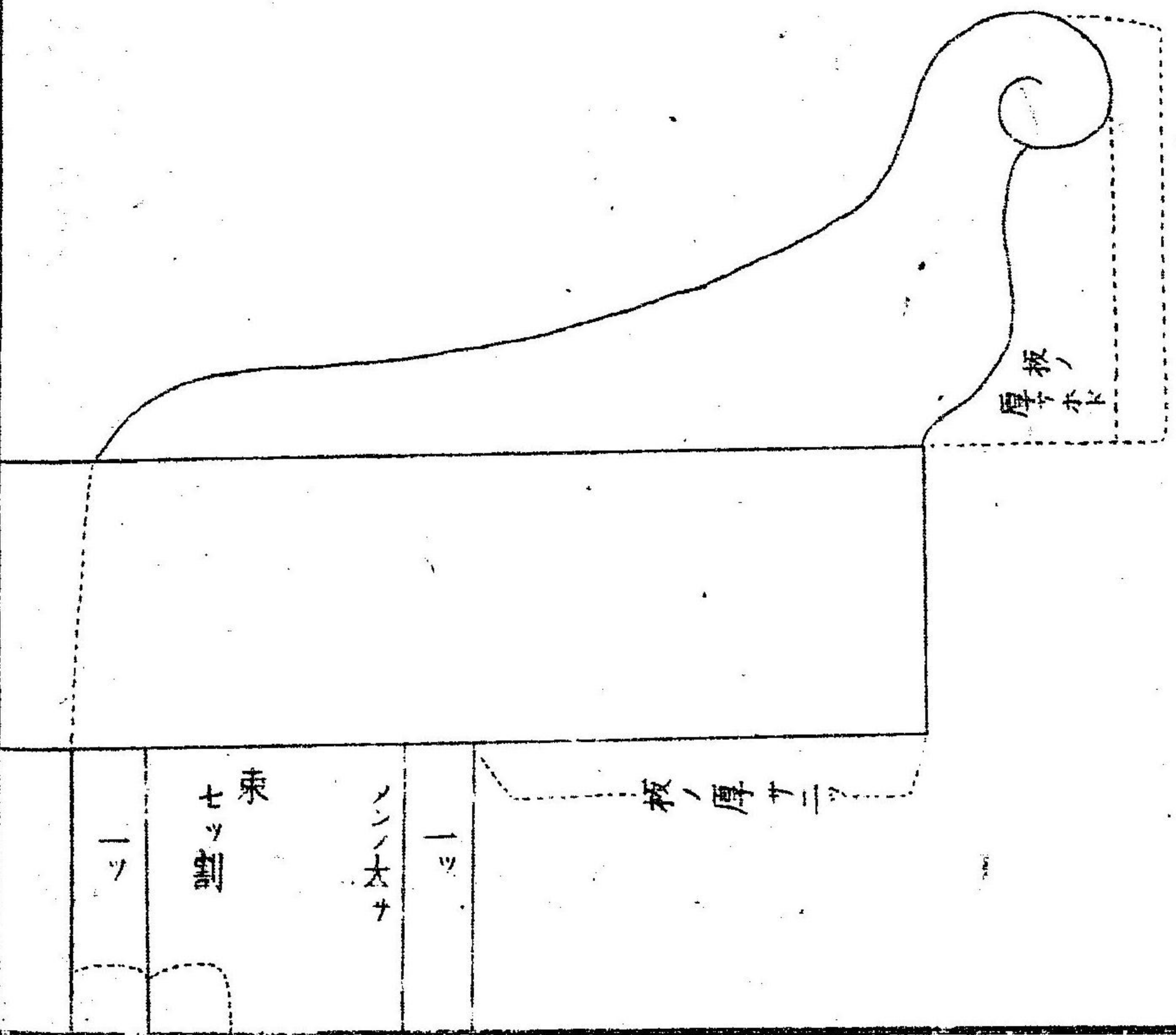
タナ板厚一ツ半
