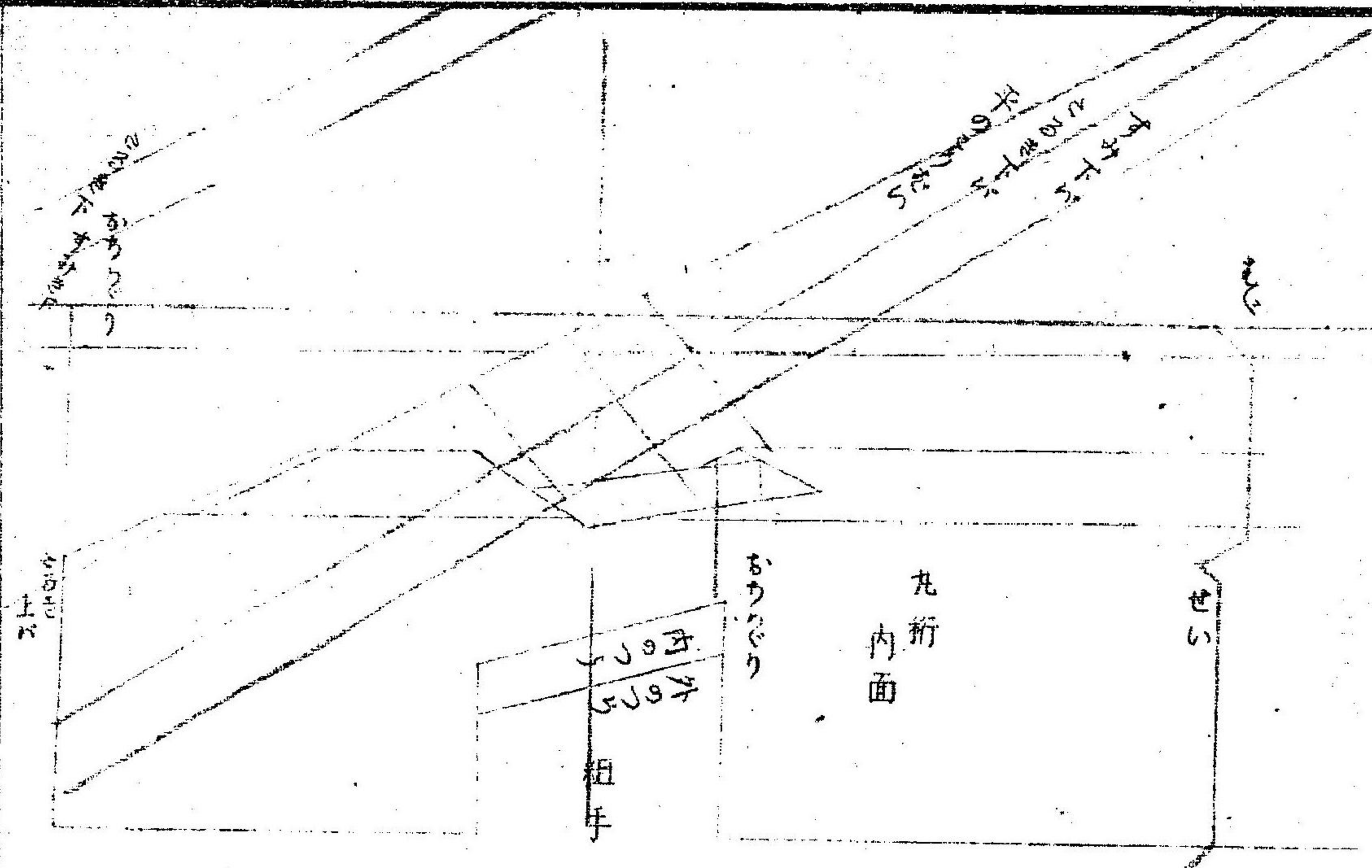
九折組手内面之圖
