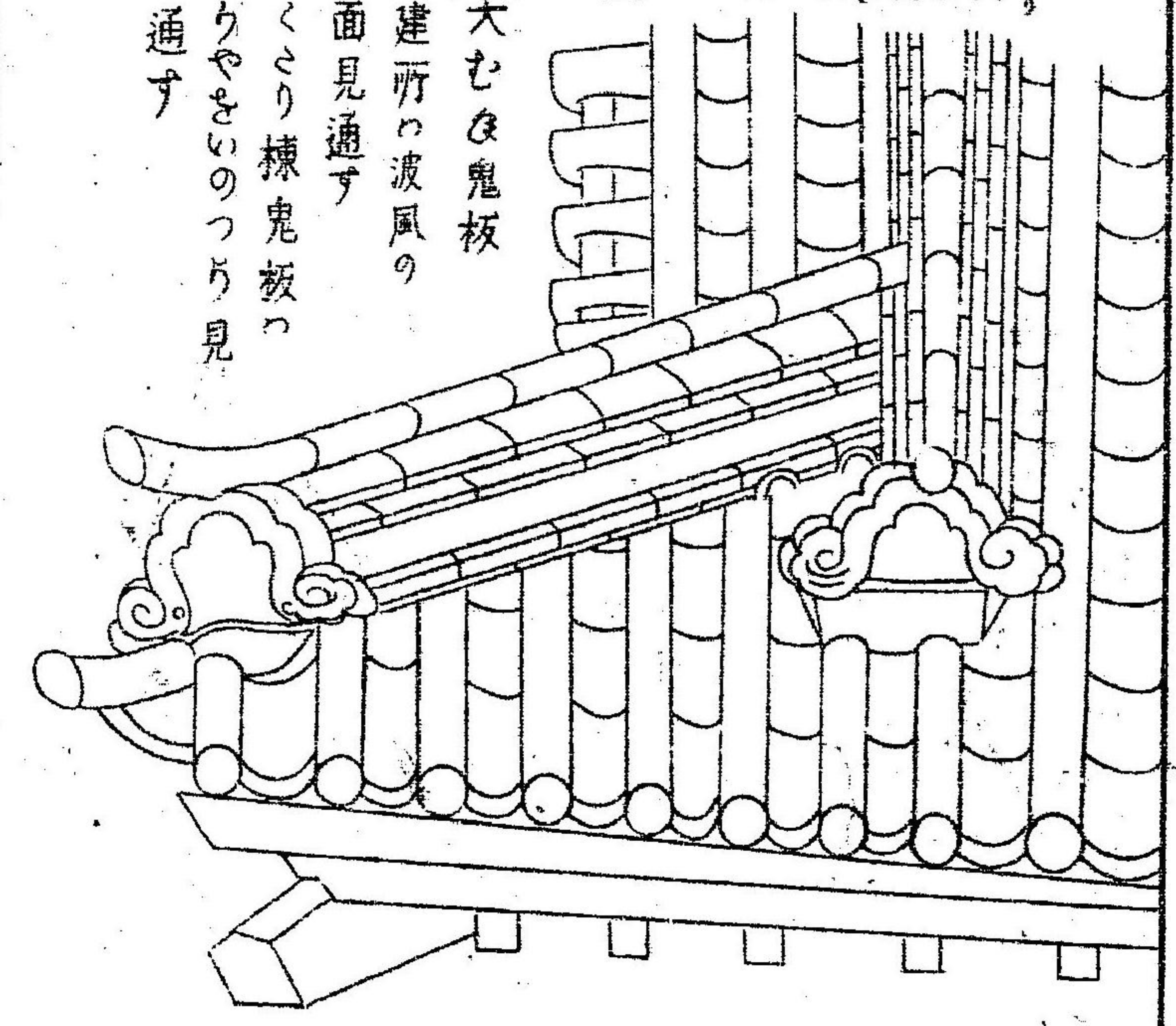
降棟軒端ノ図
