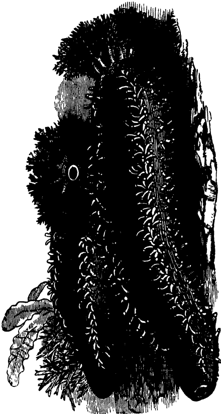
Fig 242.— Holothuridea , Sea-cucumbers.
