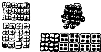
Fig. 153.— Sarcina ventriculi .
