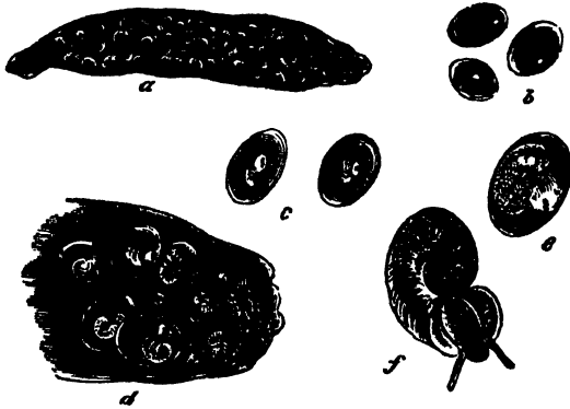
Fig. 252.— Limnæa stagnalis .
