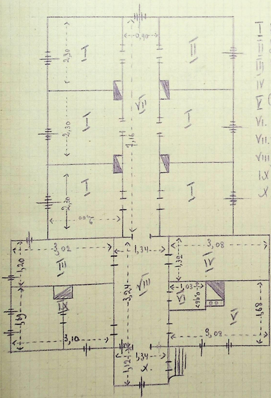
План школы №2 на ст. Квастив.
