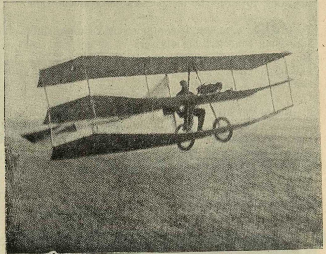
Трипланъ инженера Граде.
