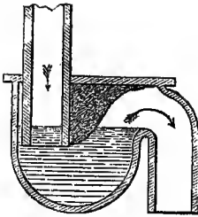
FIG. 5.—D-Trap.
