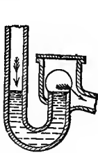
FIG. 142.—Buchan's Trap.
