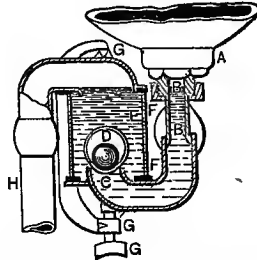
FIG. 147.—Bennor's Siphon Trap.
