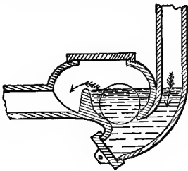
FIG. 140.—Cudell Trap.
