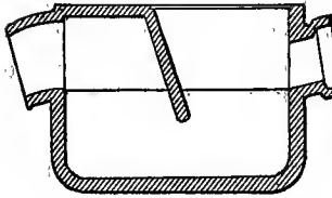
FIG. 56.—Bavin Trap.
