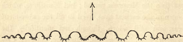
Ceratites nodosus.
