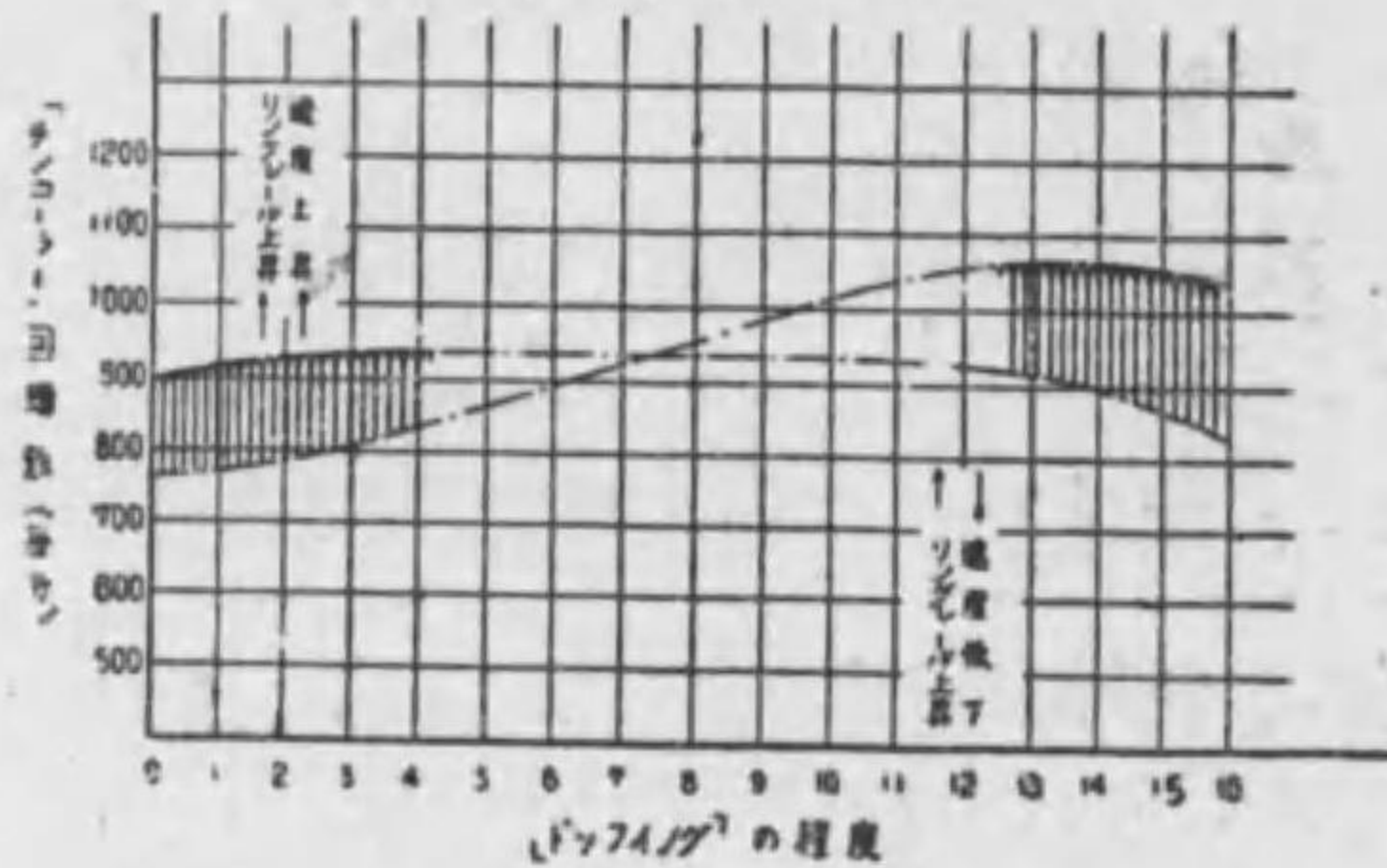
雙速度曲線
