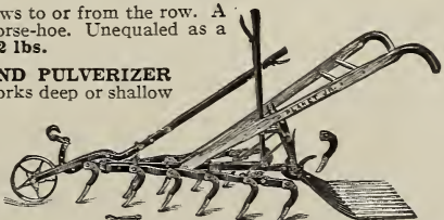
Planet Jr. 12-Tooth Harrow
