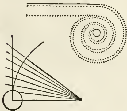
Ionicæ volutæ emendata circinatio.
