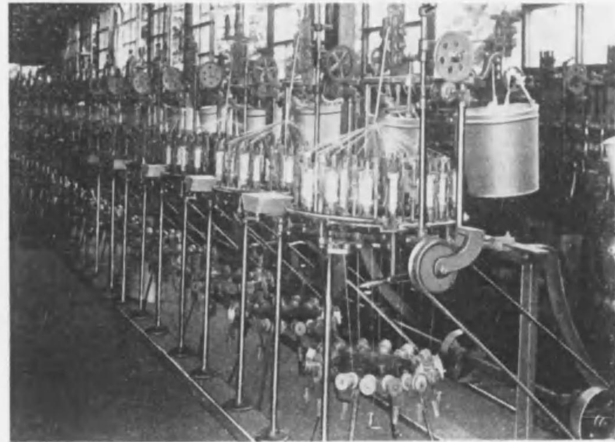
(組紐工場ノ一部)
