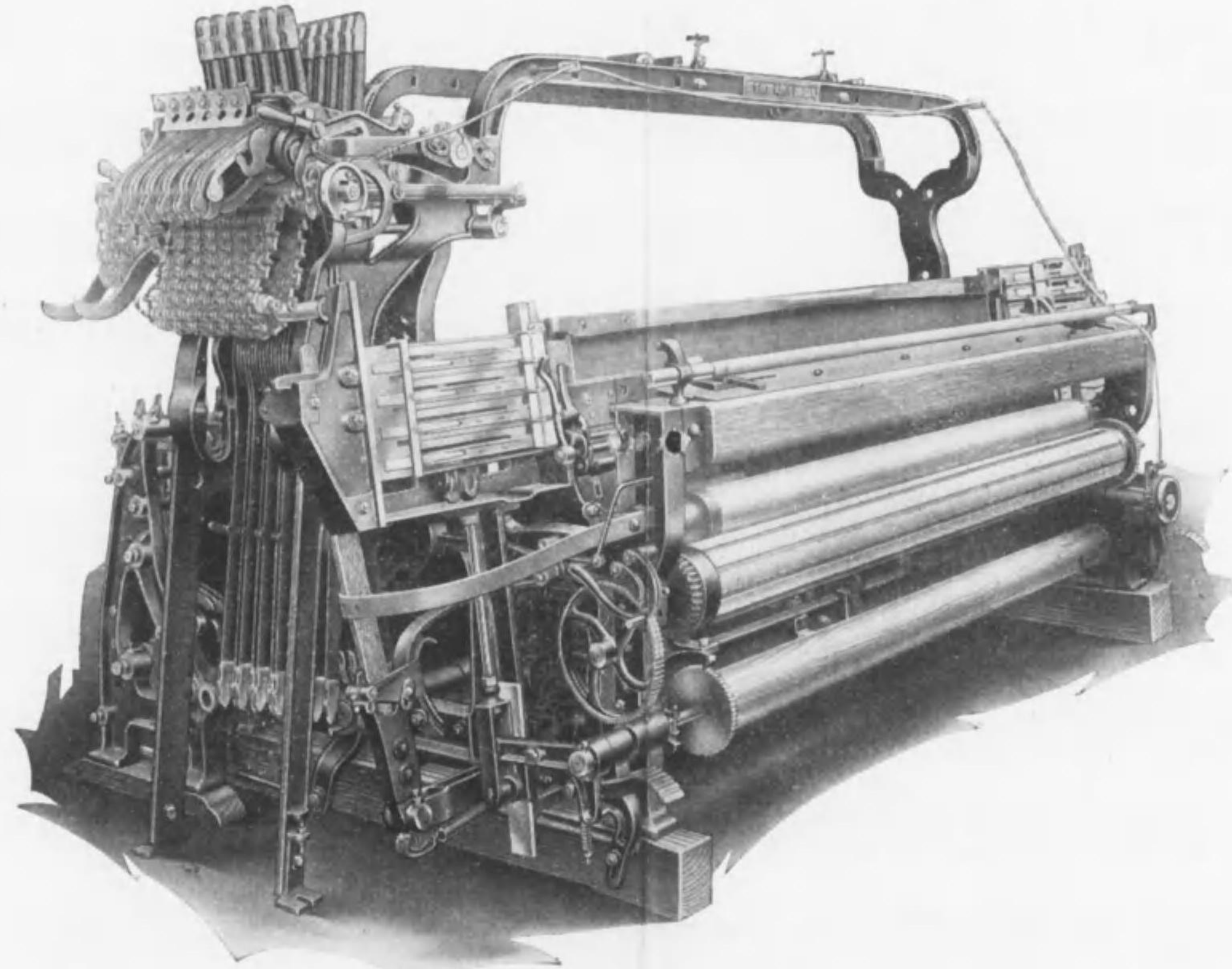
CE型92吋兩側四丁杼毛織機
