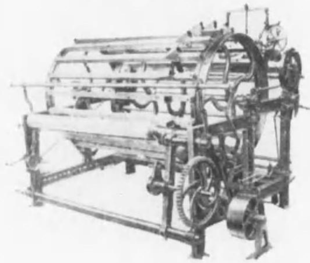
機經整分部
