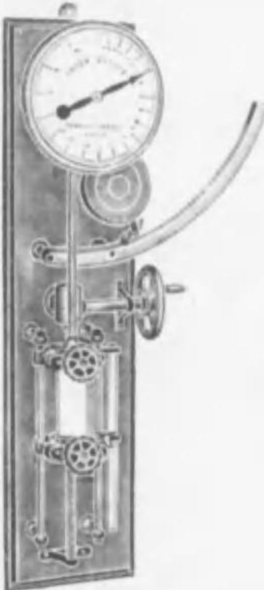
豎型クロス テスター
