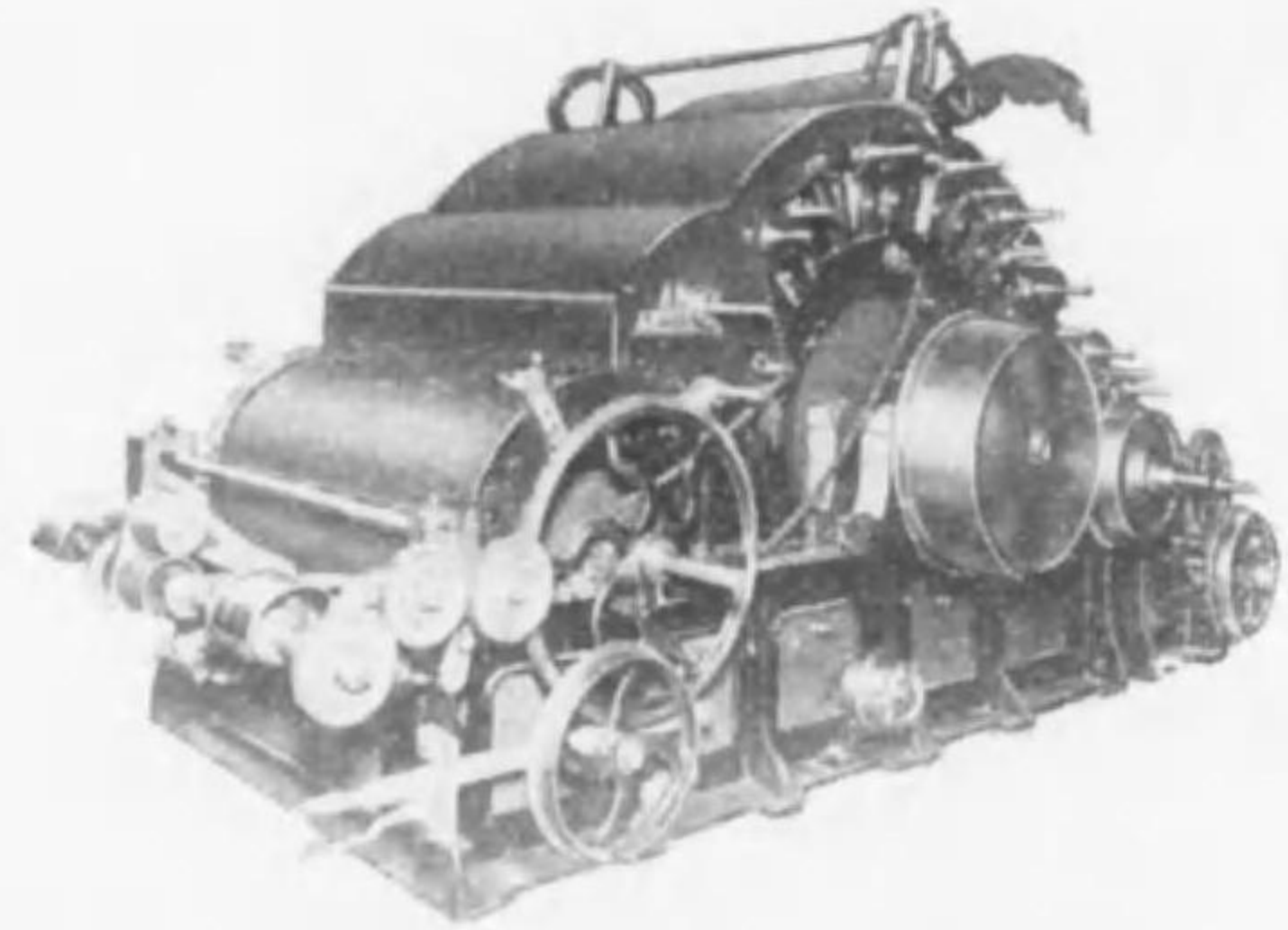
梳毛機
