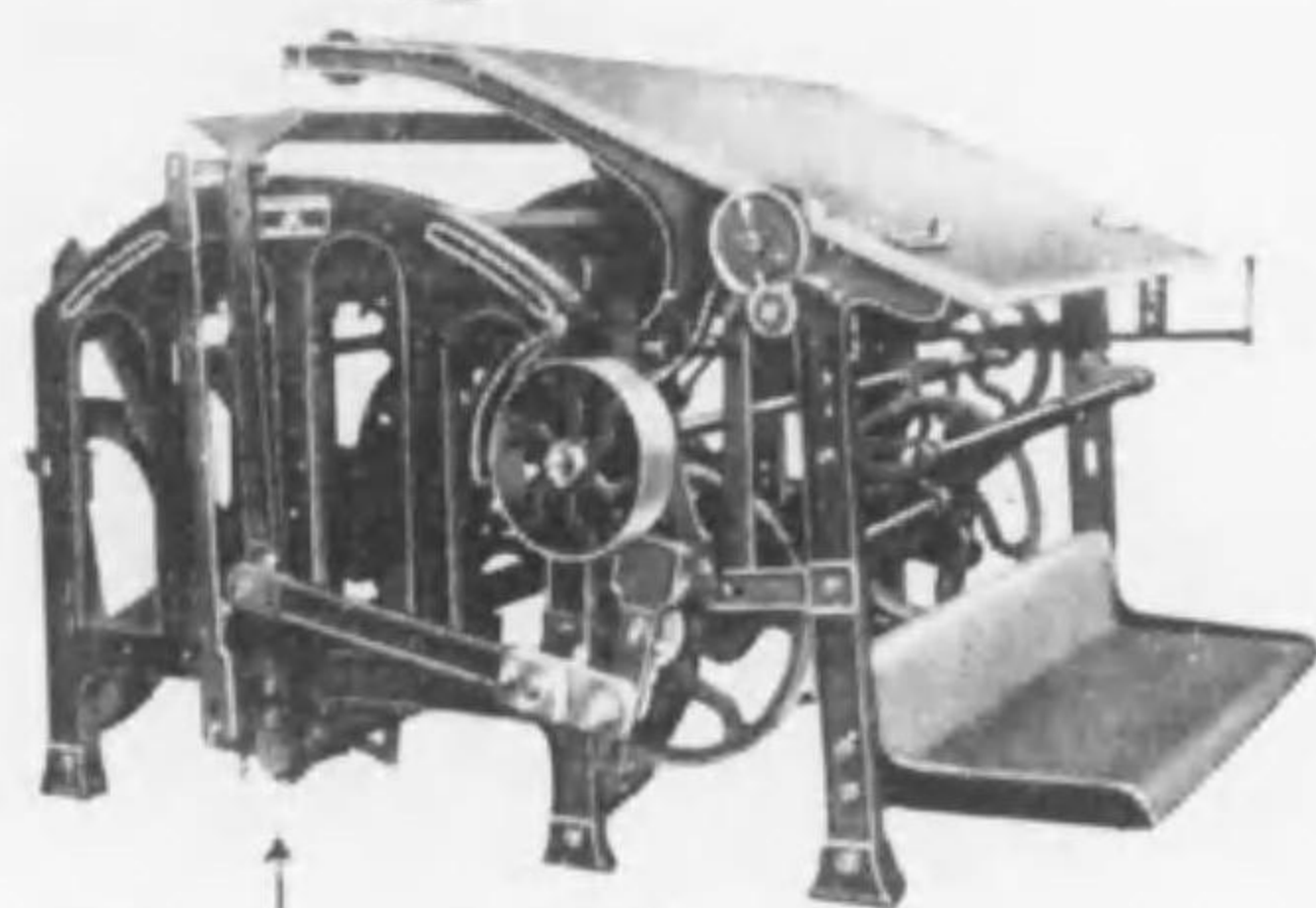
ヤルー疊機各式
