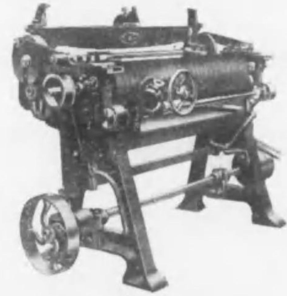
トツブグライディングマシン
