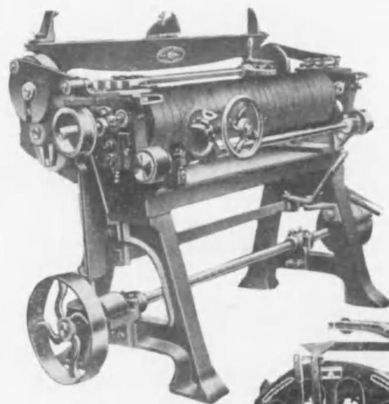
紡績用各種 附屬機械製作 トツブグラインチンク マシン
