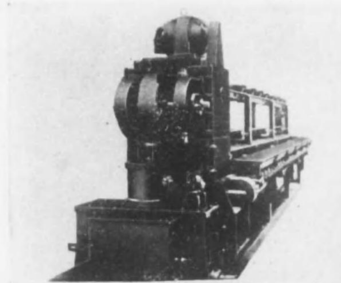
ファイバー切斷装置付き ステーブル ファイバー紡出機械
