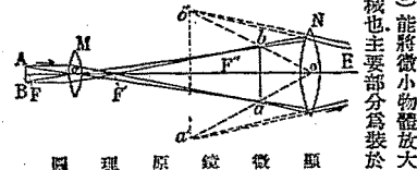
顯微鏡原理圖
