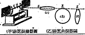
(甲)赫芝共振器圖 (乙)赫芝共振器圖
