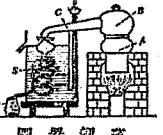
圖 器 餾 蒸
