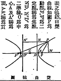
雙曲線圖
