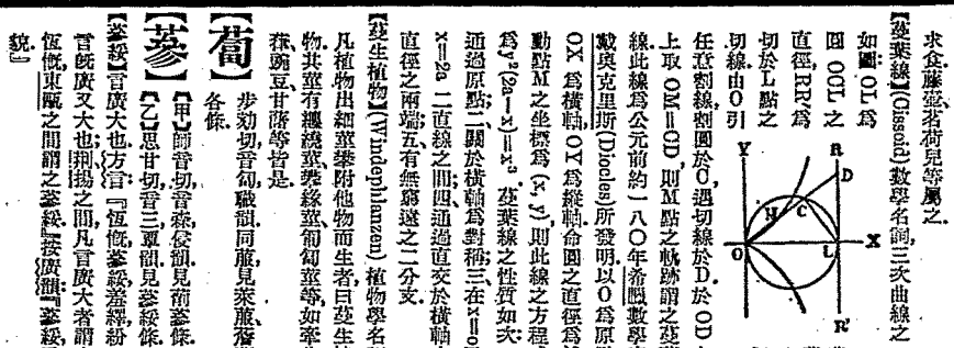
圖 斐葉線
