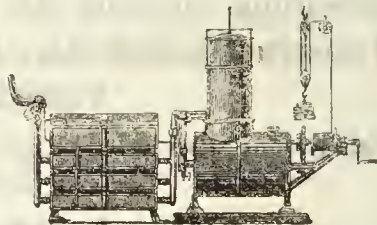
Luftgasapparat „Eureka.“
