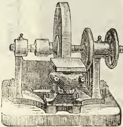
Einfache Schleifmaschine auf der Werkbank anzuschrauben, die Stahlwelle in Spitzen laufend.
