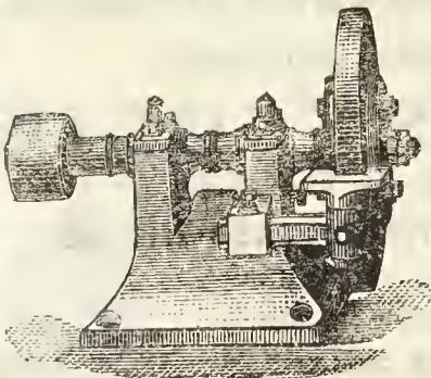
Einfache Schleifmaschine auf der Werkbank anzuschrauben.
