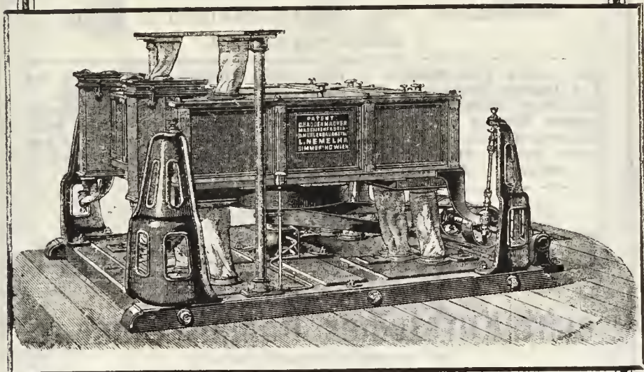
Quadratischer Plansichter.
