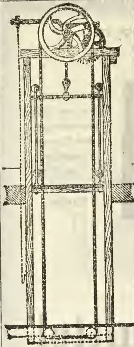
Lasten-Aufzug für Seilantrieb.
