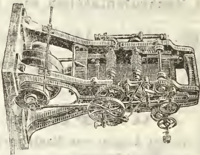
Sägegatter.
