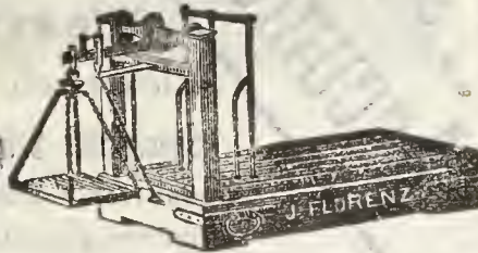
Decimalwaage mit doppelten Zugstangen (System Florenz).
